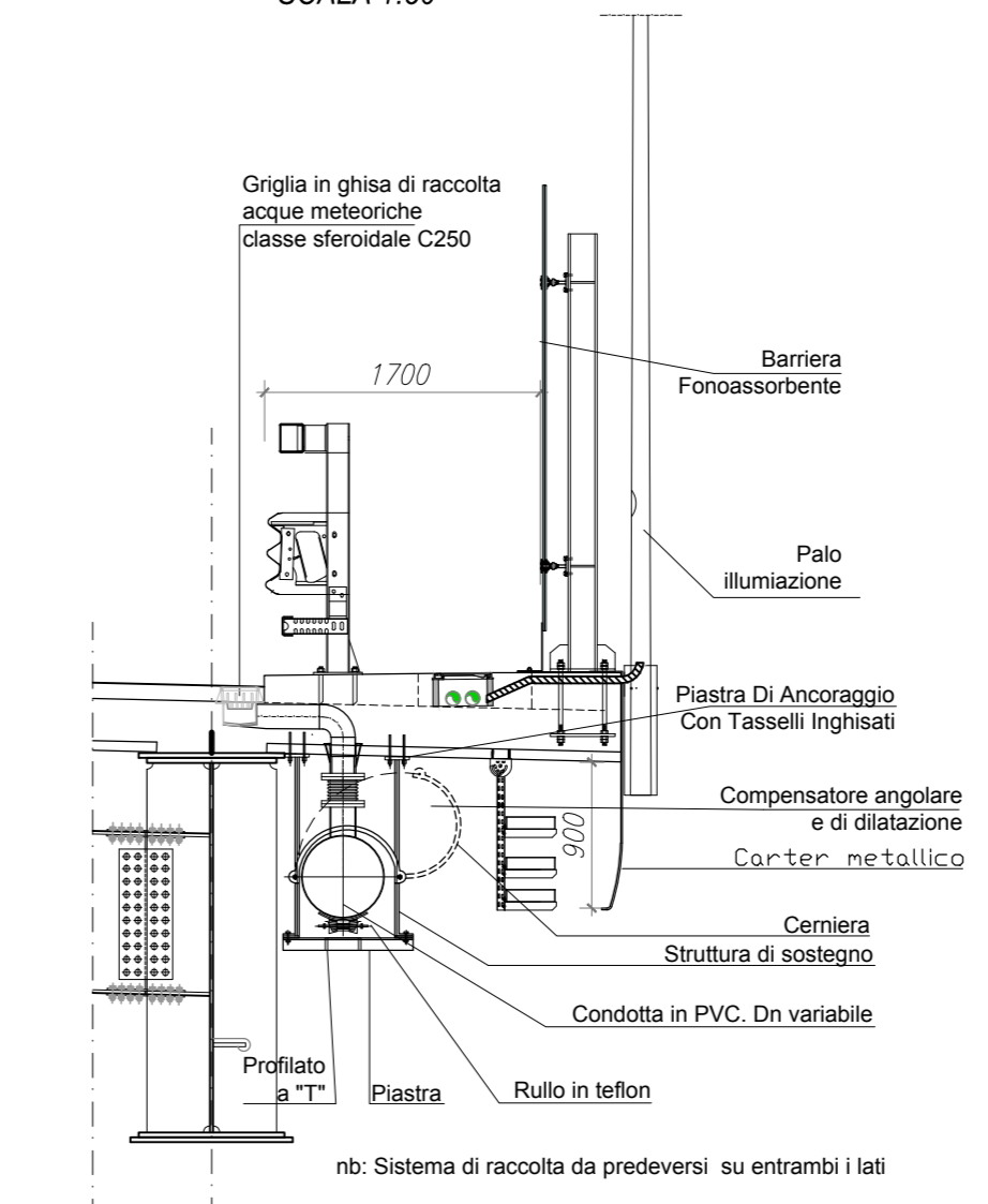
PARTICOLARE MARCIPIEDE SEZIONE SCALA 1:50
