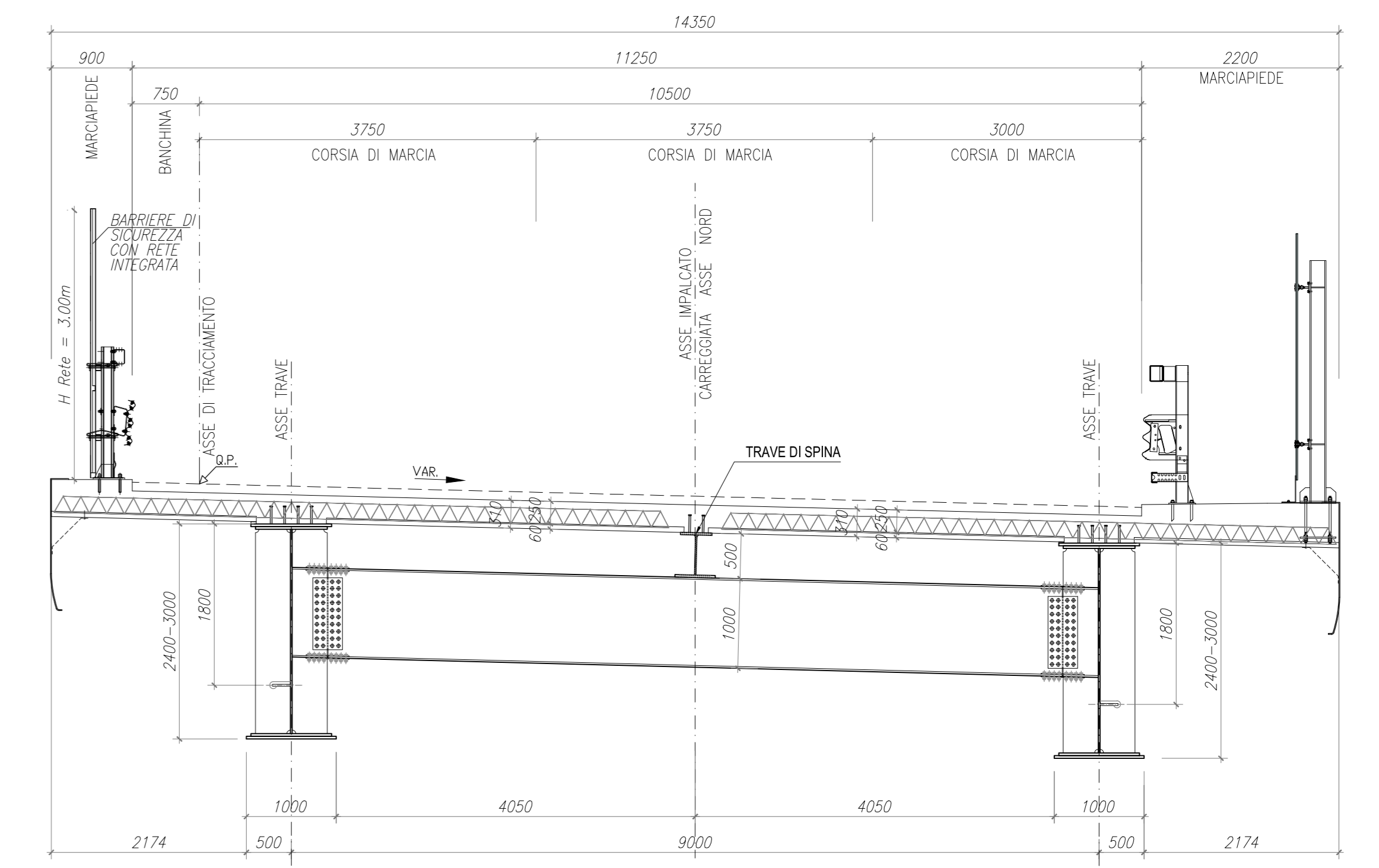
VIADOTTO SETTECA' TRAVERSO TIPO SCALA 1:50
