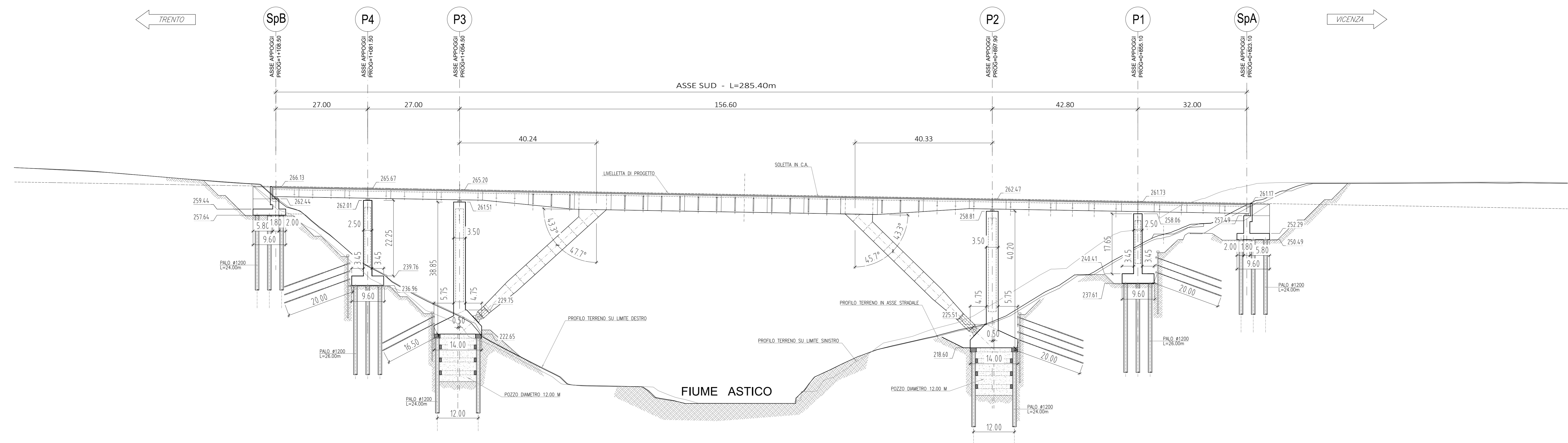
SEZIONE LONGITUDINALE CARREGGIATA SUD VIADOTTO PIOVENE SCALA 1:500
