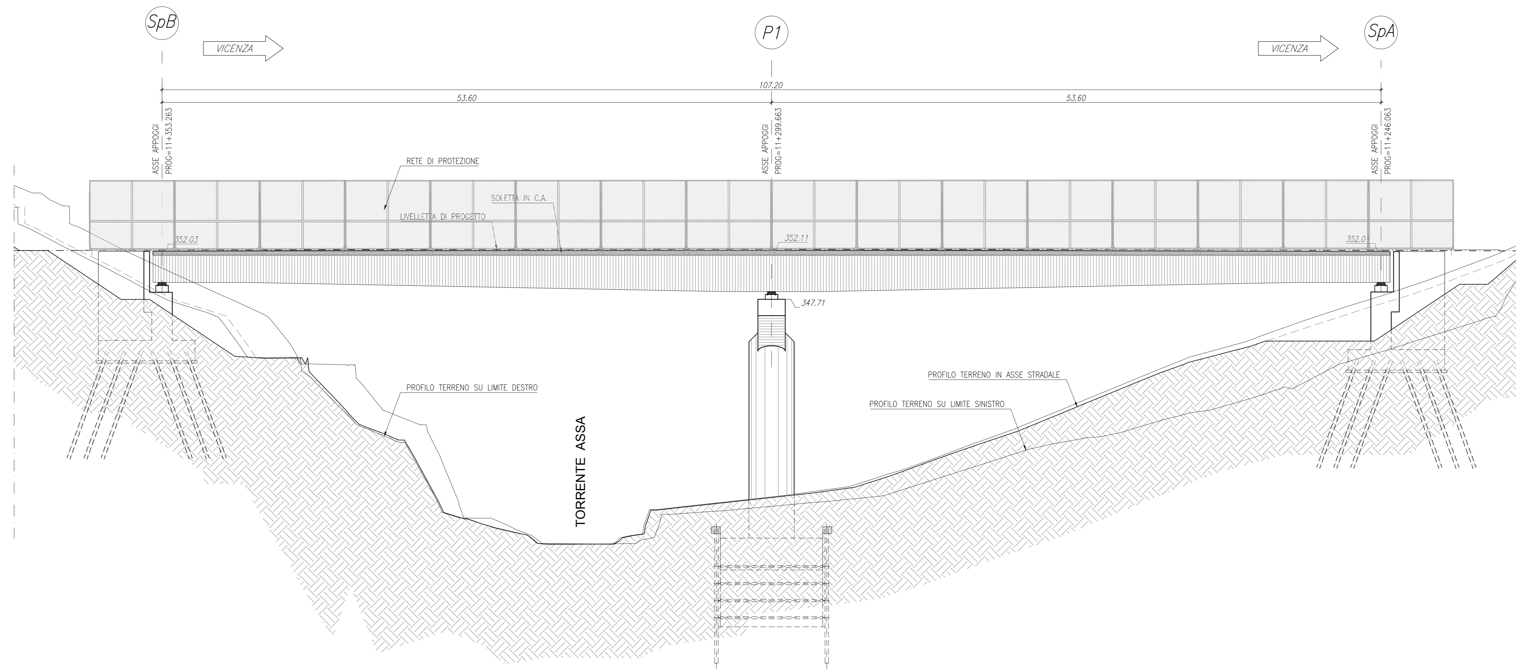
PROSPETTO LONGITUDINALE CARREGGIATA SUD SCALA 1:200
