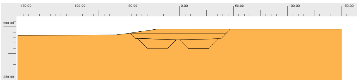
Sezione del modello Plaxis, profilo naturale del terreno
