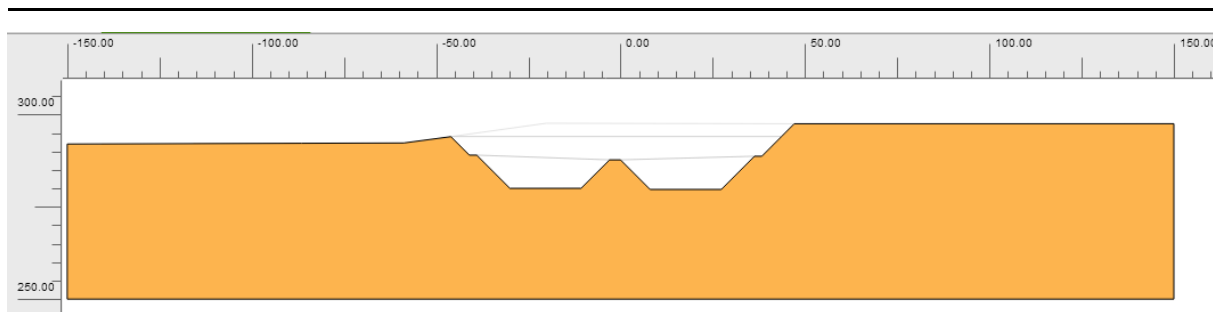
Sezione del modello Plaxis, profilo con scavo
