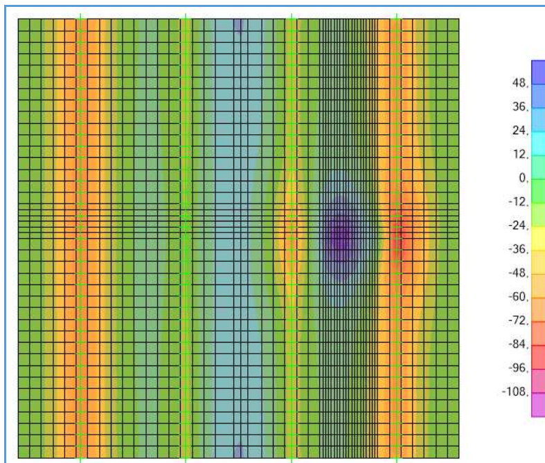
Schema di carico 2 – M_{11,MIN} - Involuppo – Mezzeria soletta
