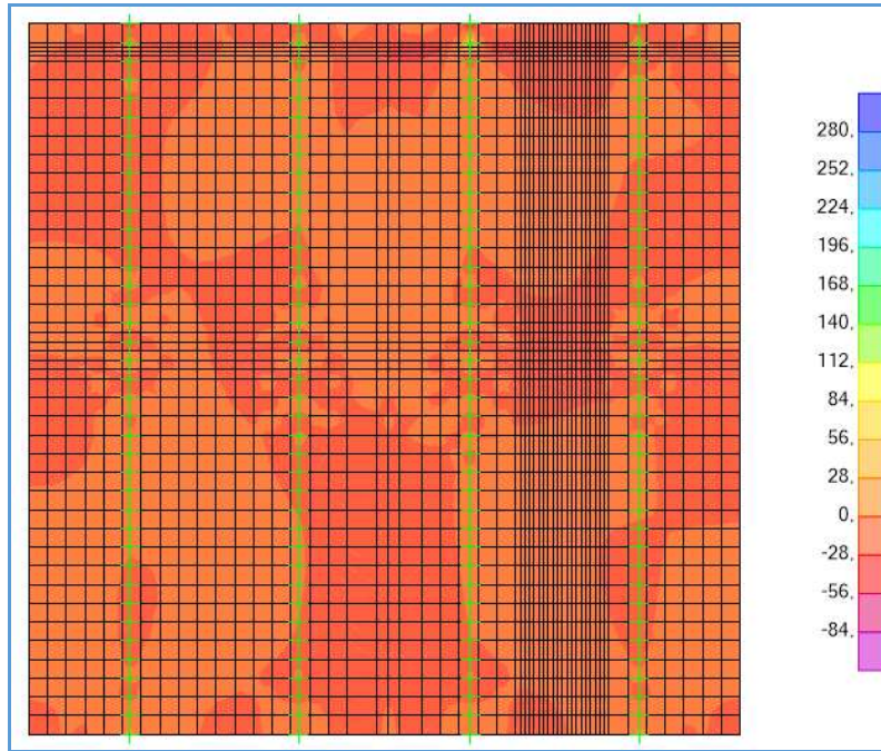
Schema di carico 2 – V_{23,MIN} - Involuppo – Bordo soletta
