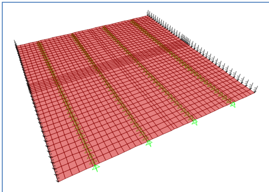
Carichi concentrati delle reti di protezione laterali applicati sui nodi
