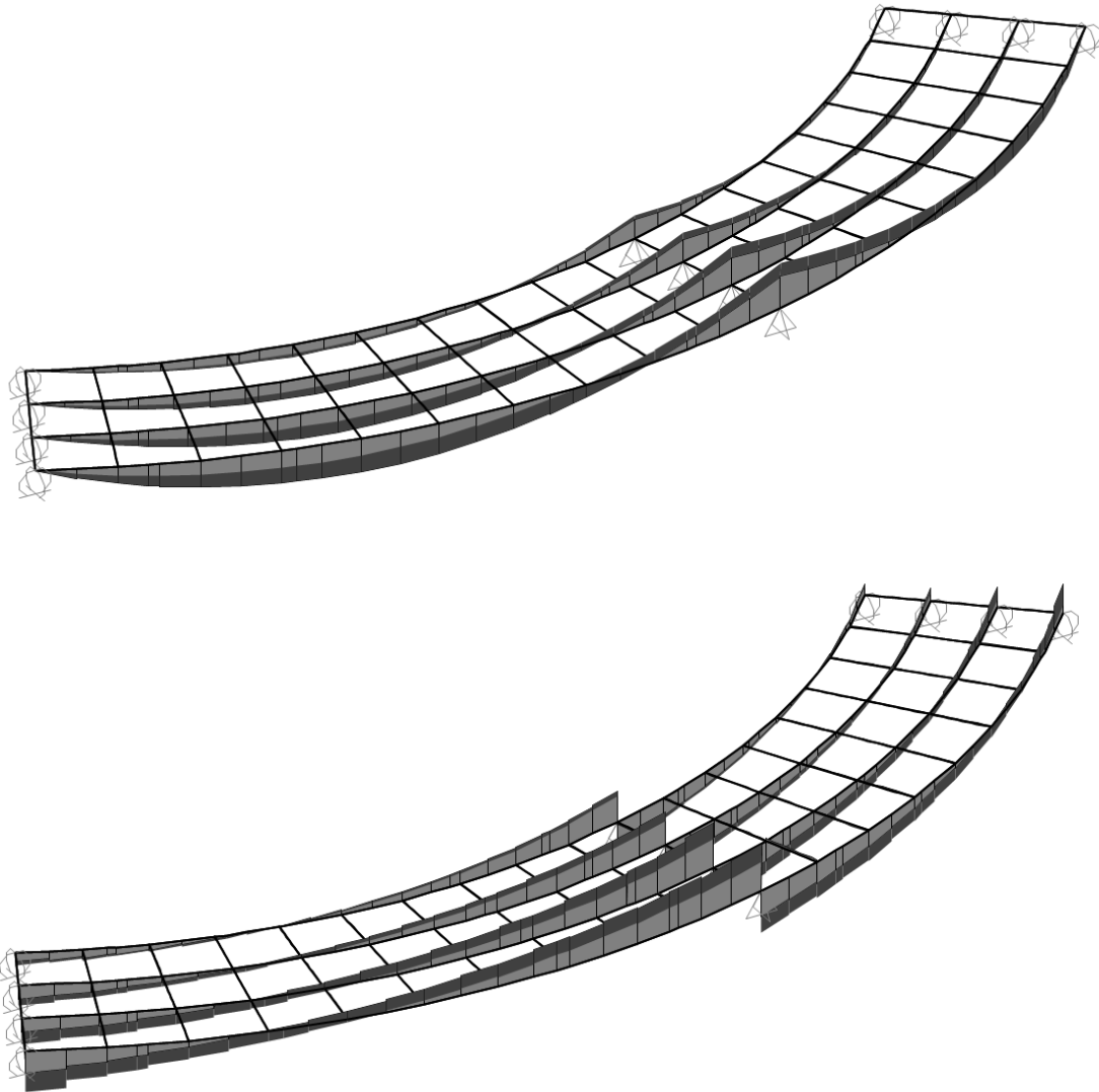
Diagramma del momento flettente e taglio
