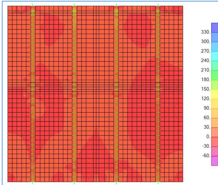
Schema di carico 1 – V_{23,MAX} - Involuppo – Bordo soletta
