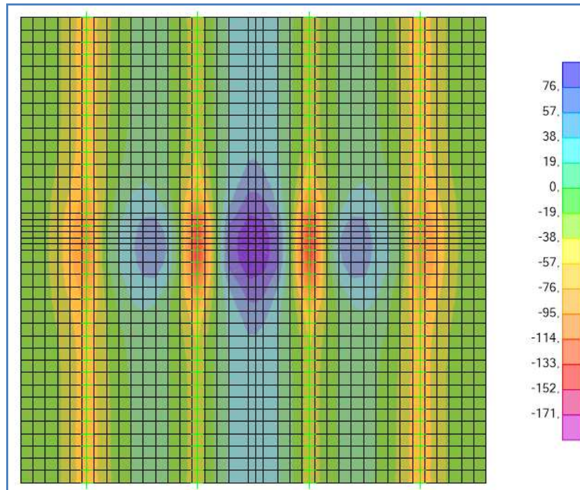
Schema di carico 1 – M_{11,MIN} - Inviluppo – Mezzeria soletta
