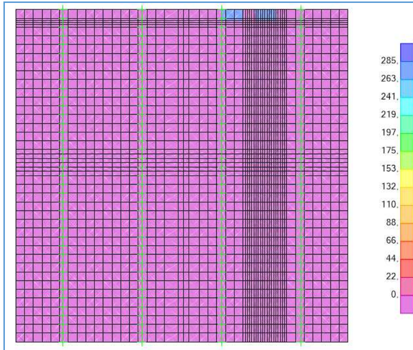
Schema di carico 2 – Disposizione C del carico – Bordo soletta
