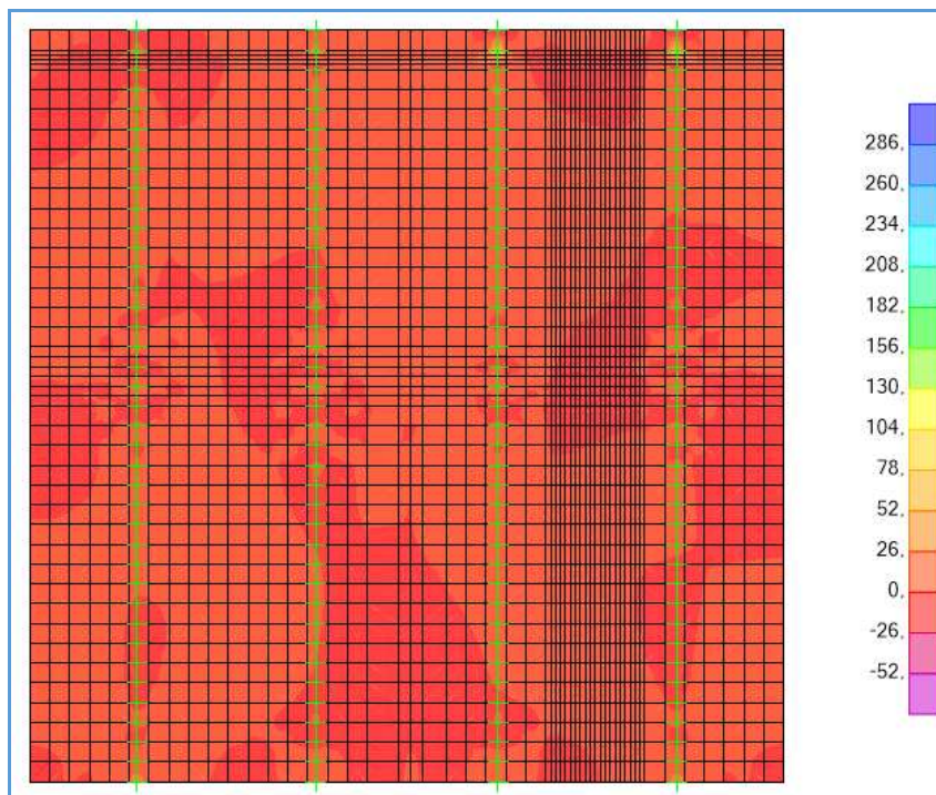
Schema di carico 2 – V_{23.MAX} - Involuppo – Bordo soletta
