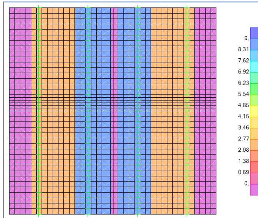
Schema di carico 1 – Disposizione E dei carichi distribuiti di corsia
