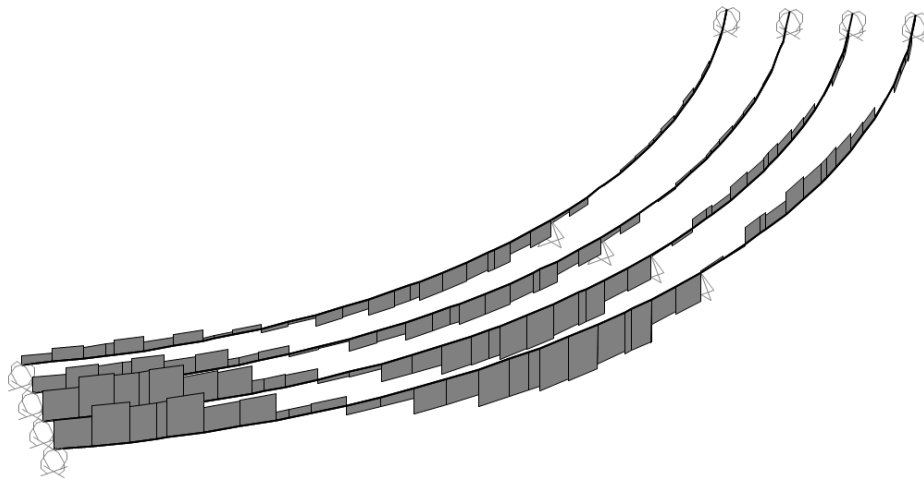
Diagramma Momenti Torcenti_g2
