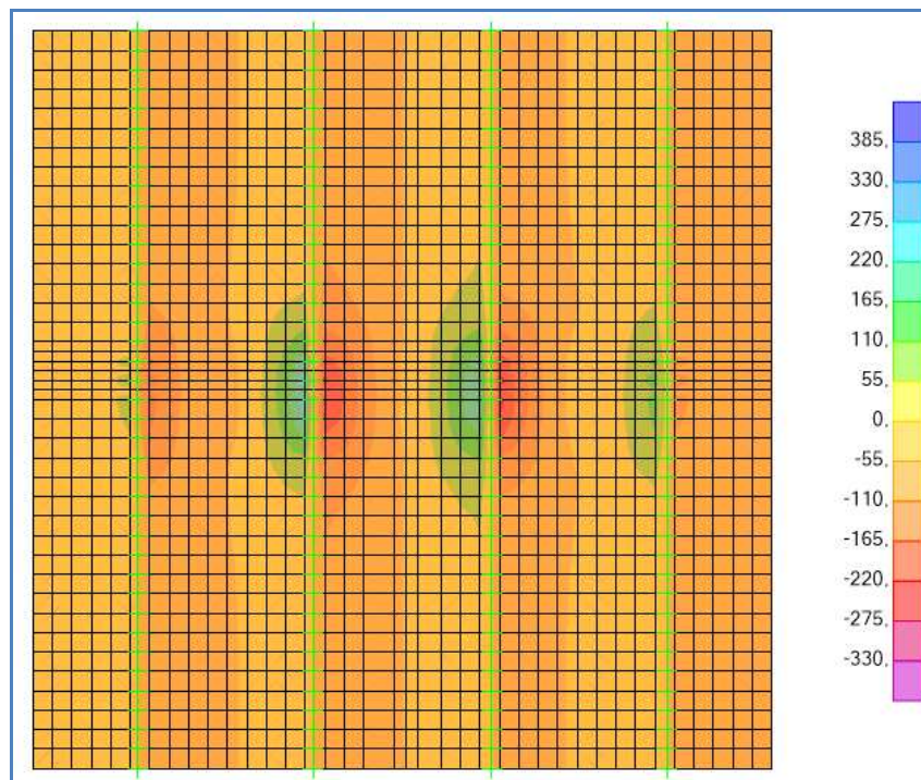
Schema di carico 1 – V_{13,MAX} - Inviluppo – Mezzeria soletta
