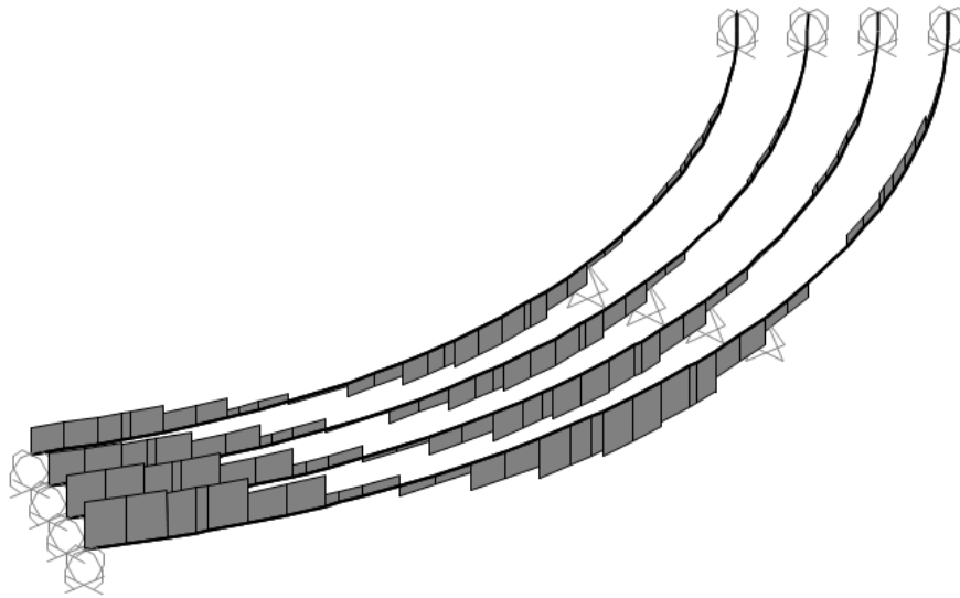
Diagramma Momenti Torcenti_G1
