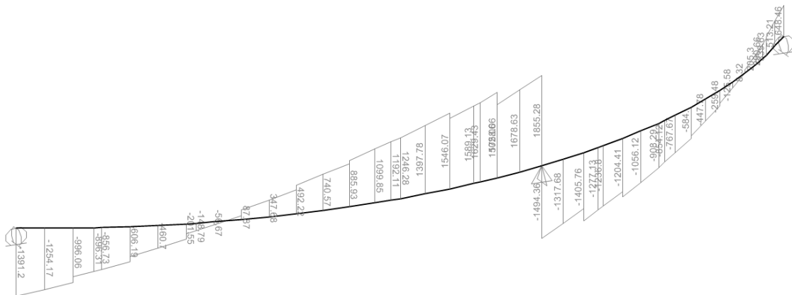
Diagramma del Momento – fase 1 (caratteristica) – modello di calcolo
