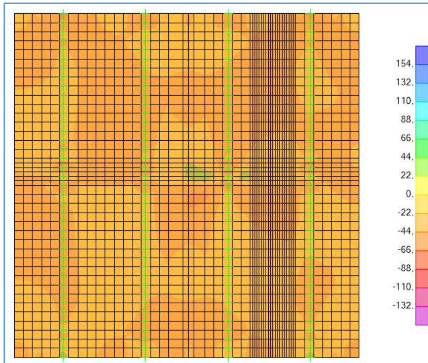
Schema di carico 2 – V_{23,MAX} - Inviluppo – Mezzeria soletta
