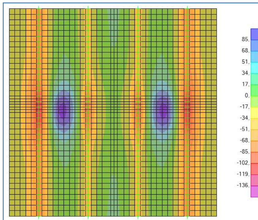
Schema di carico 1 – M 11,MAX – Inviluppo – Mezzeria soletta
