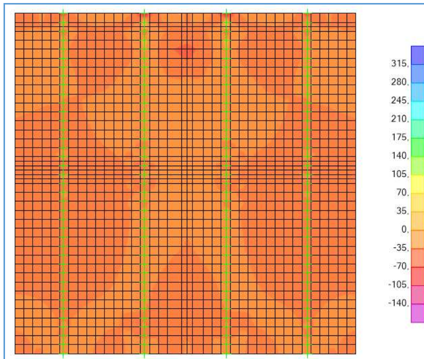
Schema di carico 1 – V_{23,MIN} - Involuppo – Bordo soletta
