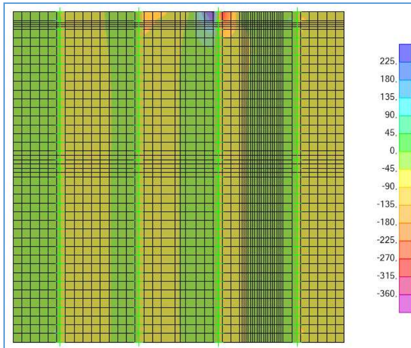
Schema di carico 2 – V_{13.MIN} - Involuppo – Bordo soletta
