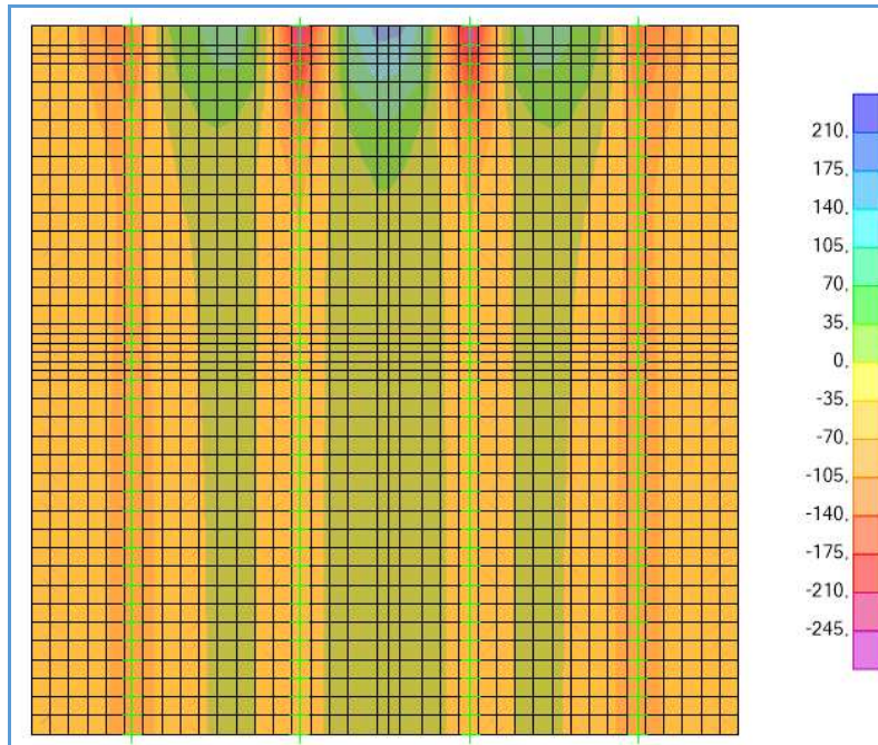
Schema di carico 1 – M_{11,MIN} - Involuppo – Bordo soletta
