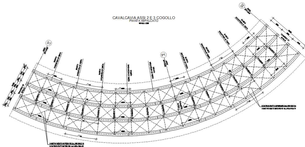
Immagine 2: Pianta impalcato
