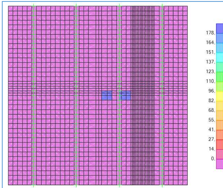
Schema di carico 2 – Disposizione C del carico – Mezzeria soletta
