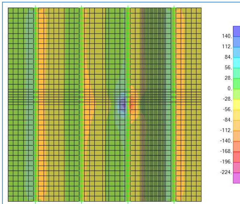
Schema di carico 2 – V_{13,MIN} - Inviluppo – Mezzeria soletta
