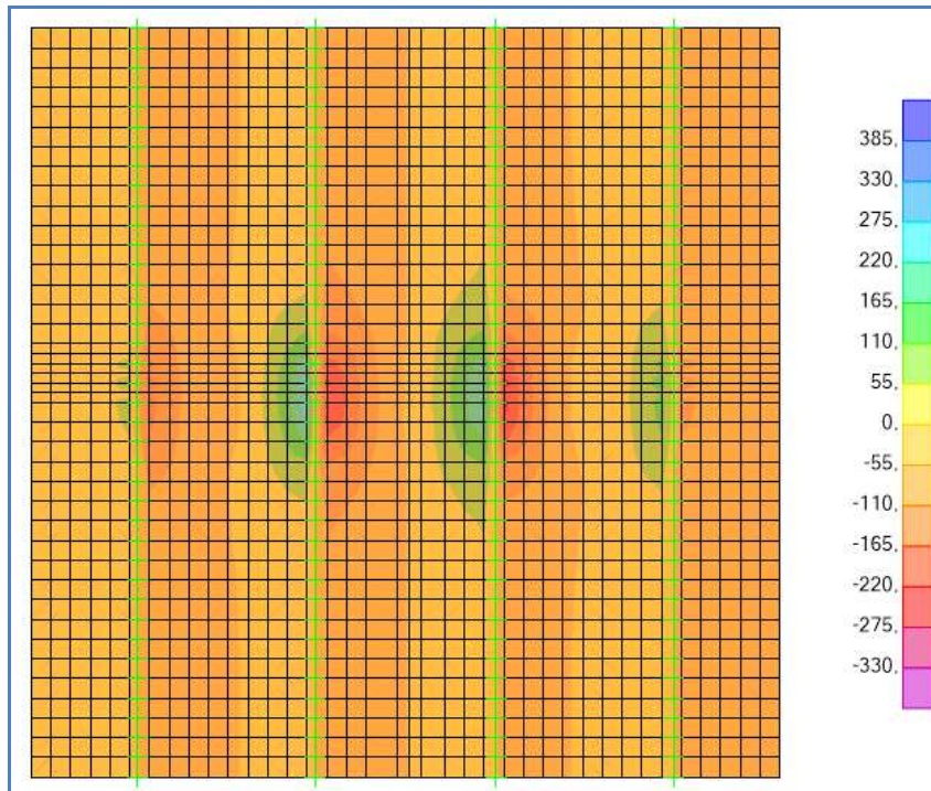
Schema di carico 1 – V_{13.MIN} - Inviluppo – Mezzeria soletta
