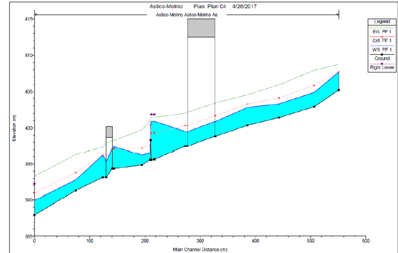
Figura 13 Profilo longitudinale del Fiume Astico in corrispondenza del viadotto Molino – Portata duecentennale – Post Operam
