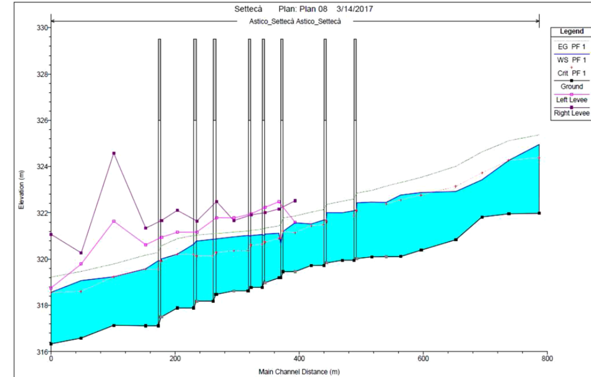
Figura 10 Profilo longitudinale del Fiume Astico in corrispondenza del viadotto Settecà – Portata duecentennale – Post Operam
