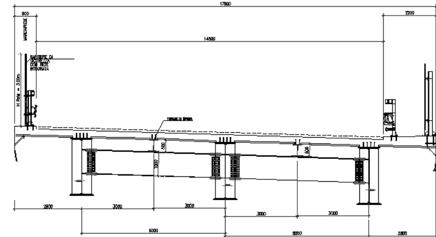
Figura 8- Sezione trasversale Viadotto Settecà
