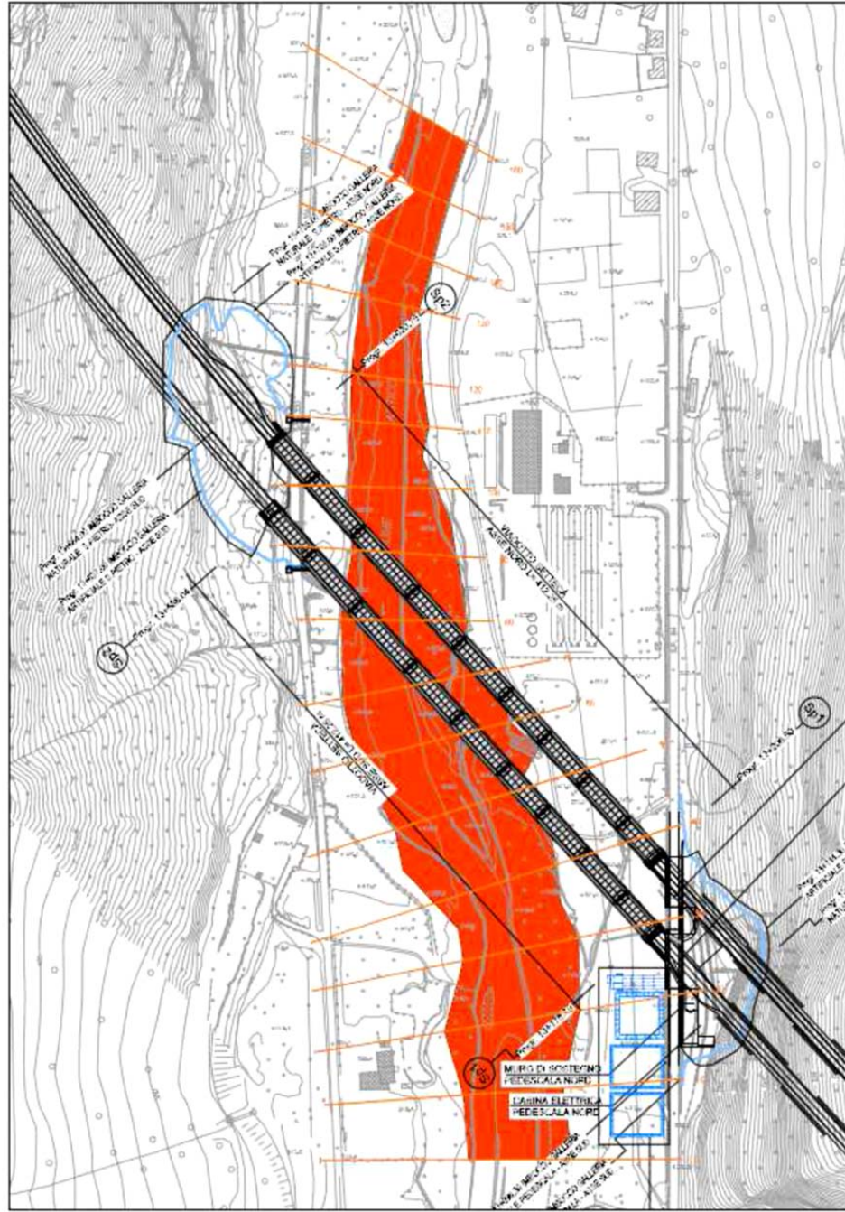
Figura 9 Aree di esondazione del Fiume Astico in corrispondenza del viadotto Settecà – Portata duecentennale – Post Operam
