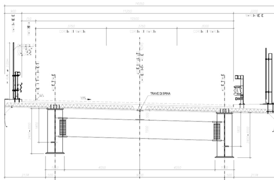
Figura 11- Sezione trasversale
