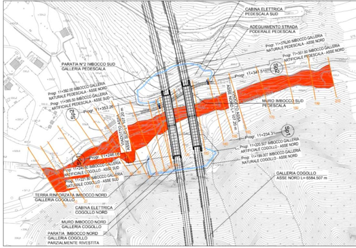
Figura 6 Aree di esondazione del Torrente Assa in corrispondenza del viadotto Assa – Portata duecentennale – Post Operam
