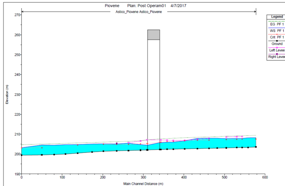
Figura 4 Profilo longitudinale del Fiume Astico in corrispondenza del viadotto Piovene – Portata duecentennale – Post Operam
