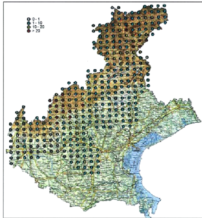
Figura 29 Frazioni di abitazioni (%) con livelli eccedenti 200 Bq/m 3 dopo smoothing e riempimento (dati normalizzati ad housing stock) sovrapposte alla carta geografica del Veneto (Fonte: ARPAV).
