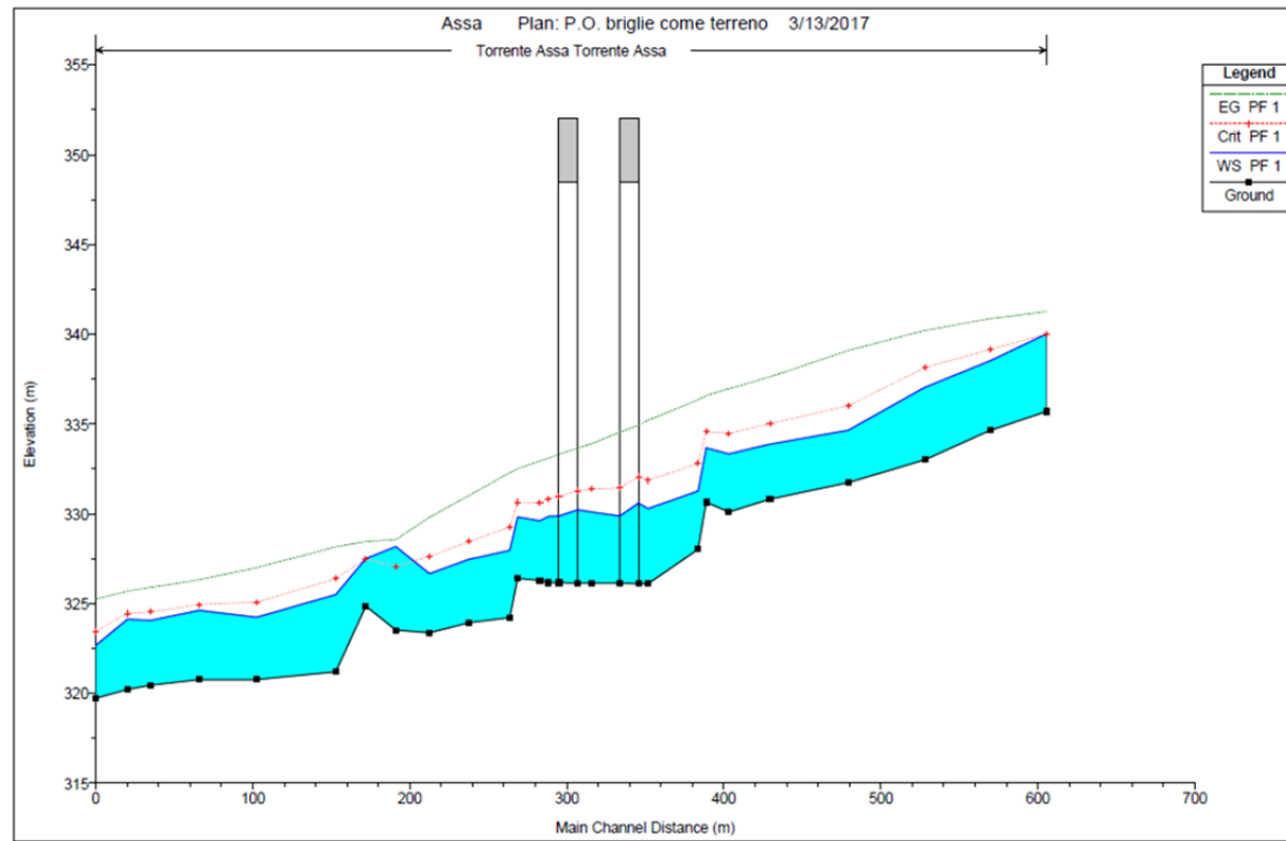
Figura 7 Profilo longitudinale del Torrente Assa in corrispondenza del viadotto Assa – Portata duecentennale – Post Operam
