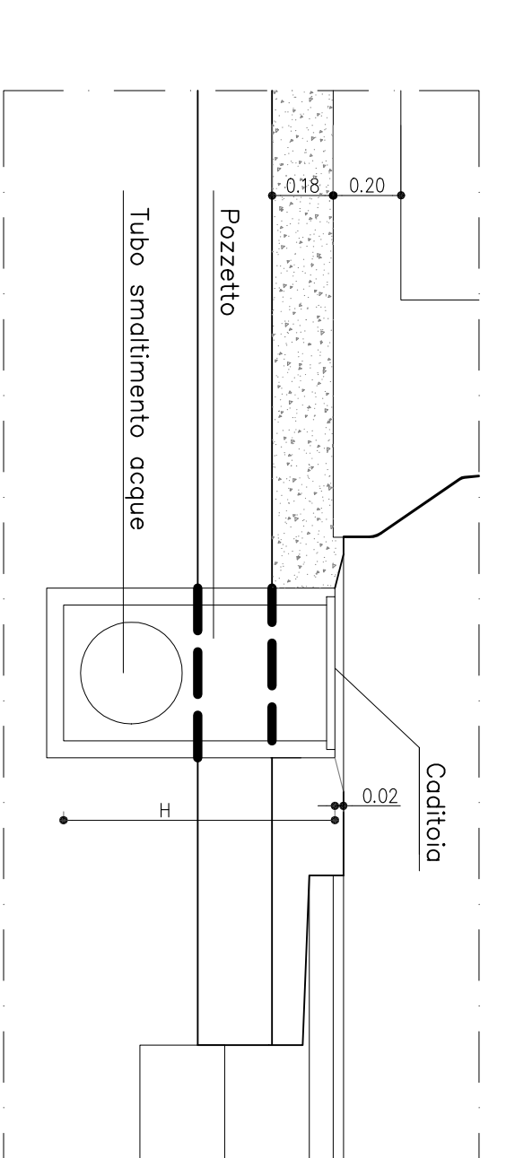
PARTICOLARE CADITOIA SEZIONE SCALA 1:20
