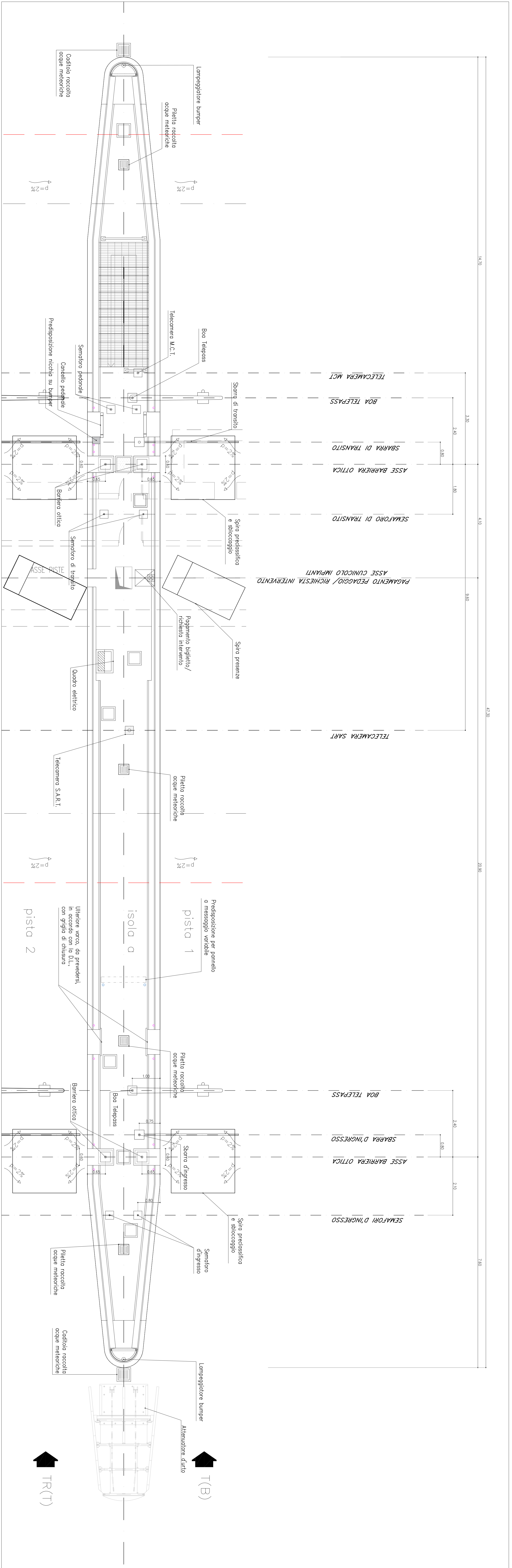
PARTICOLARE PISTA IN ENTRATA SCALA 1:50
