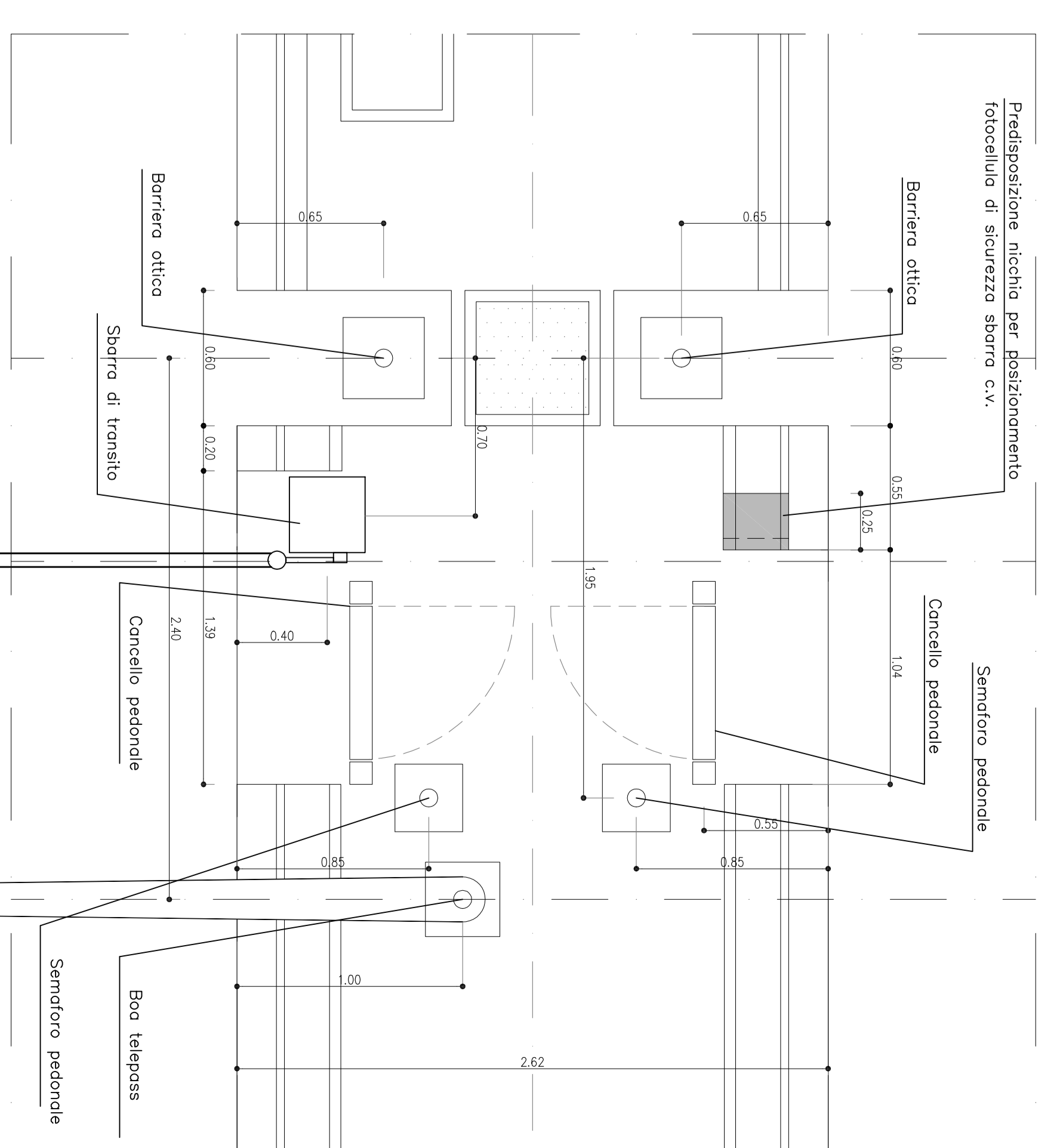
PARTICOLARE ATTRAVERSAMENTO PEDONALE SCALA 1:20
