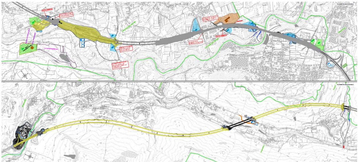
Figura 34 – Opere da iniziare a realizzare in Fase 2
