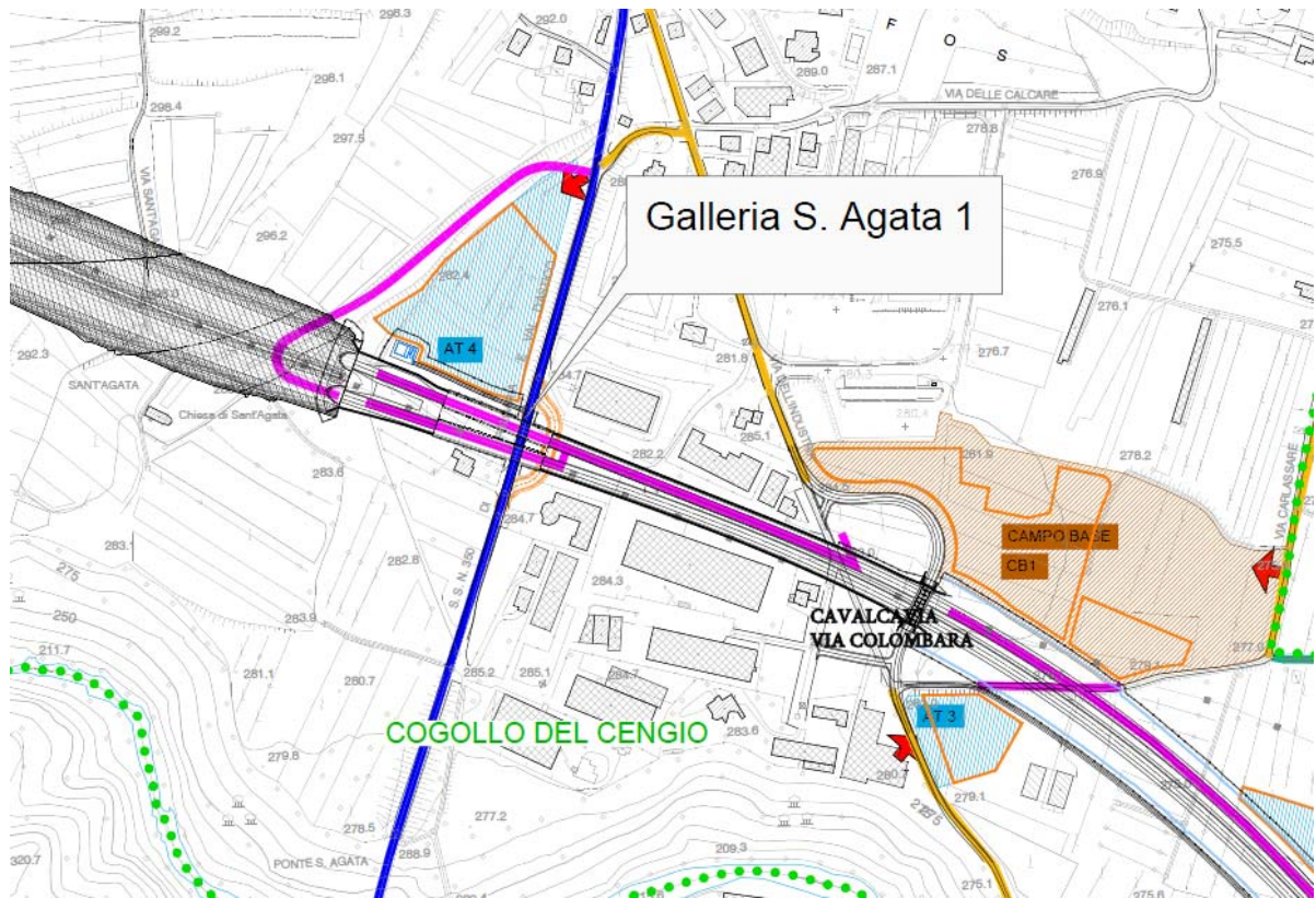
Figura 32 - Interferenze con S.Agata 1 e Cavalcavia Colombara
