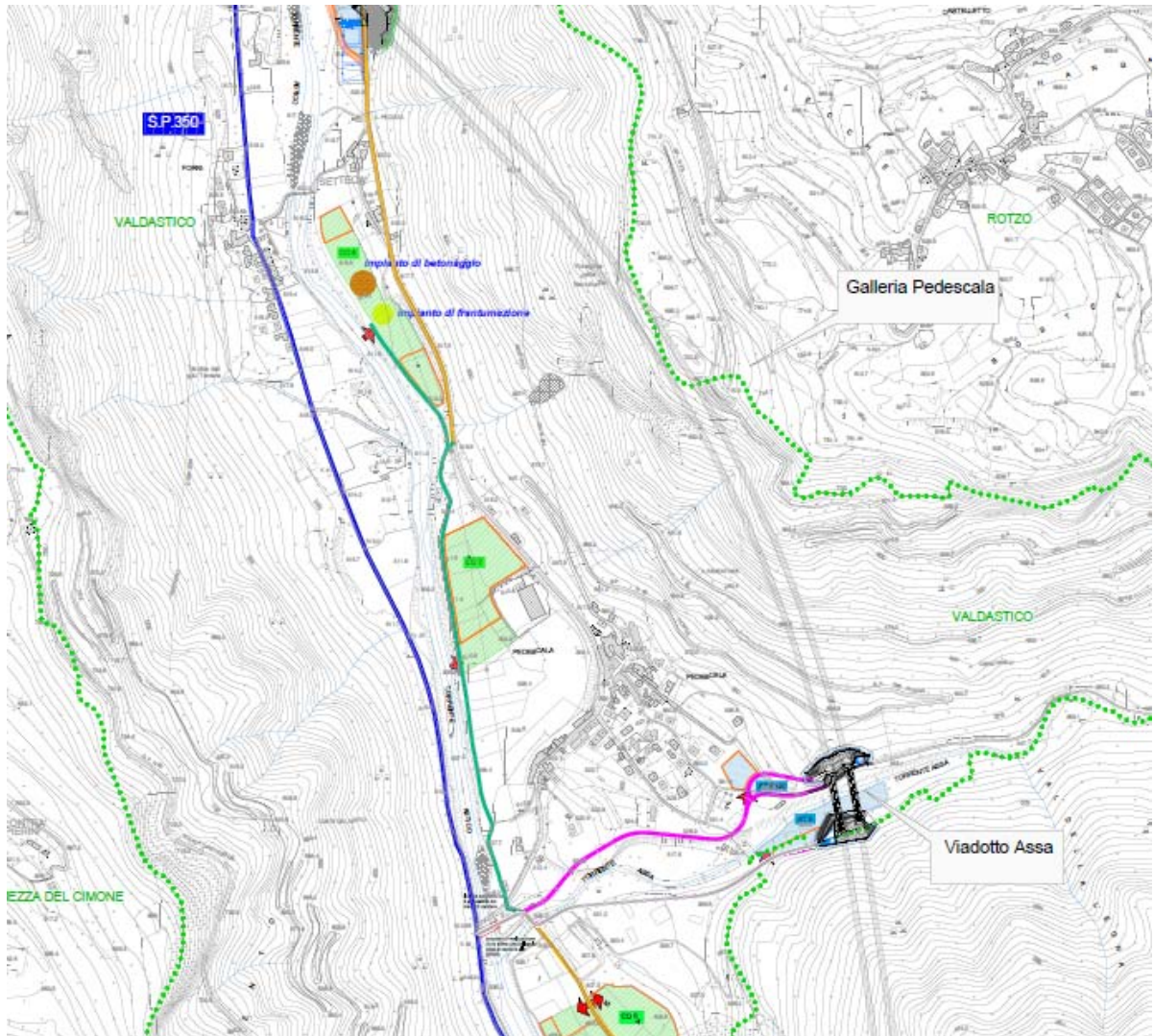
Figura 35 – Galleria Pedescala
