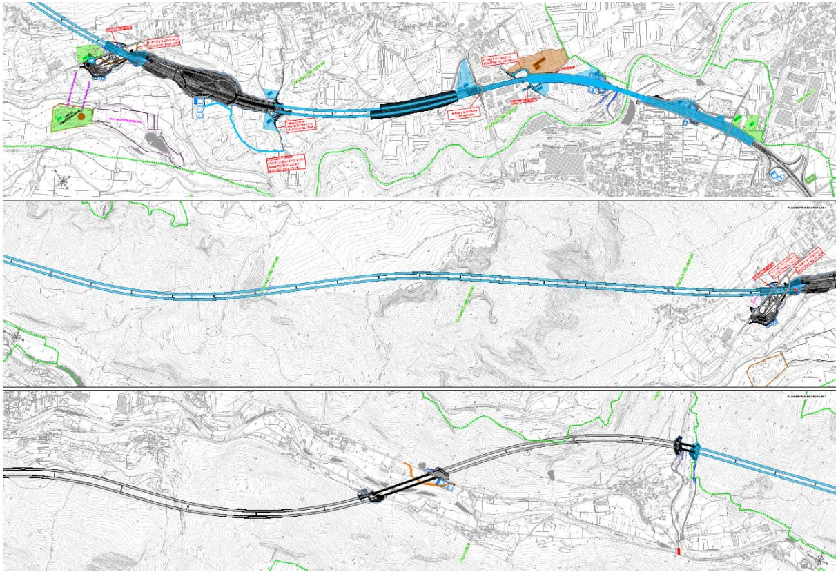
Figura 28 -- Opere da iniziare a realizzare in Fase 1
