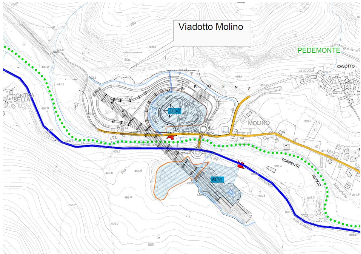
Figura 37 – Viadotto Molino e Svincolo di Valle dell'Astico
