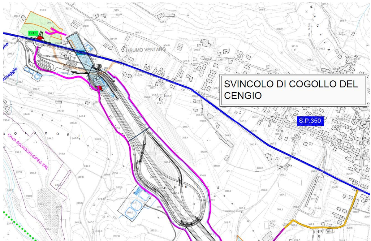
Figura 29 – Imbocco sud Galleria Cogollo e Vincolo di Cogollo del Cengio
