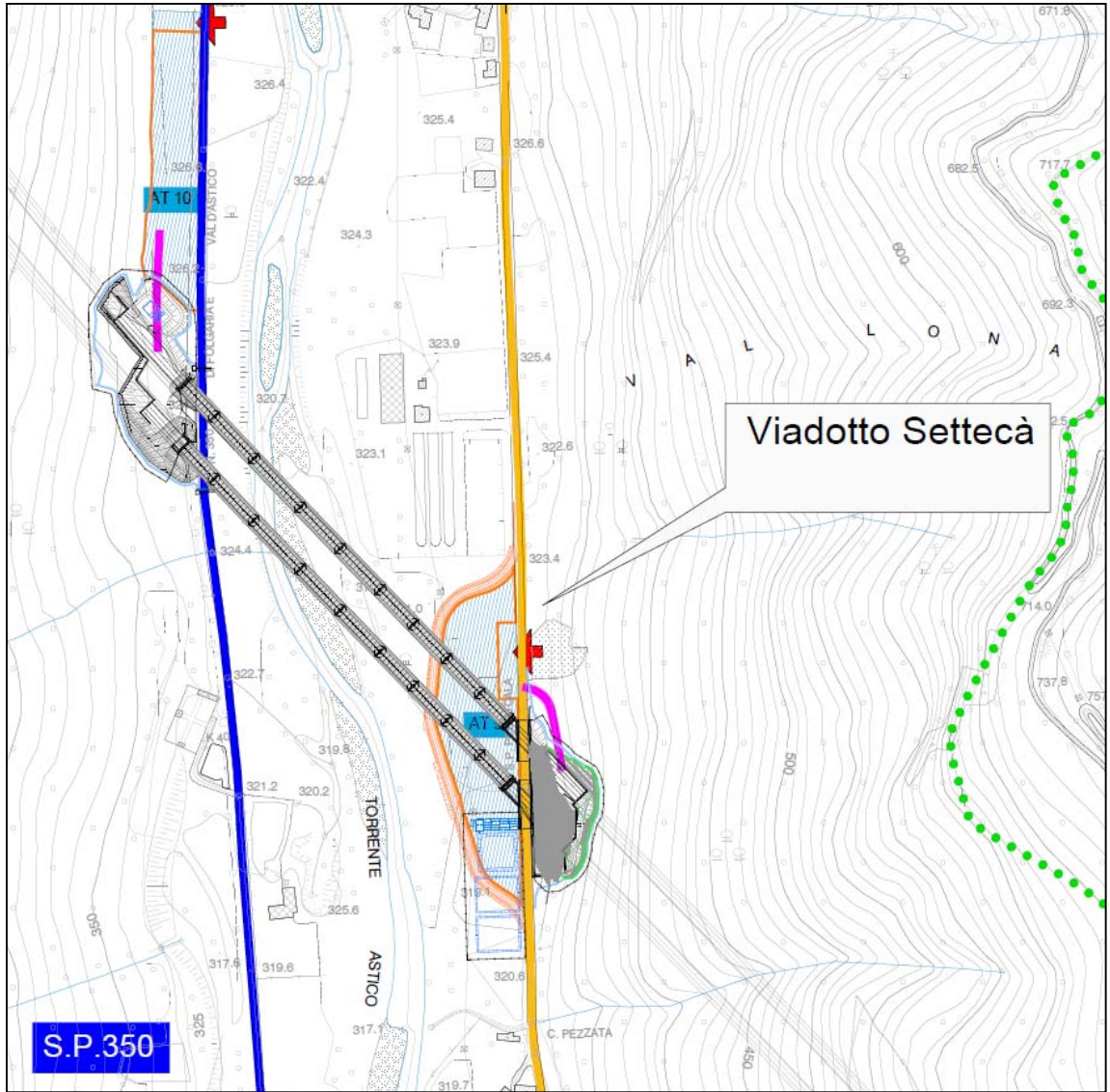
Figura 39 – Viadotto Settecà
