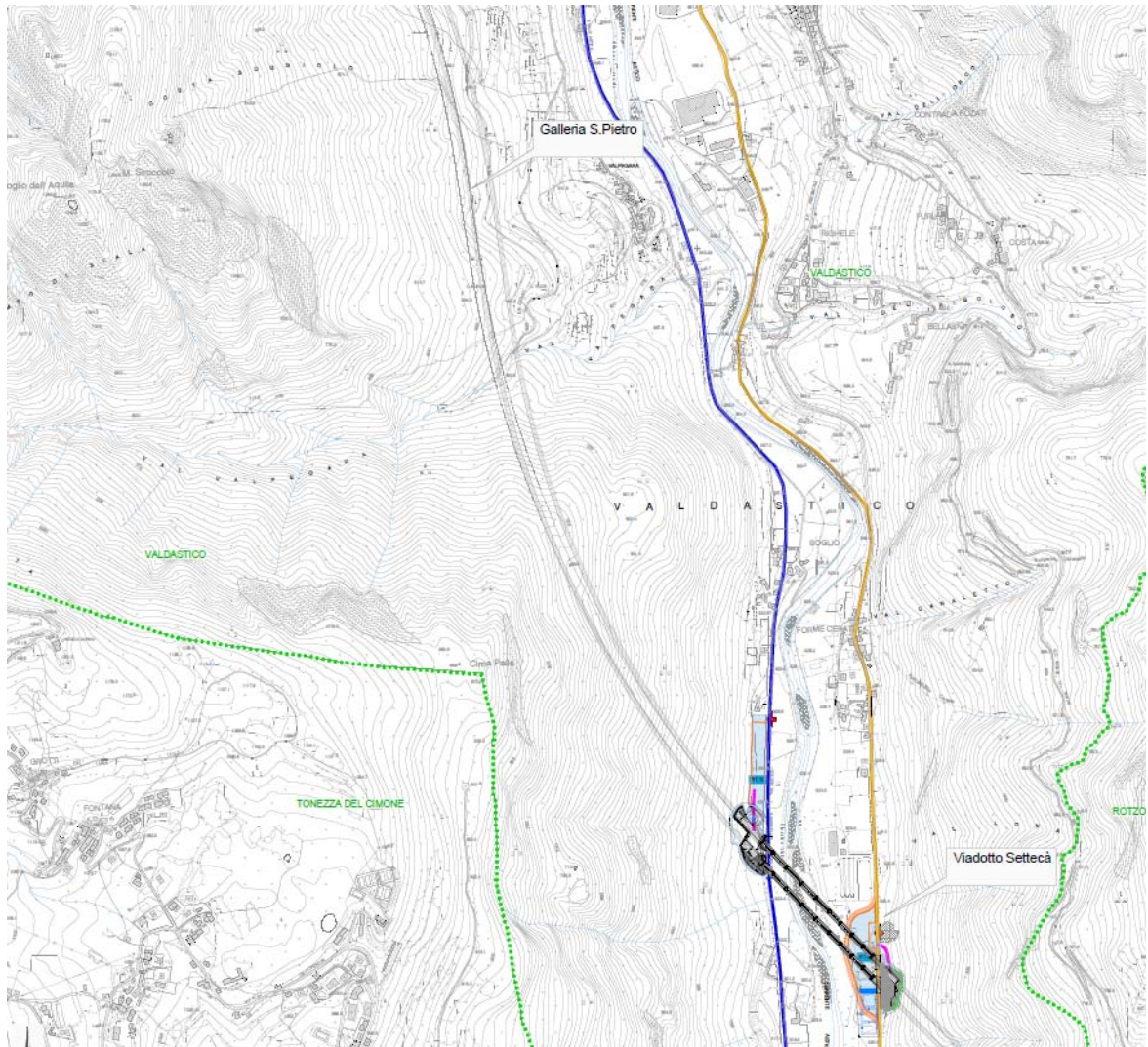
Figura 36– Galleria S.Pietro
