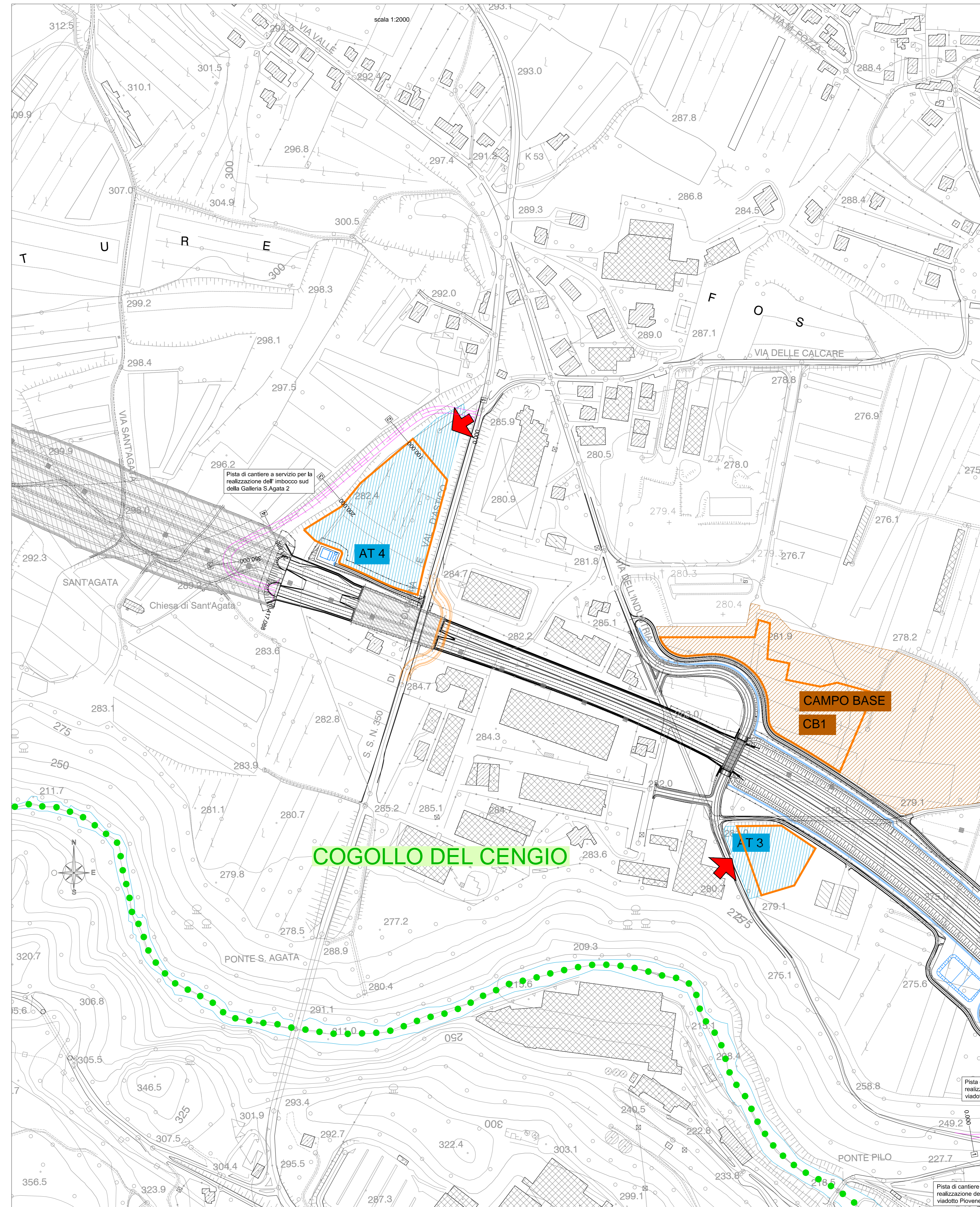
PLANIMETRIA DI PROGETTO IMBOCCO SUD GALLERIA S.AGATA 2- PISTE DI CANTIERE - TAV 2 scala 1:2000
