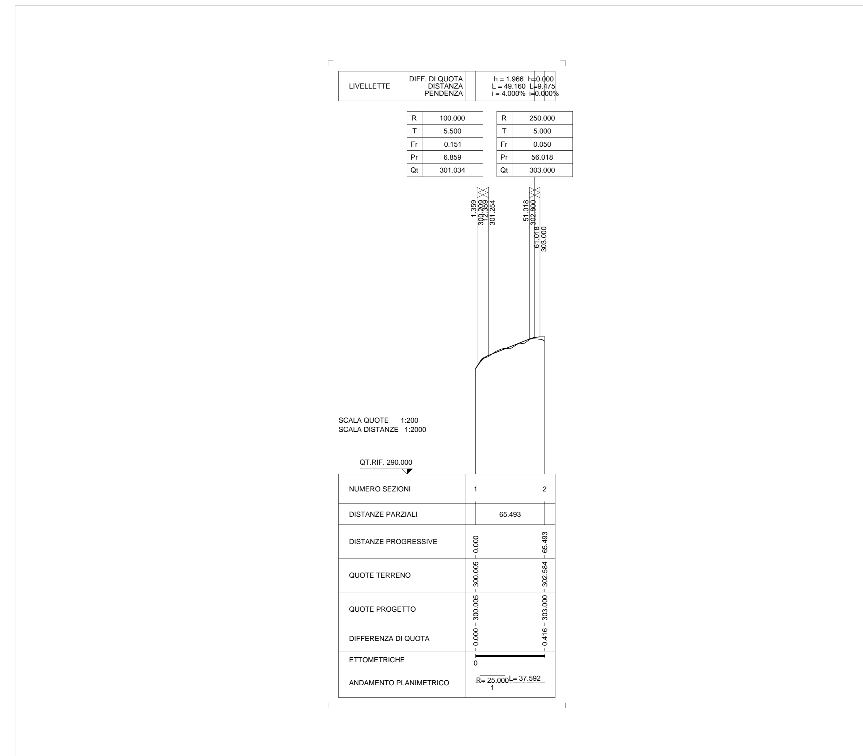
PROFILO LONGITUDINALE PISTA DI CANTIERE A SERVIZIO PER LA REALIZZAZIONE DEI MICROPALI DELL'IMBOCCO SUD GALLERIA COGOLLO scala 1:2000/200
