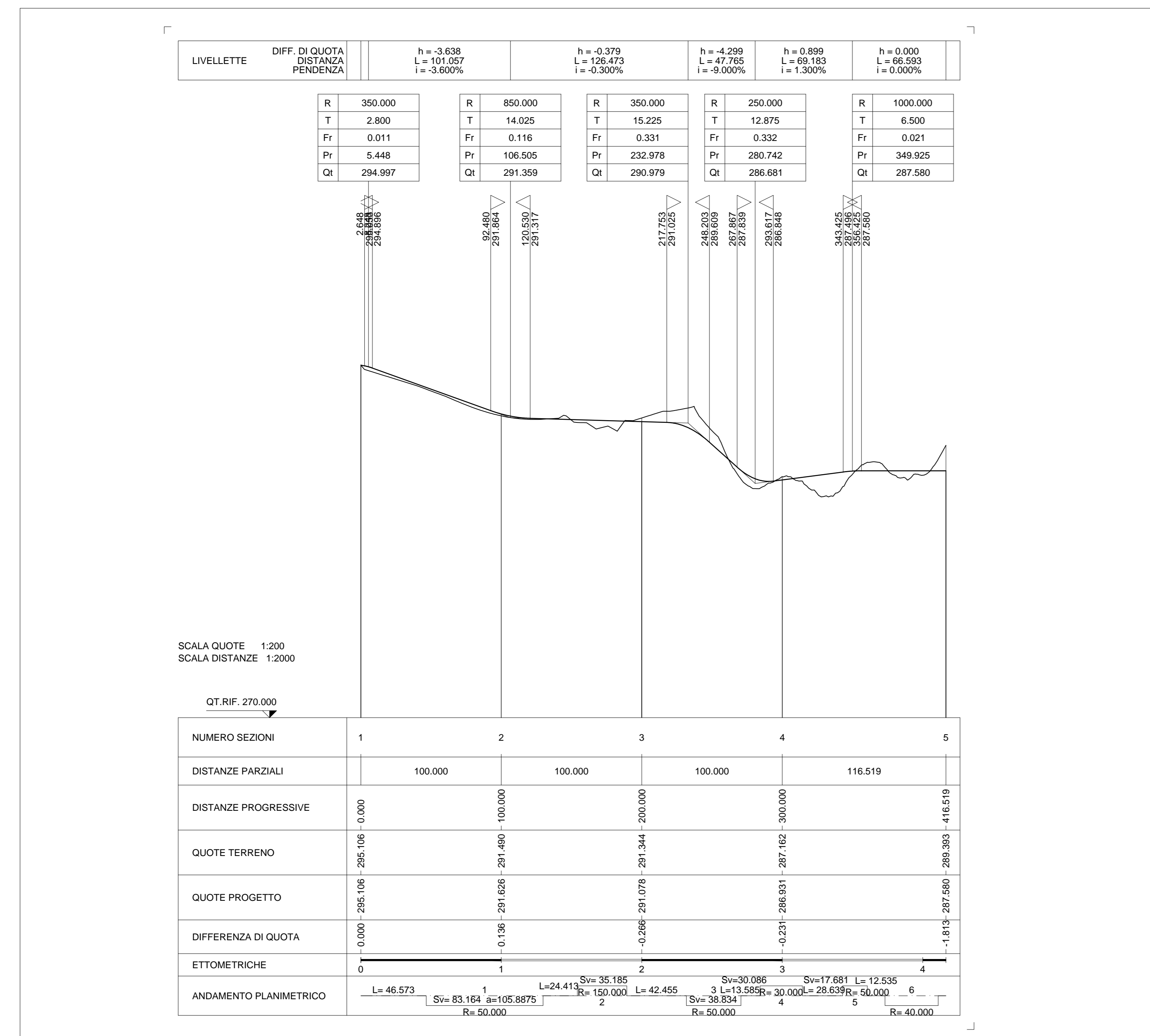
PROFILO LONGITUDINALE PISTA DI CANTIERE A SERVIZIO PER LA REALIZZAZIONE DEI MICROPALI DELL'IMBOCCO SUD GALLERIA COGOLLO scala 1:2000/200
