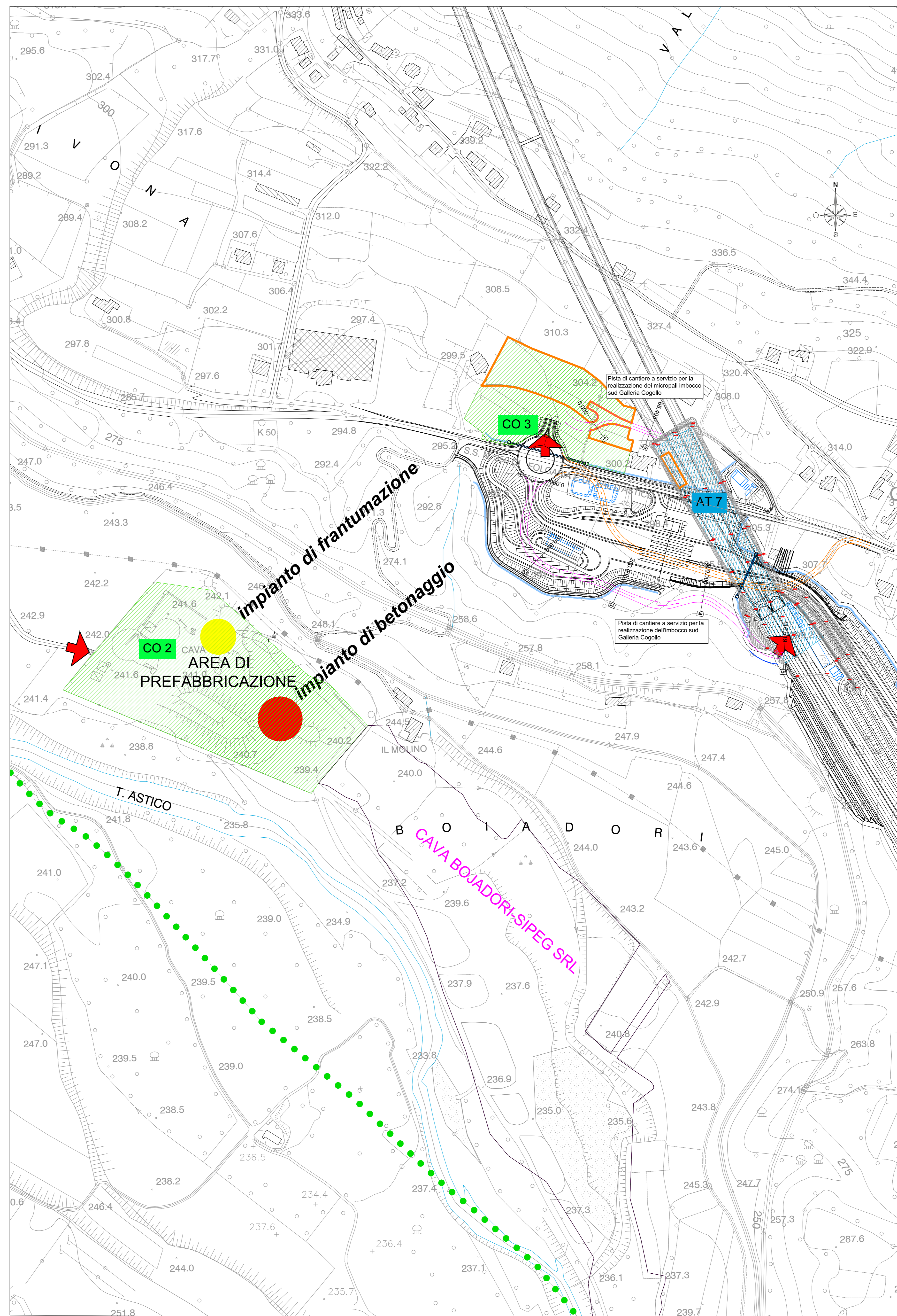
PLANIMETRIA DI PROGETTO IMBOCCO SUD GALLERIA COGOLLO - PISTE DI CANTIERE - TAV 2 scala 1:2000
