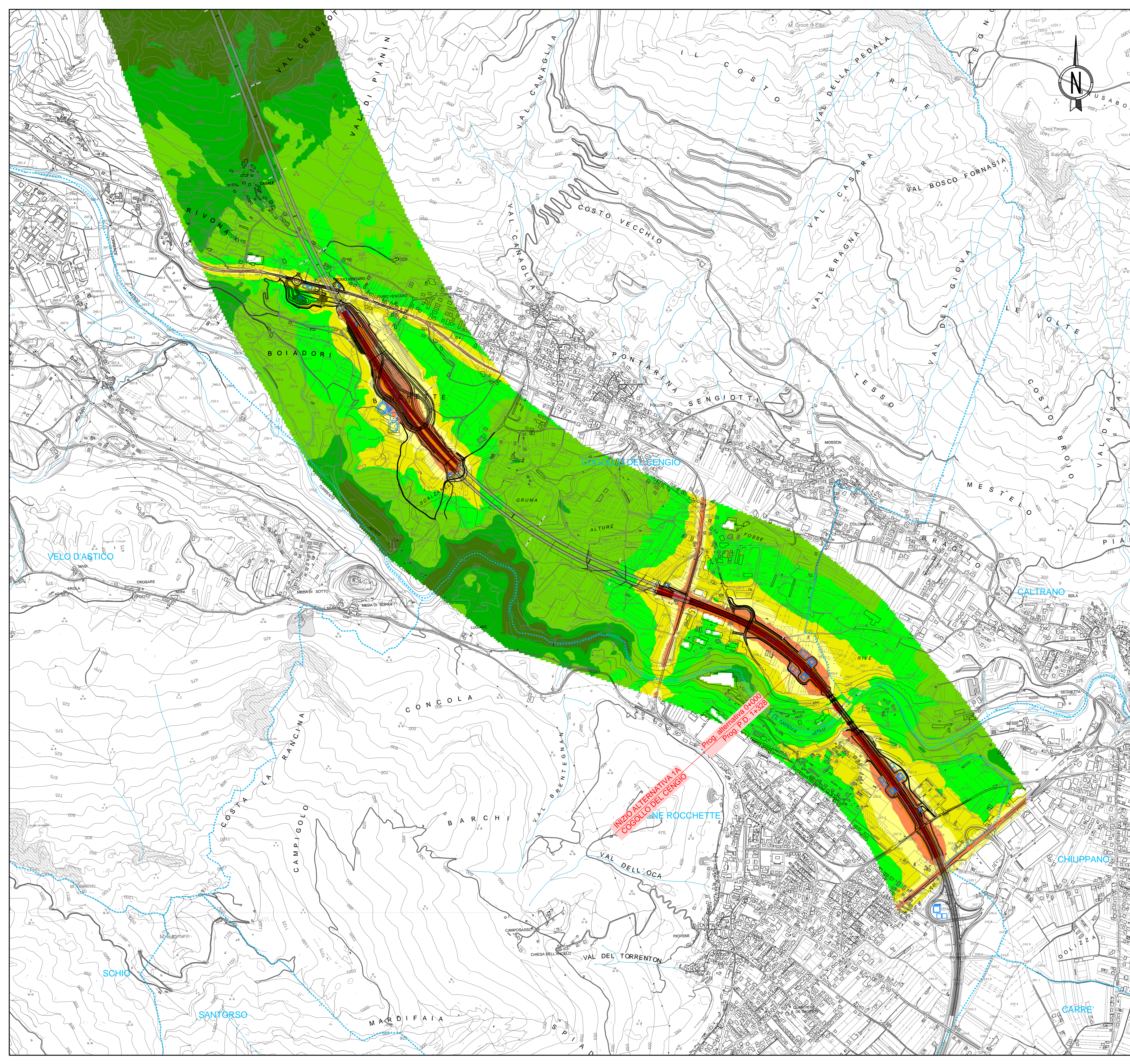
LIVELLO SONORO CONTINUO EQUIVALENTE dB(A)
