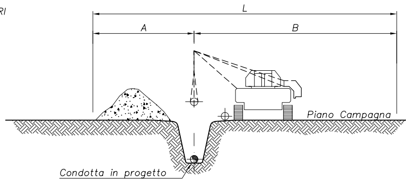
PISTA DI LAVORO TIPICA
