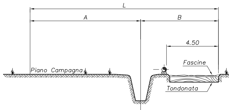
PISTA DI LAVORO IN PALUDE
