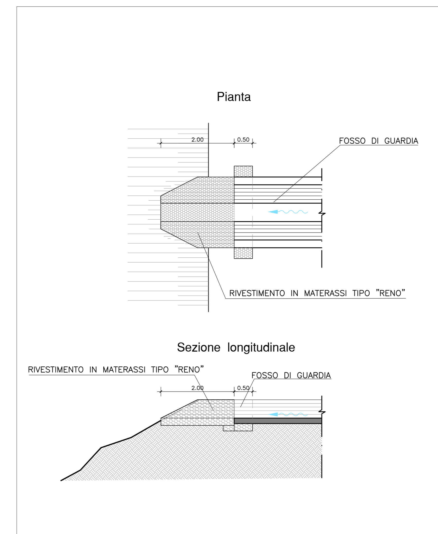
PARTICOLARE SCARICO FOSSI DI GUARDIA - Scala 1:10 -
