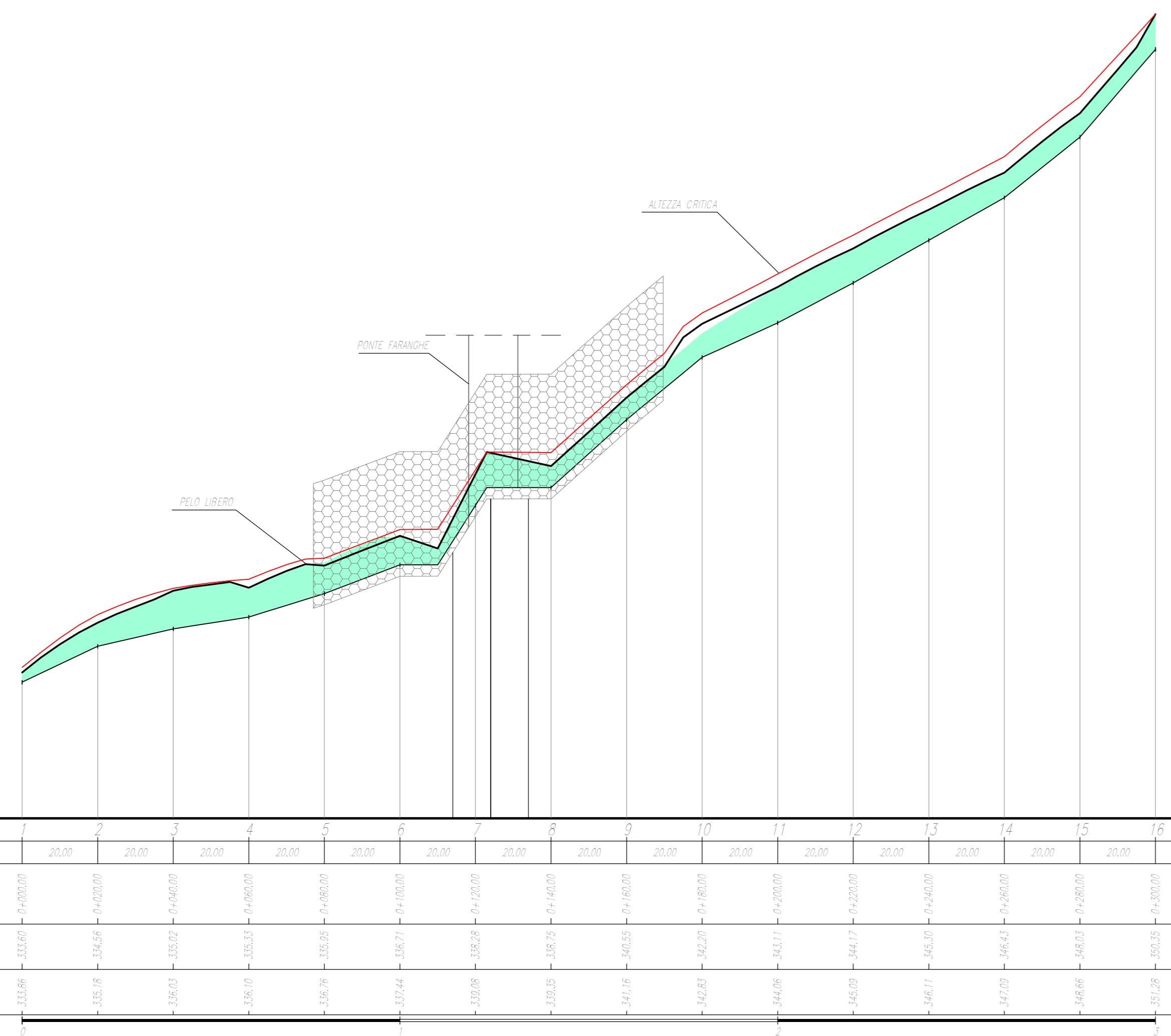
PROFILO LONGITUDINALE - Scala 1:1000/100 -
