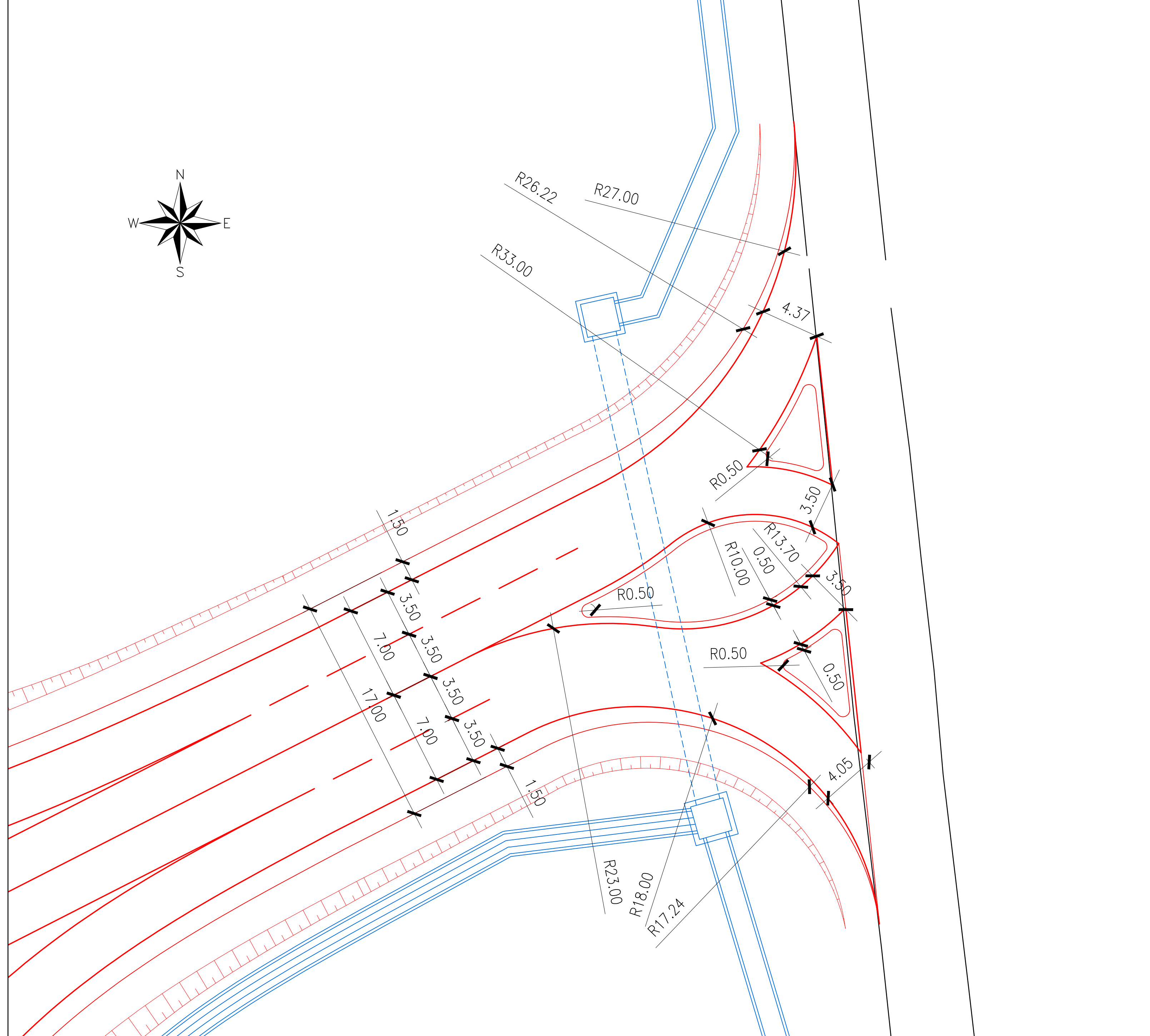
INTERSEZIONE A T (SVINCOLO DI MATELICA SUD)
