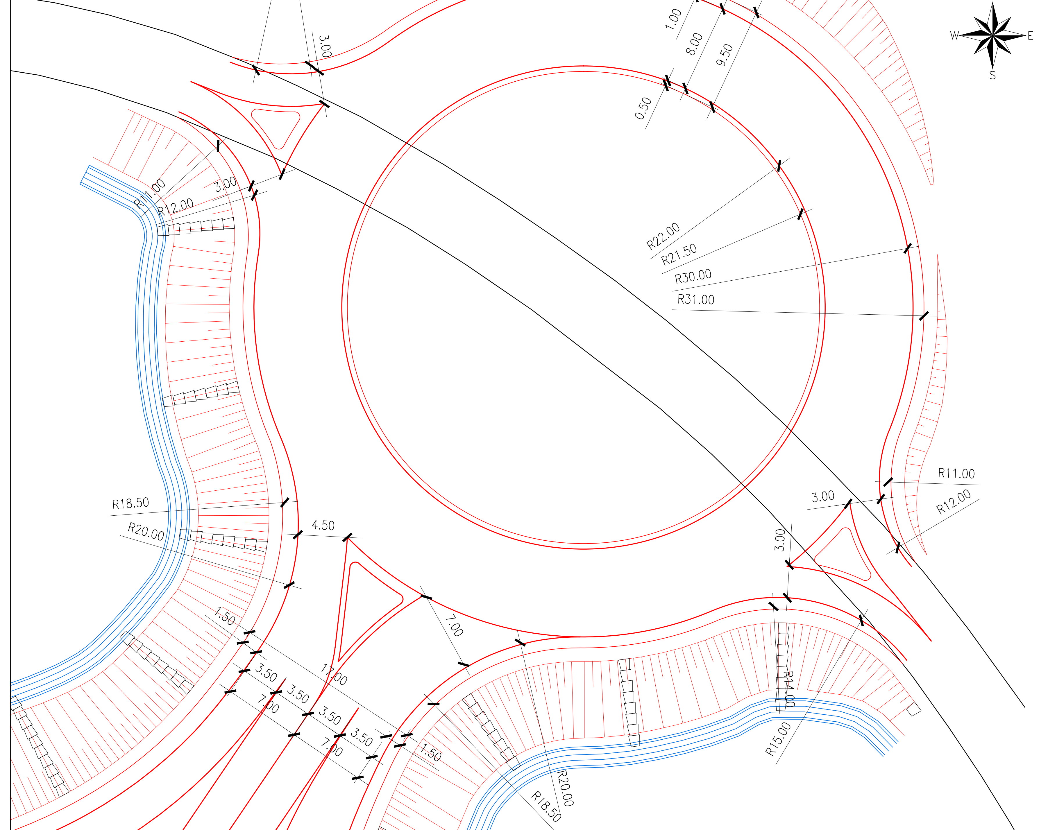
Intersezione a rotatoria (Svincolo di Castelraimondo Nord)
