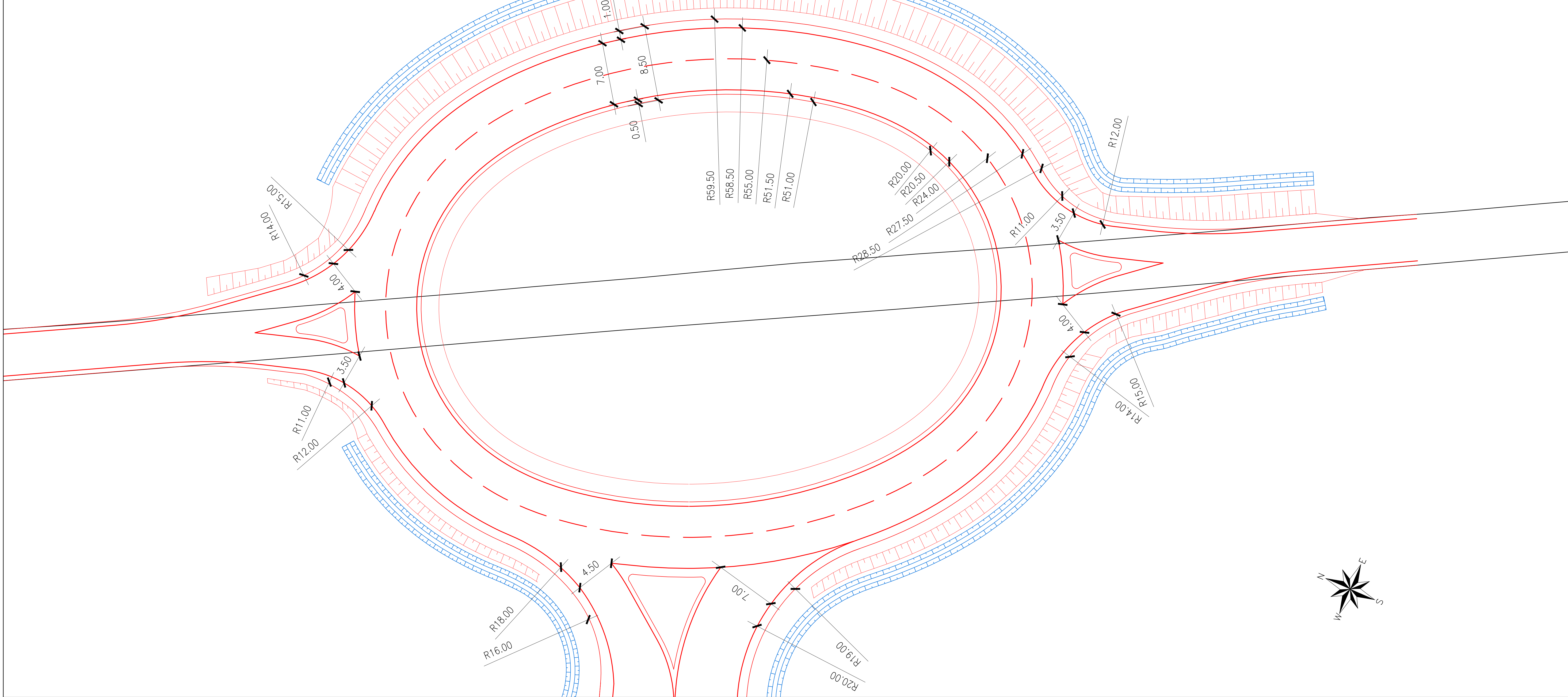
SISTEMAZIONE CON "CIRCOLAZIONE ROTATORIA" (SVINCOLO DI MATELICA OVEST)
