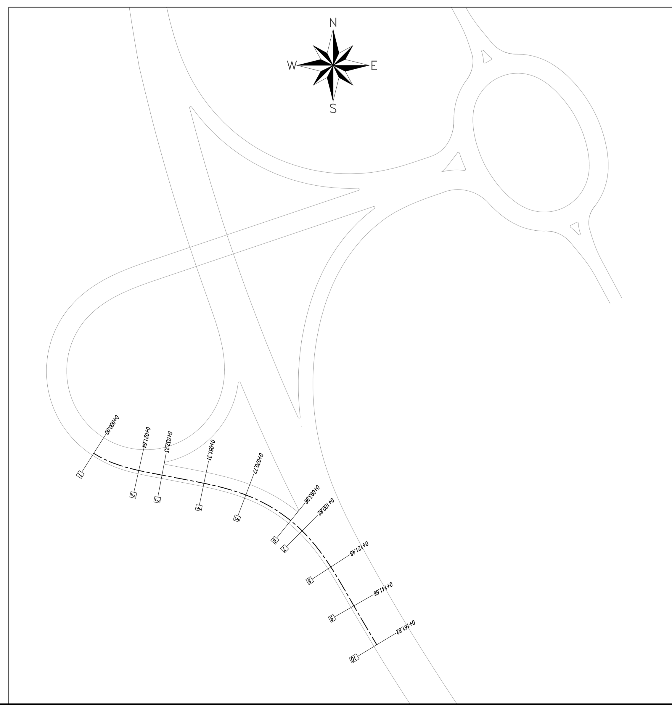
POSIZIONE PLANIMETRICA PICC. RAMPA B-D - Scala 1:1000
