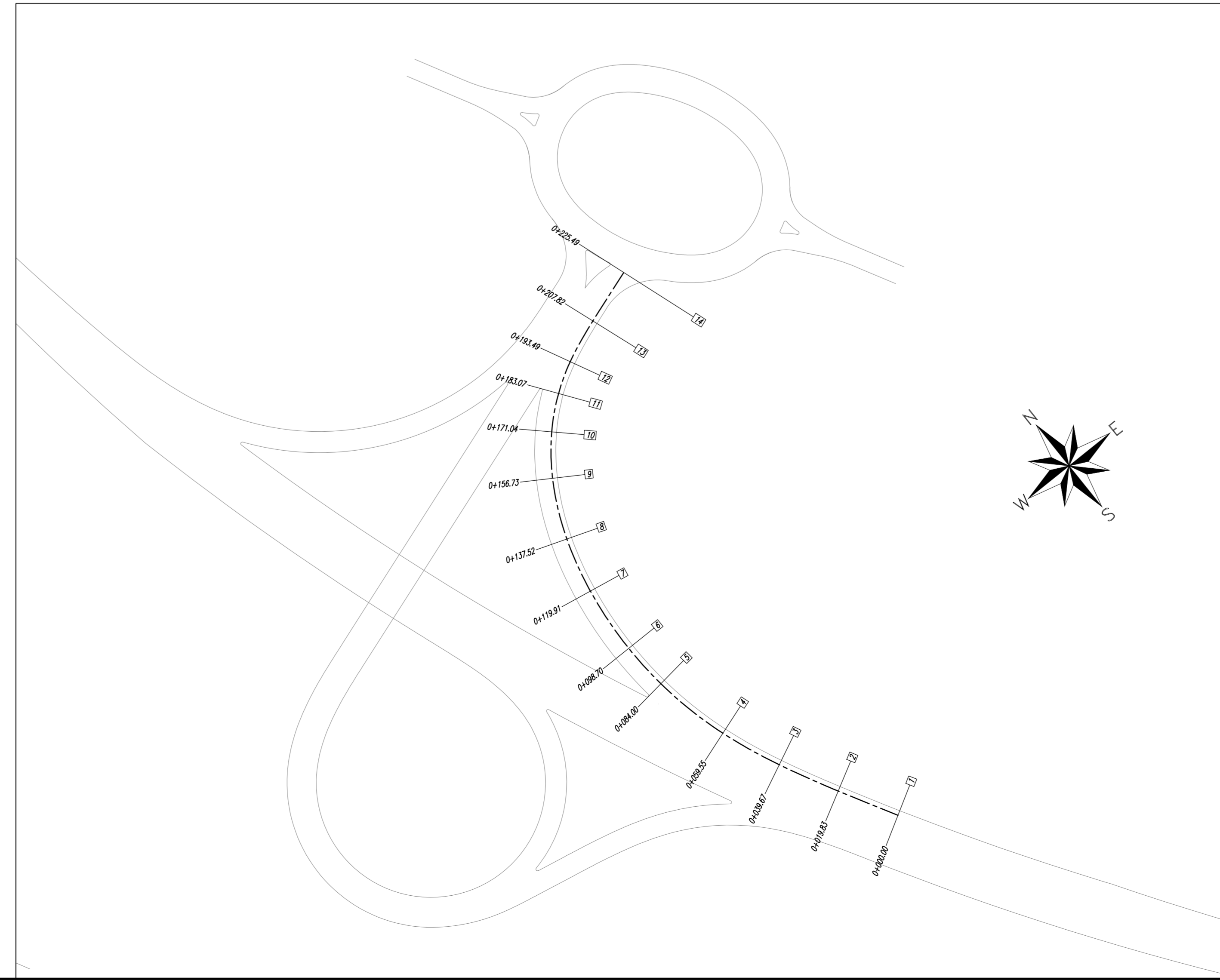
POSIZIONE PLANIMETRICA PICC. RAMPA E-F - Scala 1:1000
