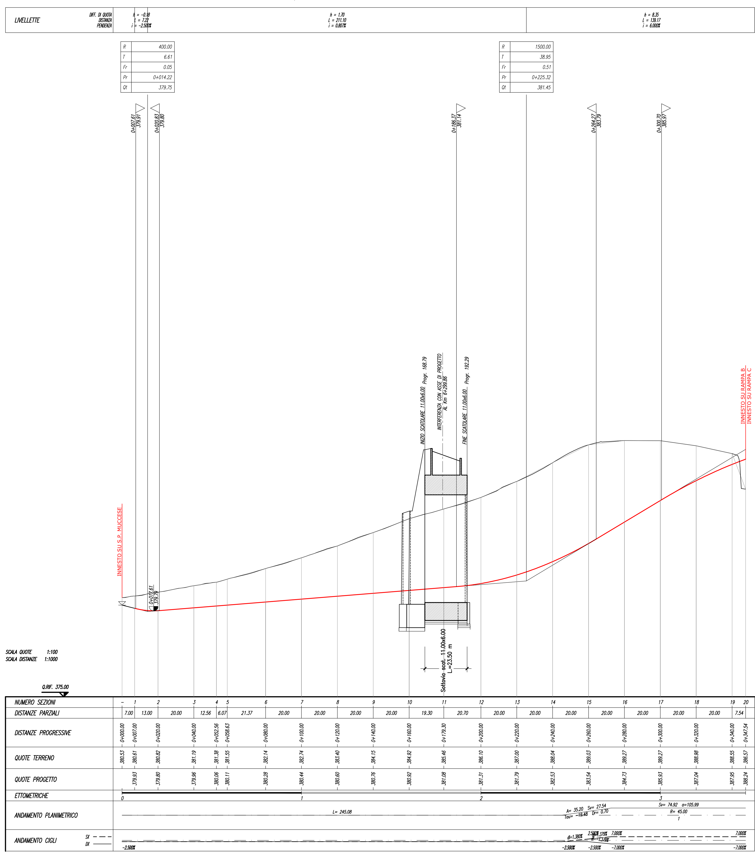
PROFILO LONGITUDINALE RAMPA A - Scala 1:1000/100
