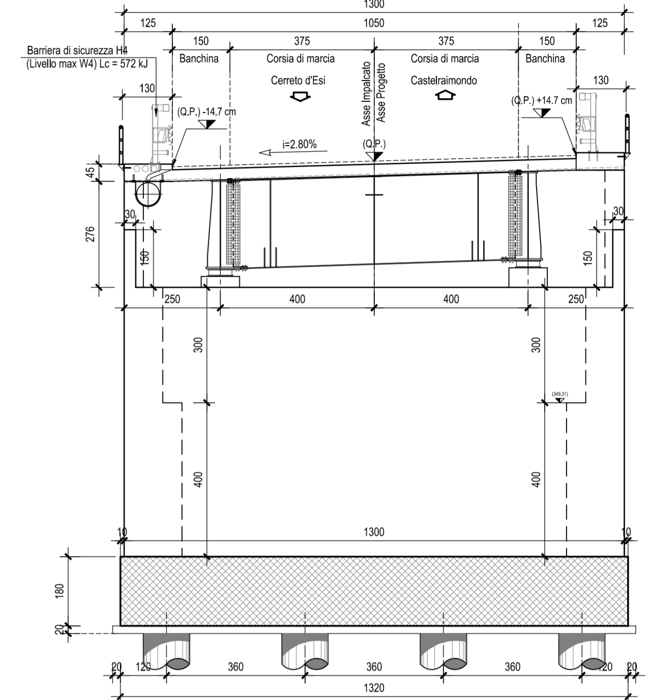
SEZIONE TRASVERSALE-Scala 1:100 (IN CORRISPONDENZA DELLA SPALLA)
