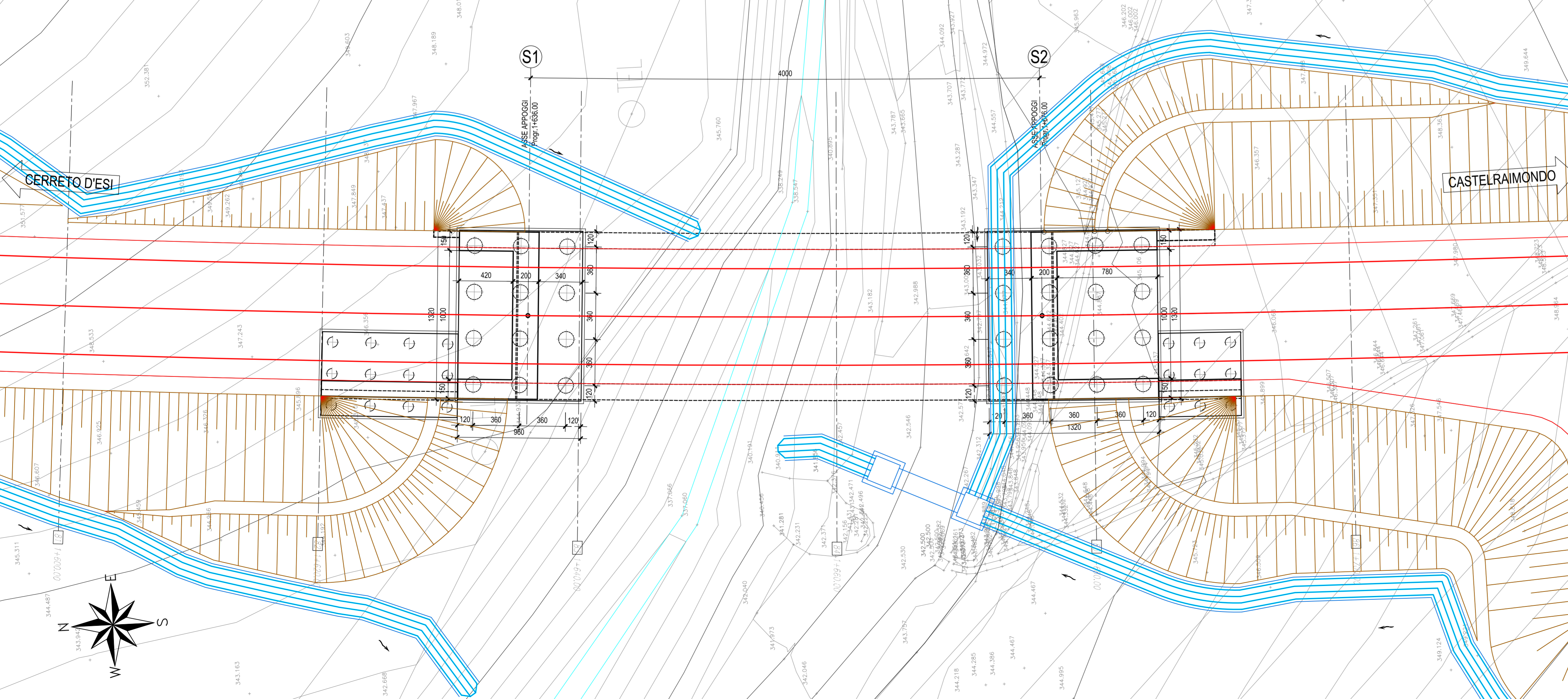
PIANTA FONDAZIONE-Scala 1:200
