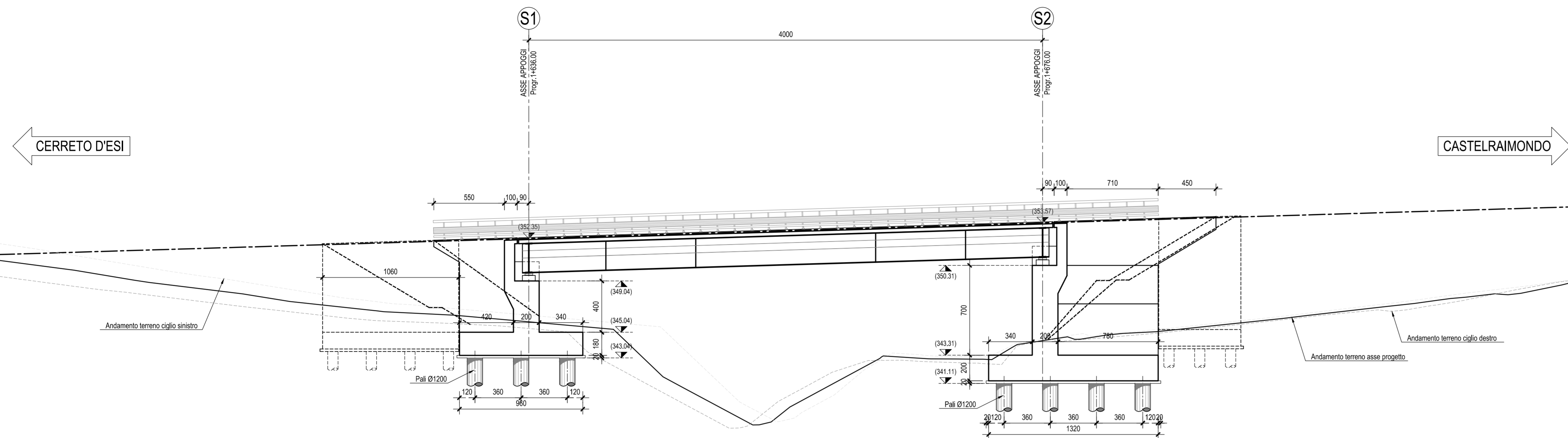
SEZIONE LONGITUDINALE-Scala 1:200
