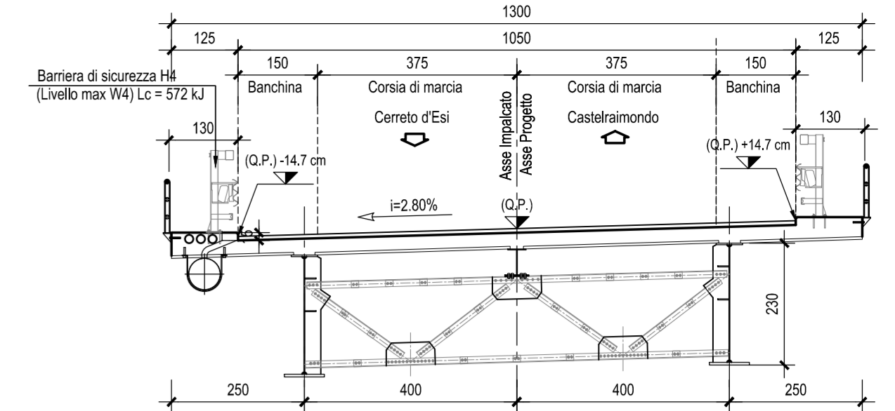
SEZIONE TRASVERSALE-Scala 1:100 (IN CORRISPONDENZA DELLA SPALLA)
