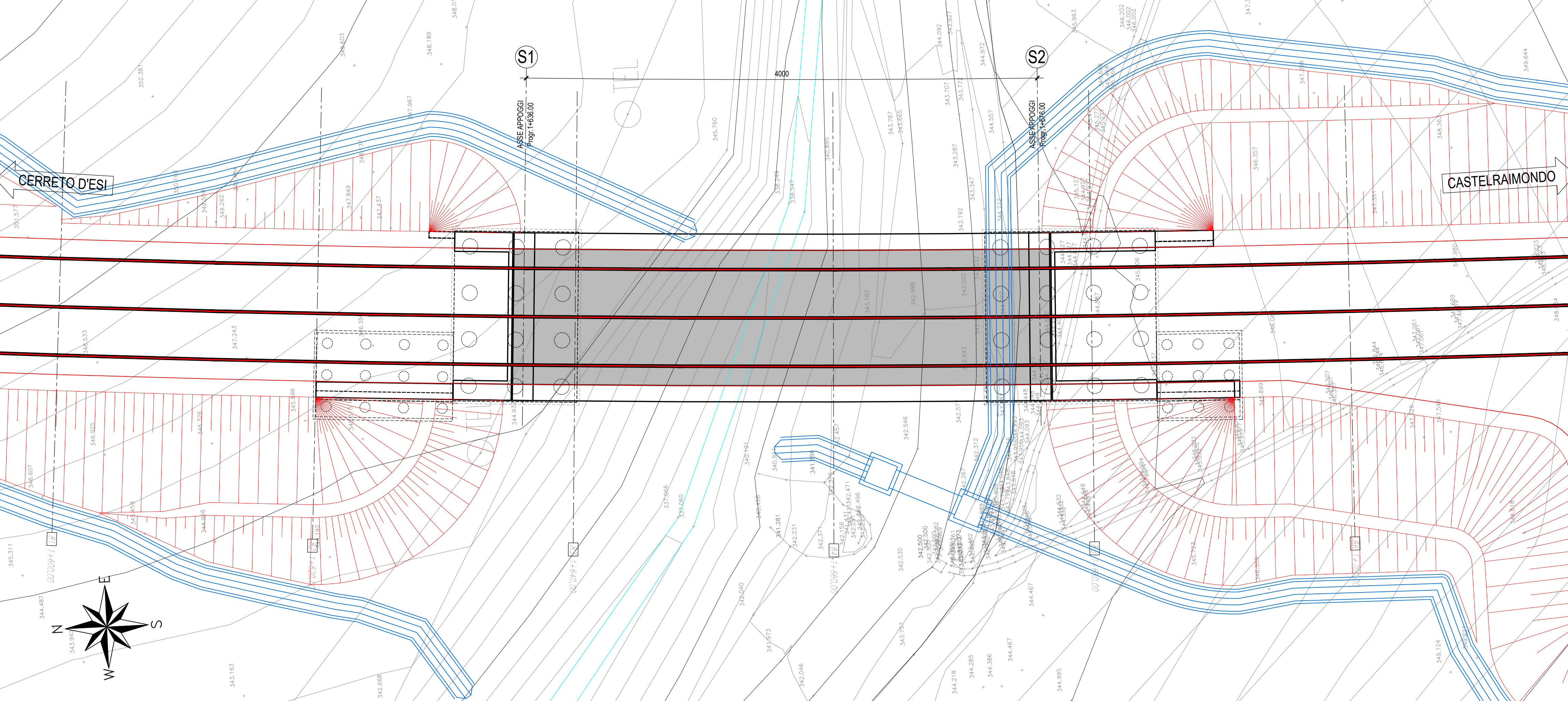
PIANTA IMPALCATO-Scala 1:200
