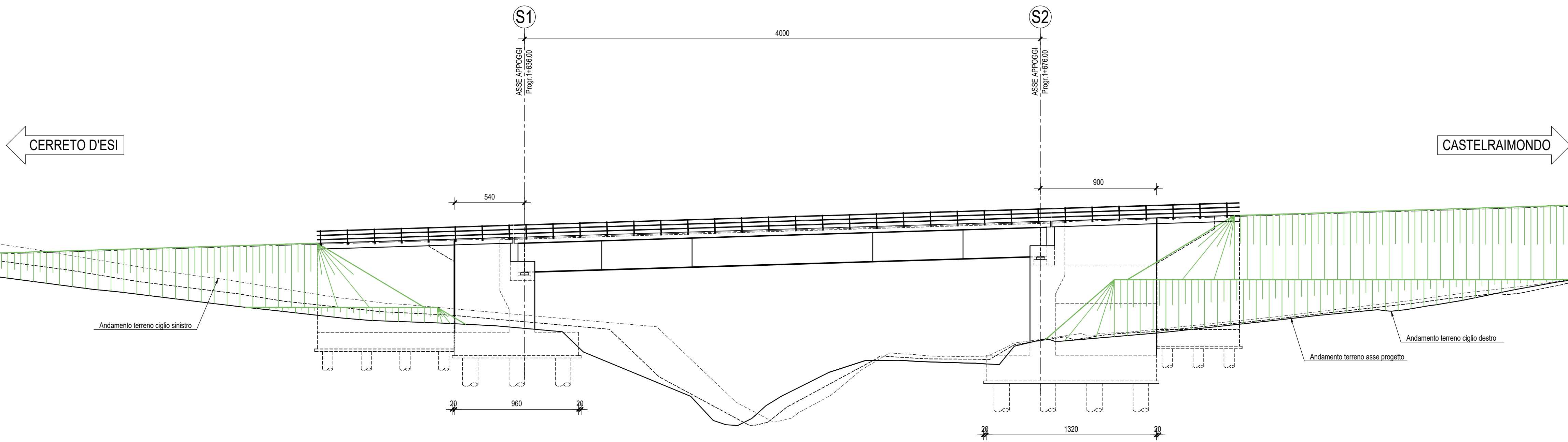
PROSPETTO-Scala 1:200
