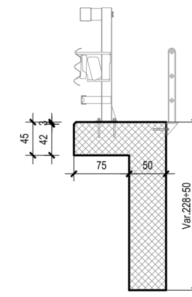
SEZIONE E-E-Scala 1:50
