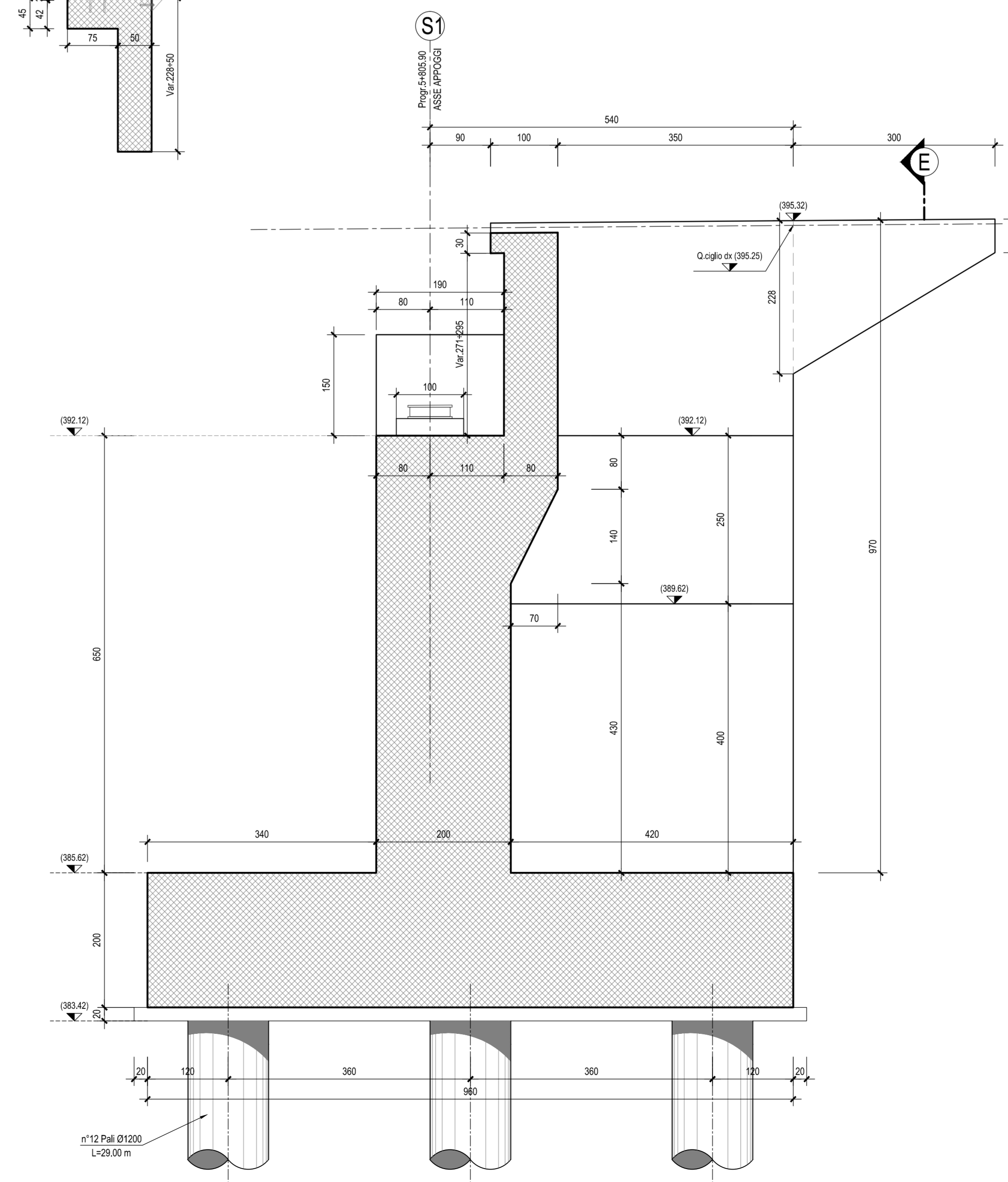
SEZIONE A'-A'-Scala 1:50
