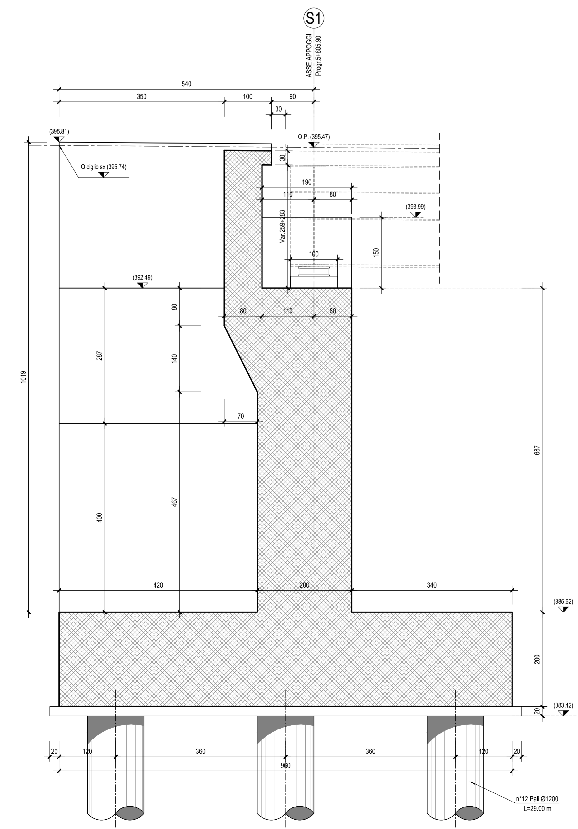
SEZIONE A-A-Scala 1:50
