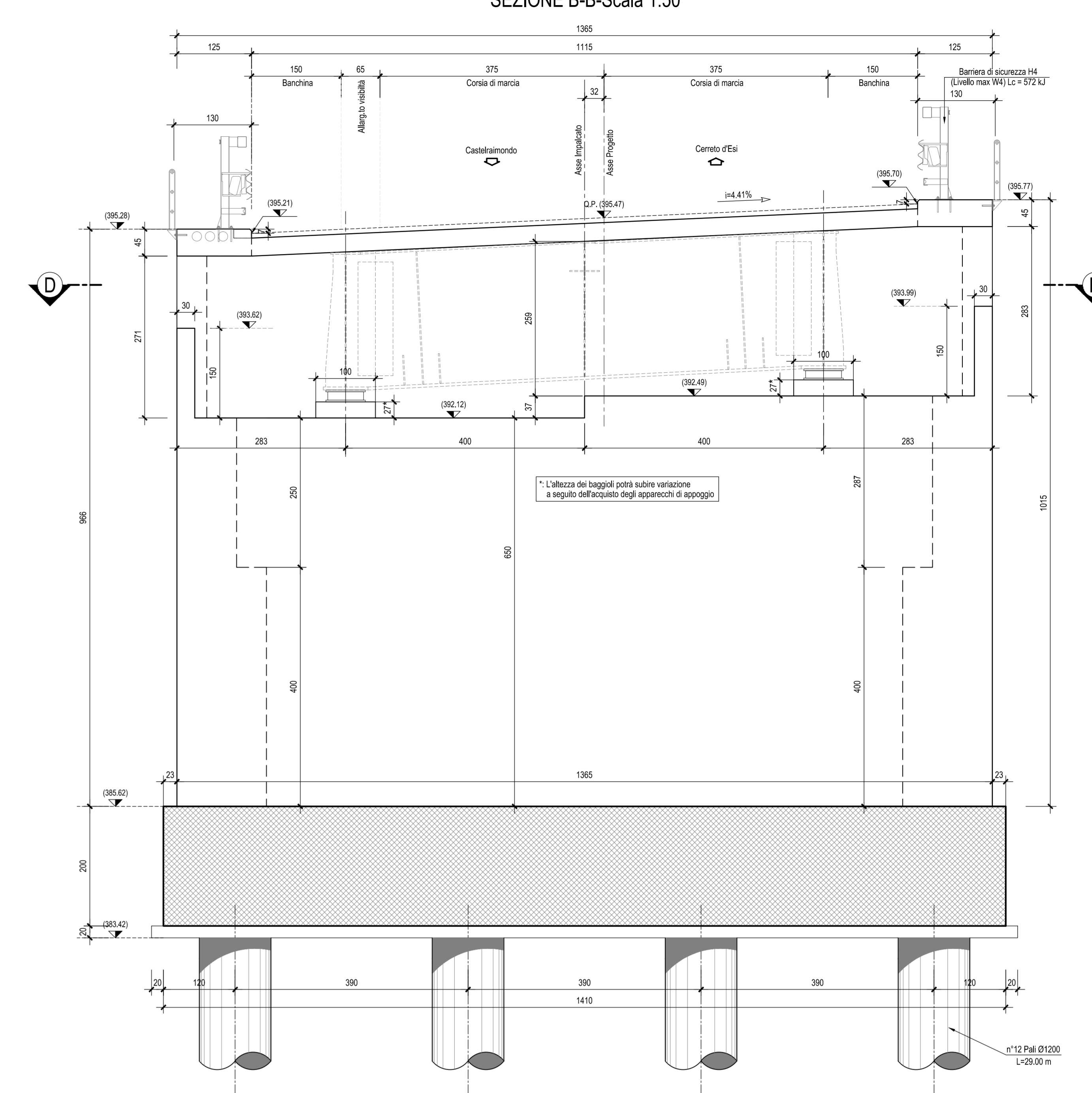
SEZIONE B-B-Scala 1:50
