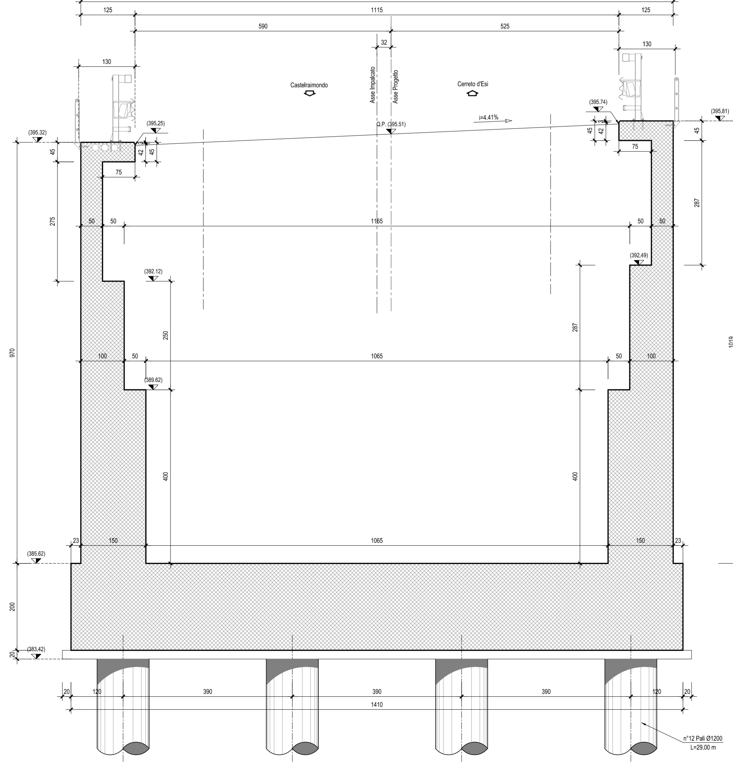
SEZIONE C-C-Scala 1:50
