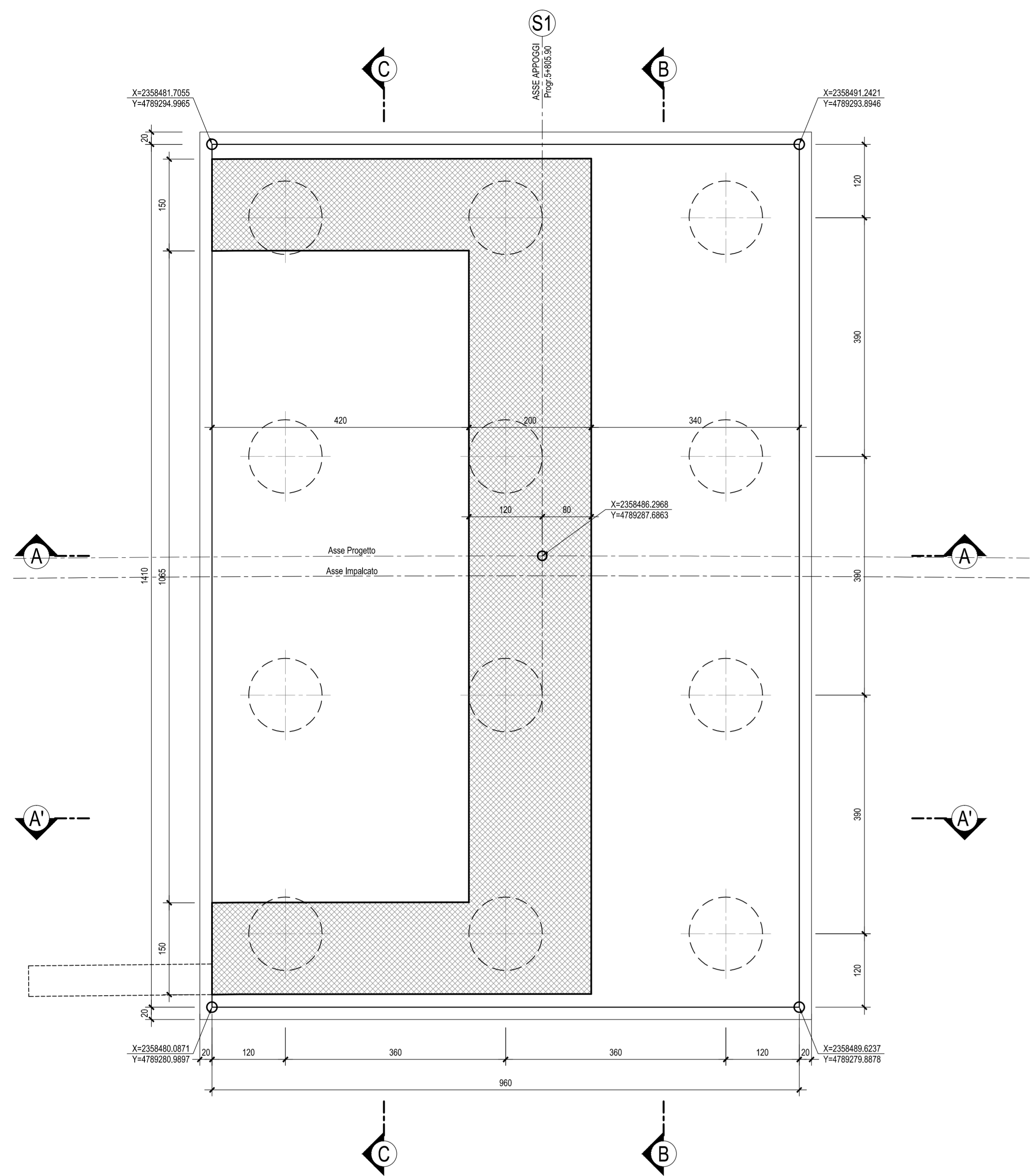
PIANTA FONDAZIONI-Scala 1:50
