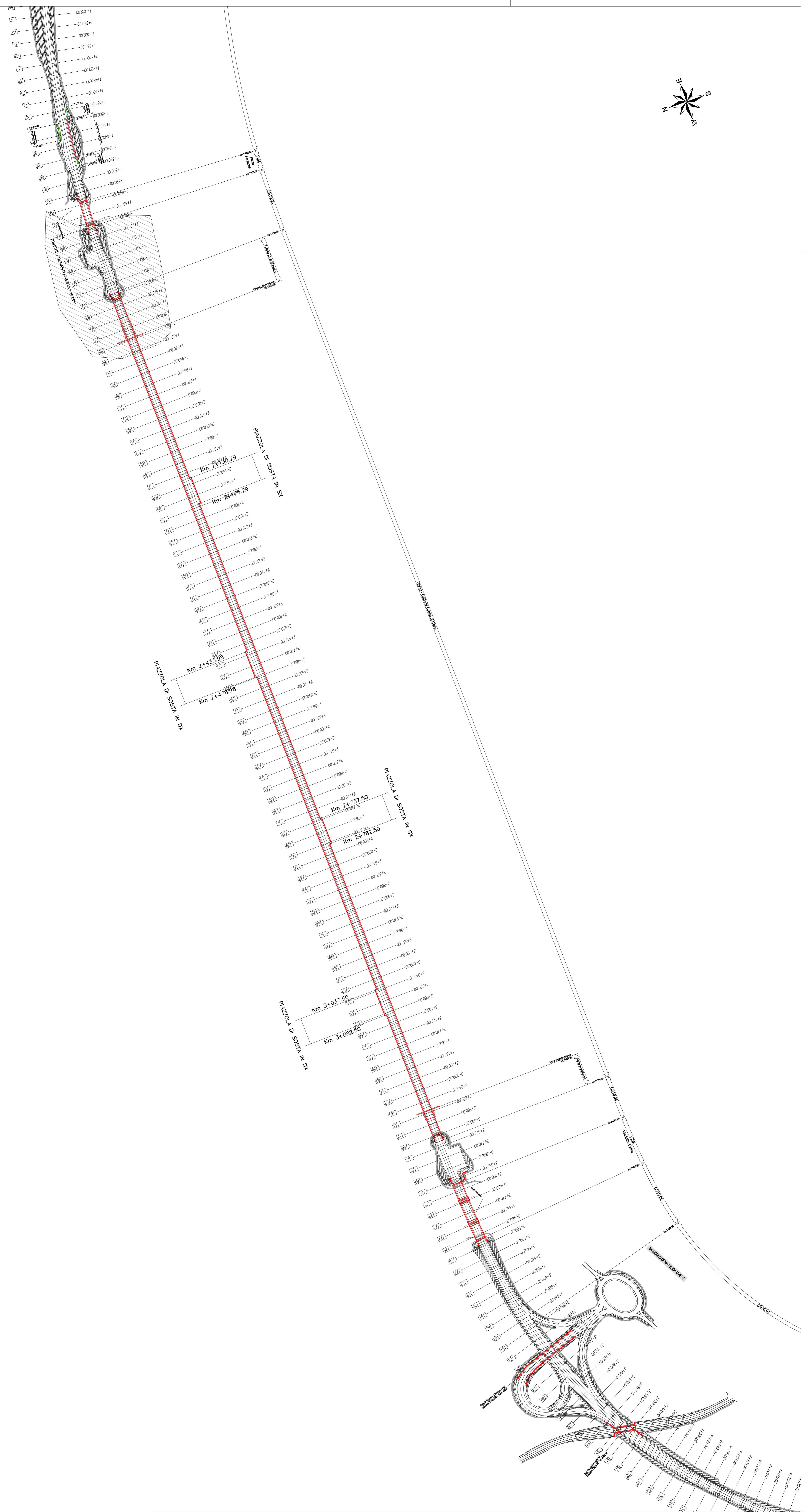
Key-plan
