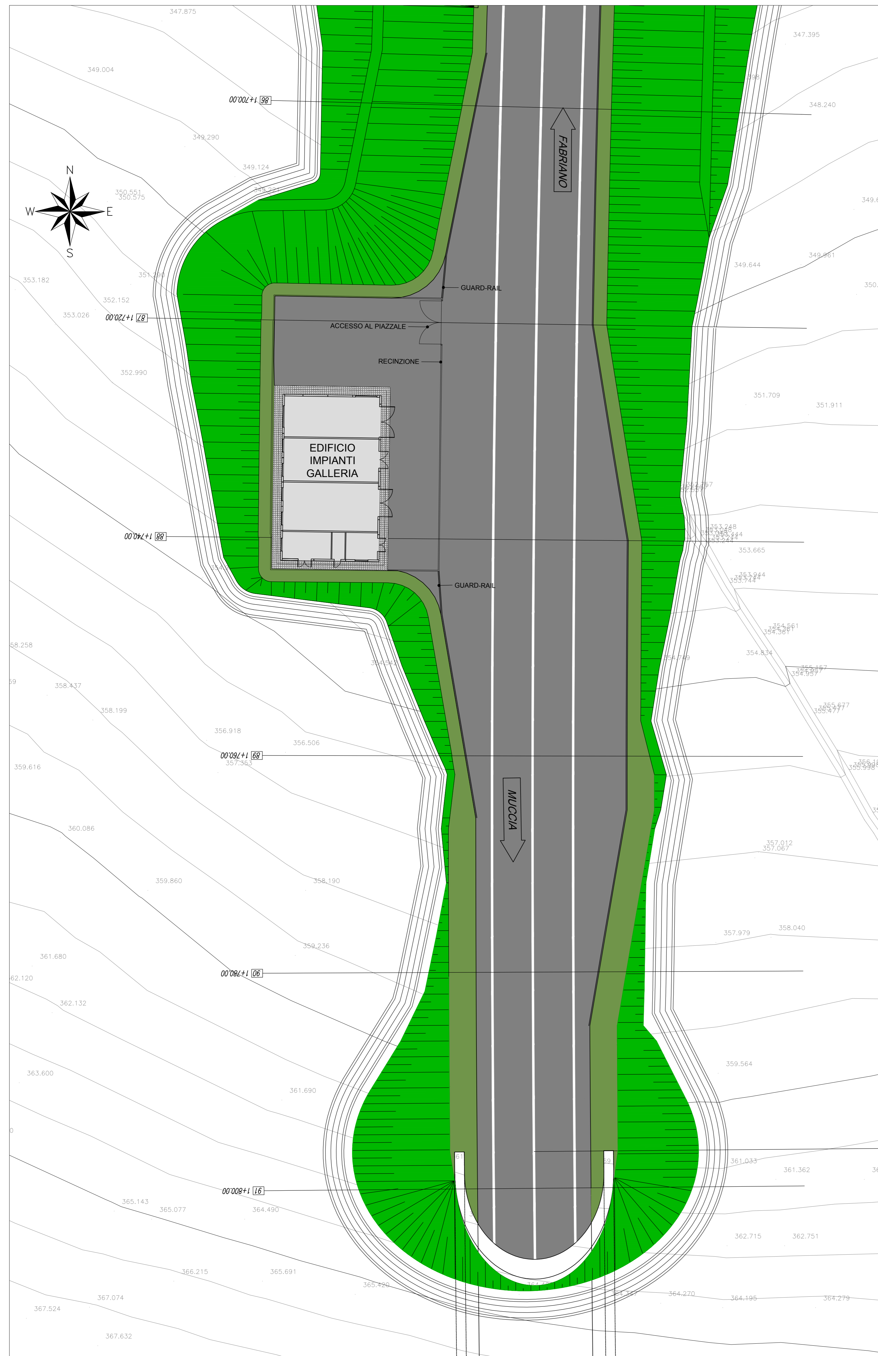
PLANIMETRIA PIAZZALE IMBOCCO NORD - Scala 1:200 -
