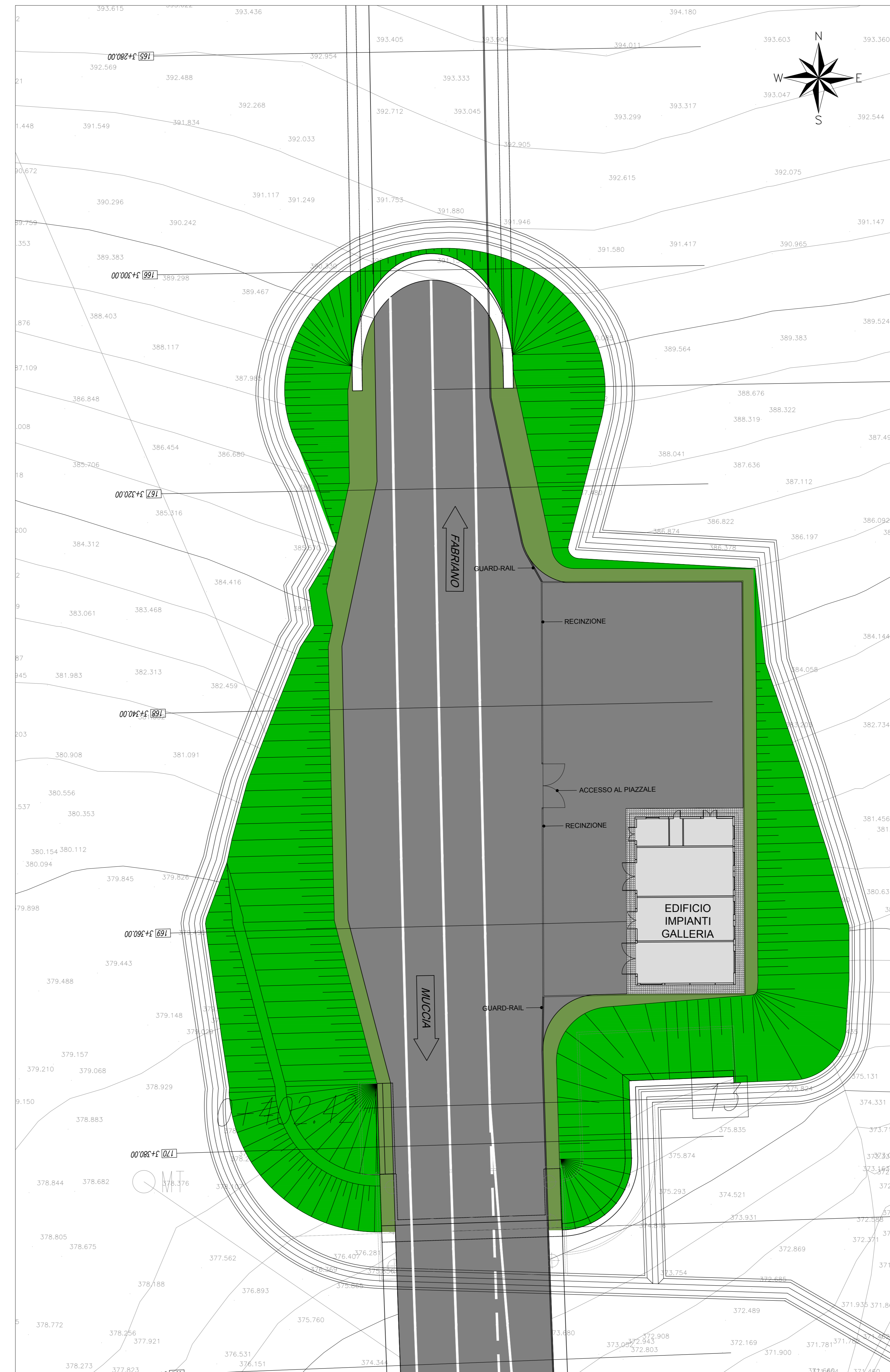
PLANIMETRIA PIAZZALE IMBOCCO SUD - Scala 1:200 -
