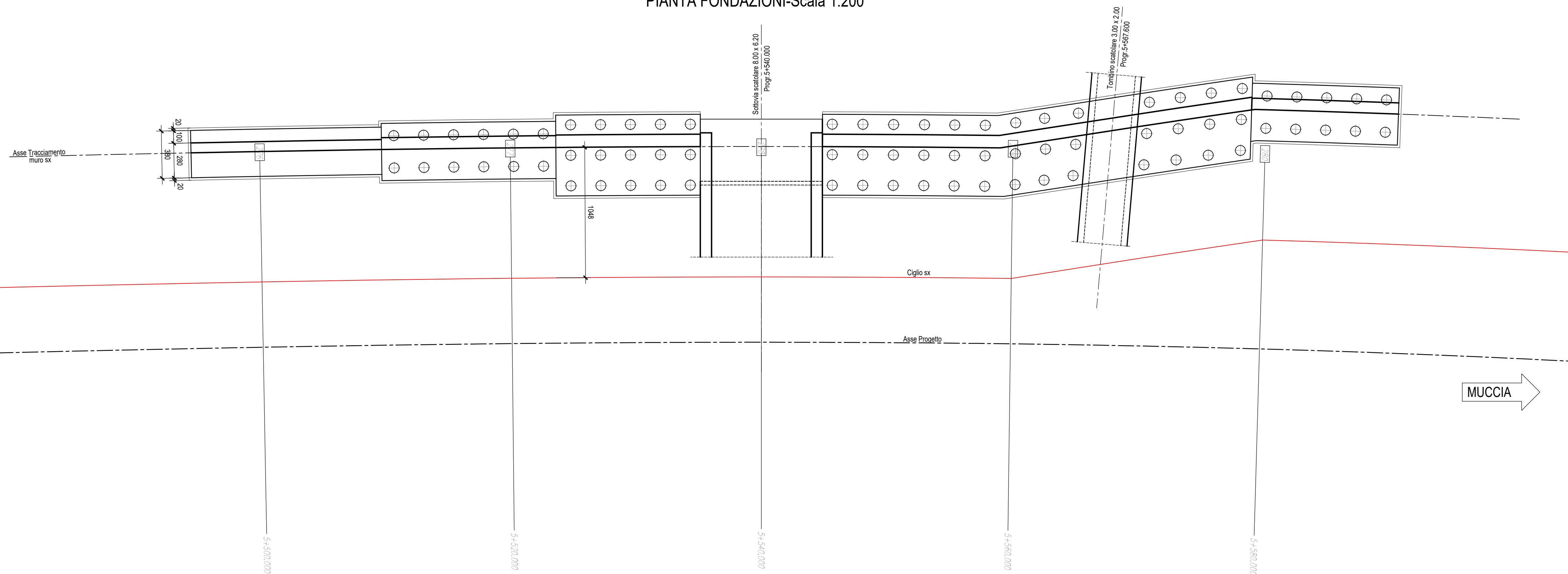
PIANTA FONDAZIONI-Scala 1:200
