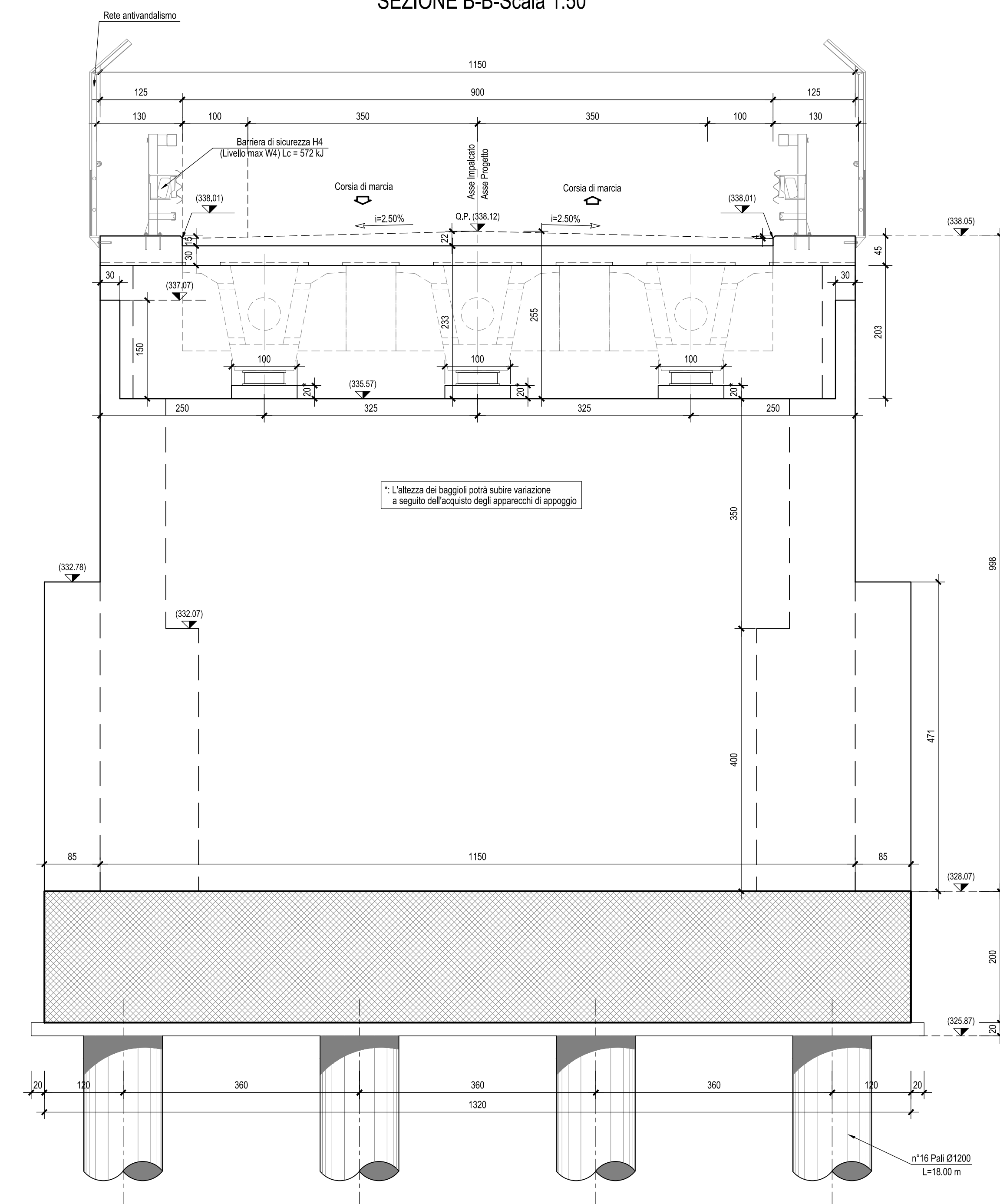
SEZIONE B-B-Scala 1:50
