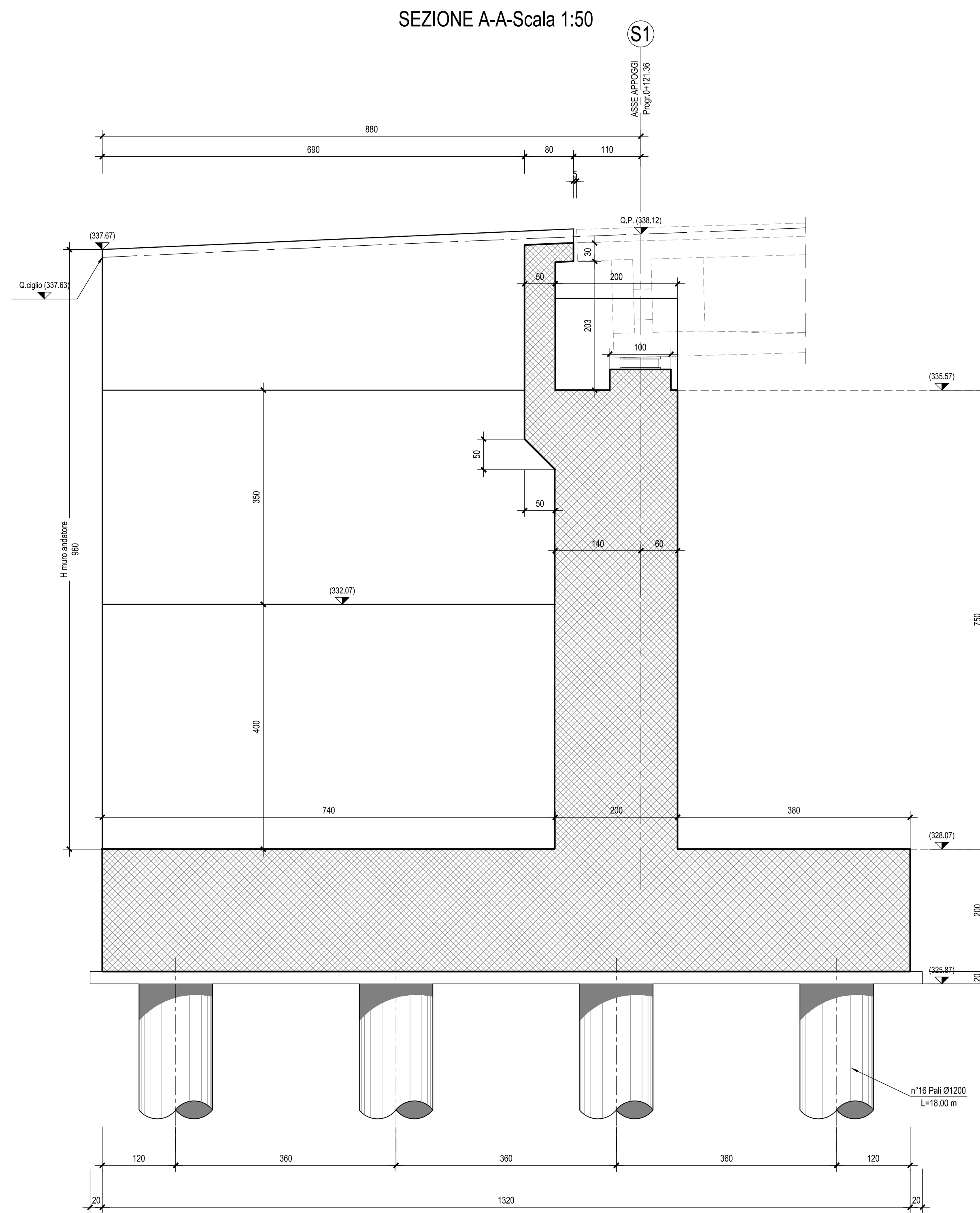
SEZIONE A-A-Scala 1:50
