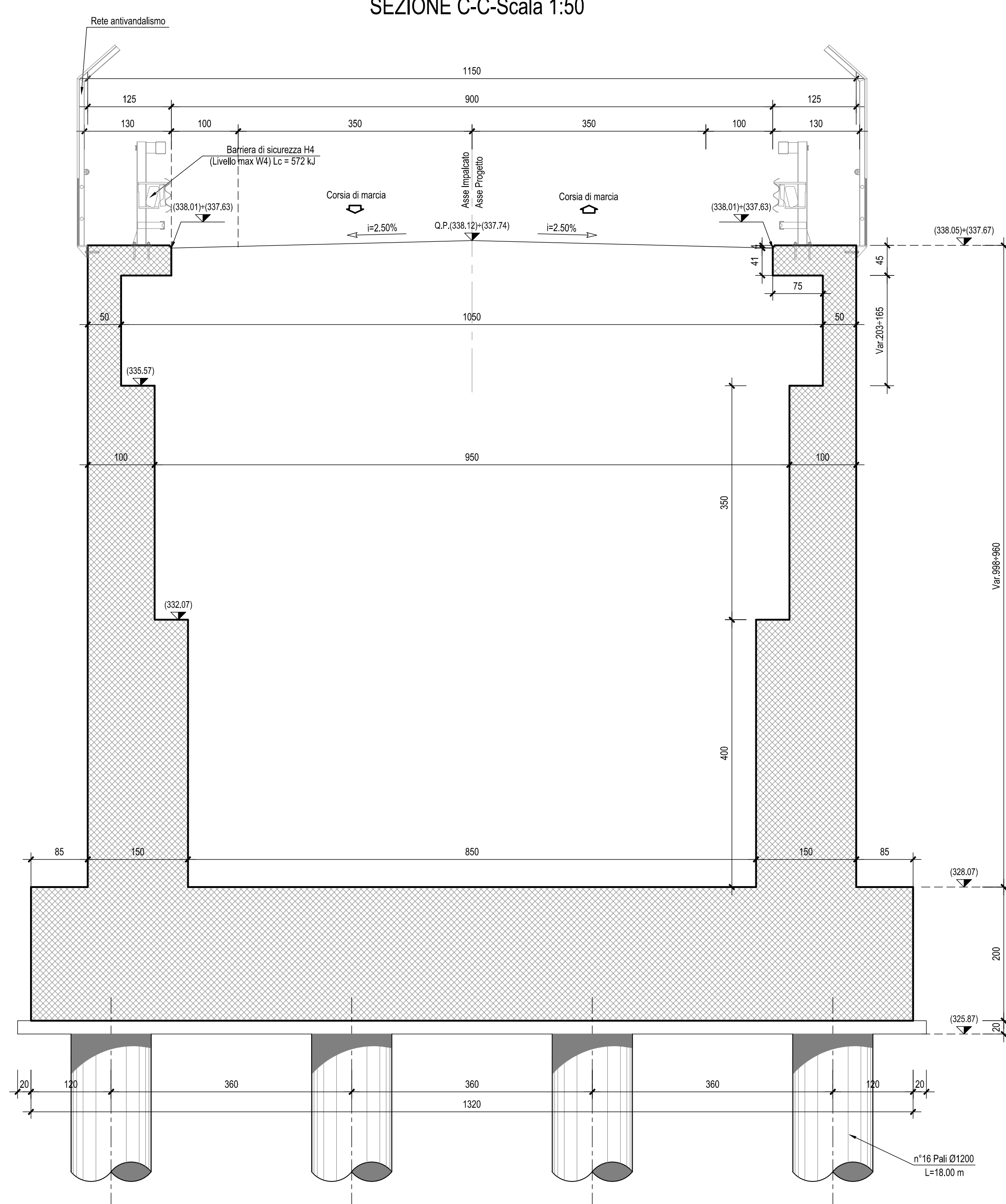
SEZIONE C-C-Scala 1:50
