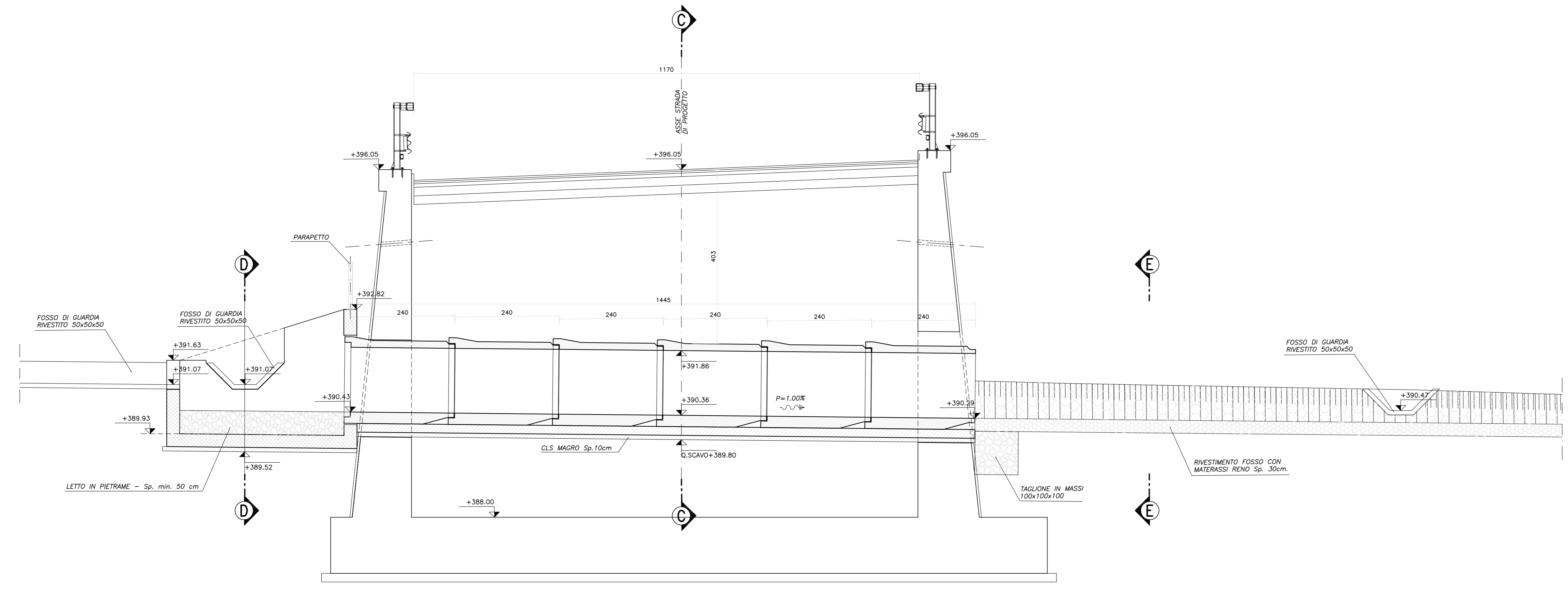
SEZIONE LONGITUDINALE A-A Scala 1:50
