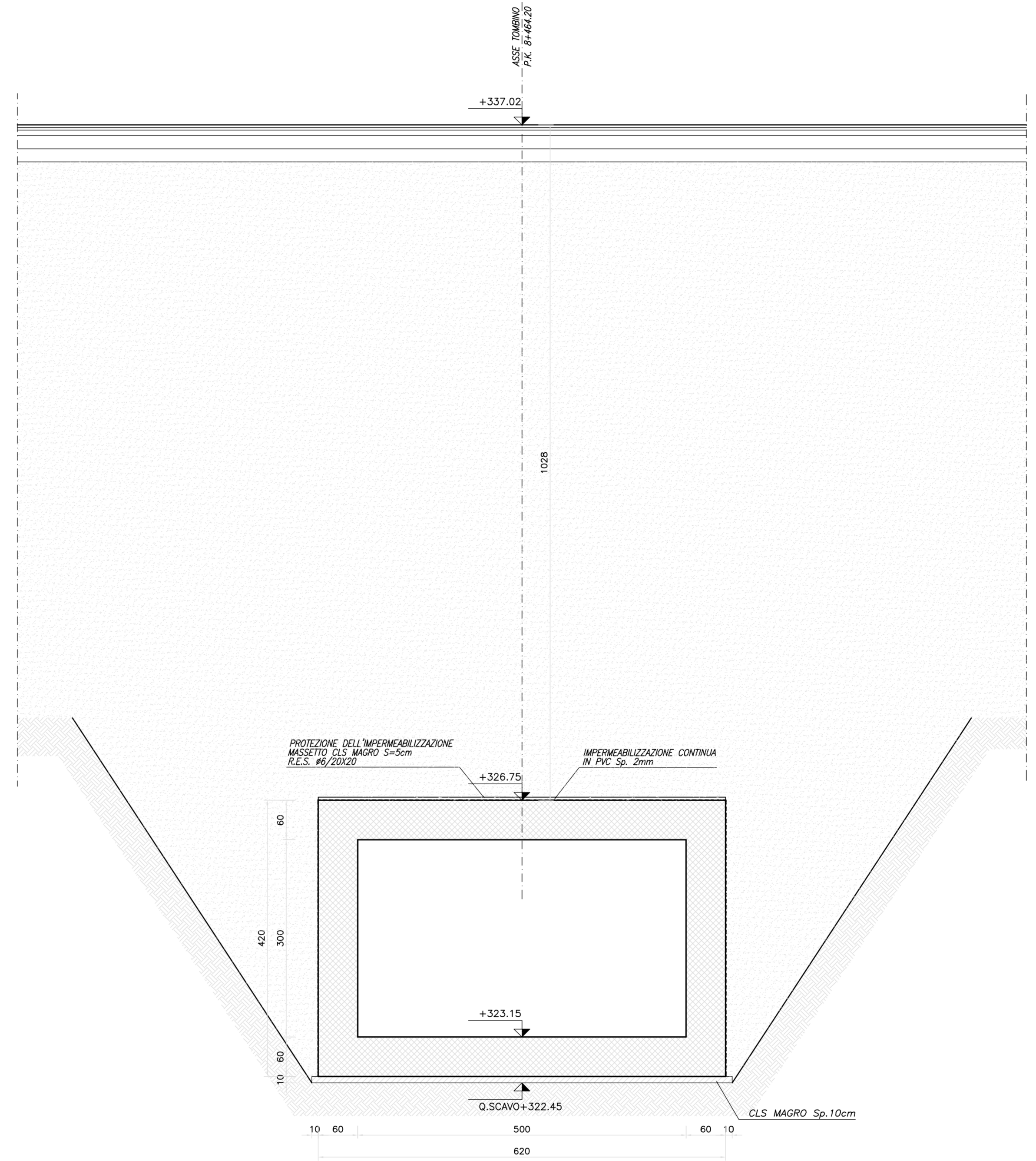
SEZIONE TRASVERSALE F-F Scala 1:50
