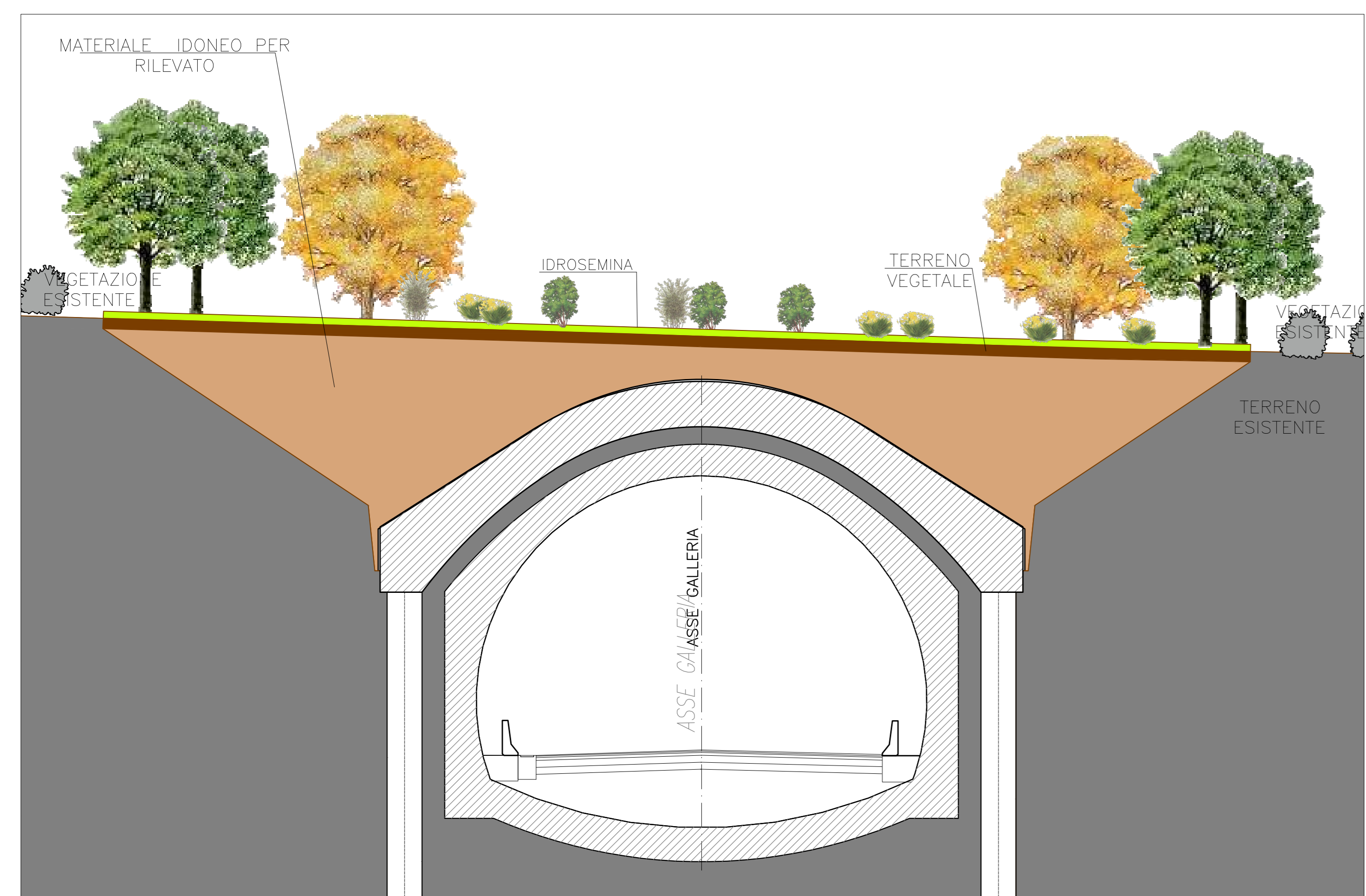
Sezione AB - Scala 1:100
