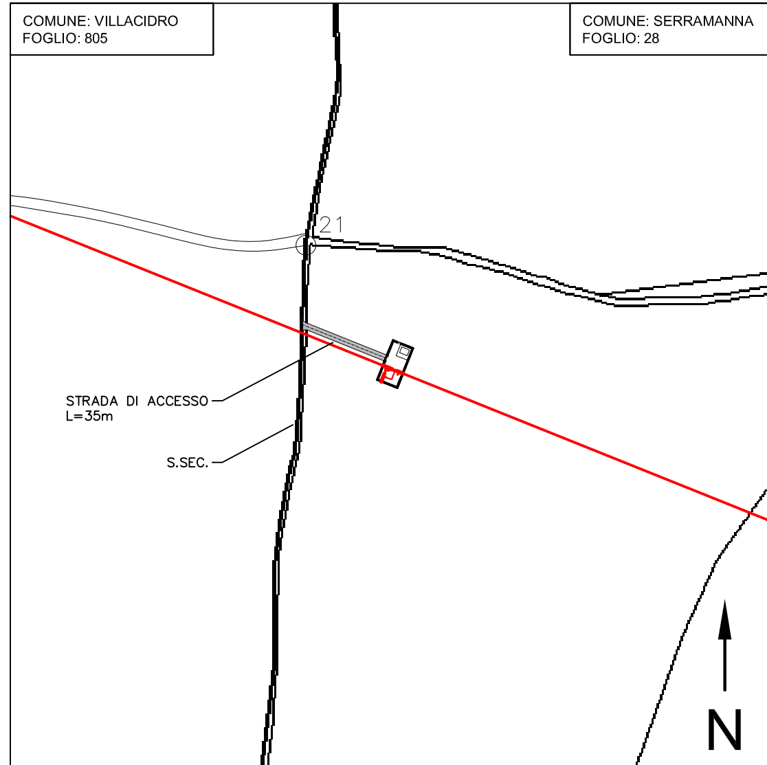
STRALCIO CATASTALE 1:2000
