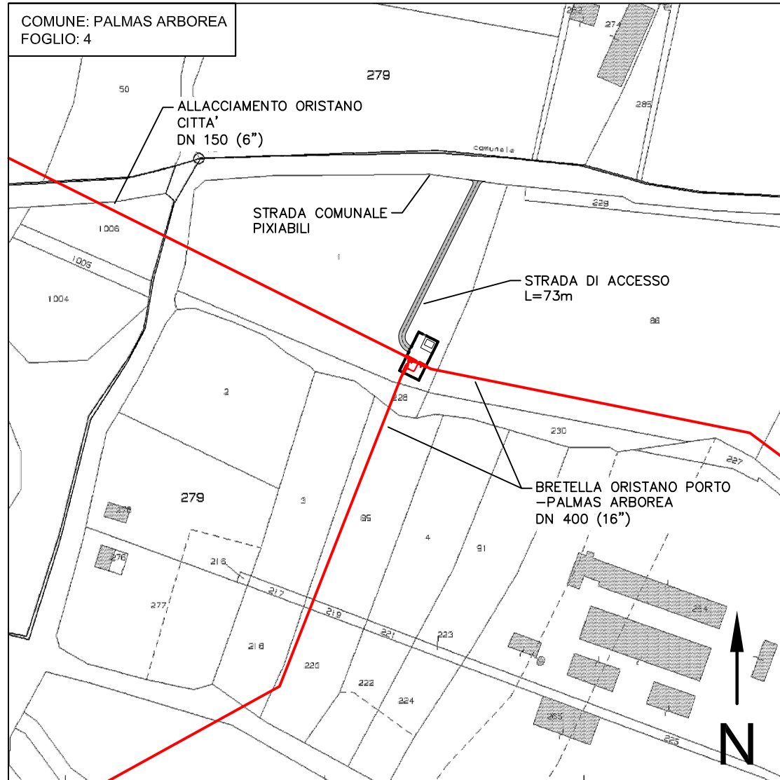
STRALCIO CATASTALE 1:2000
