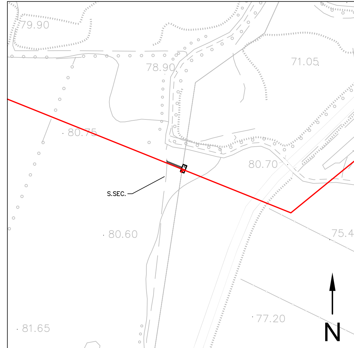
STRALCIO CTR 1:5000
