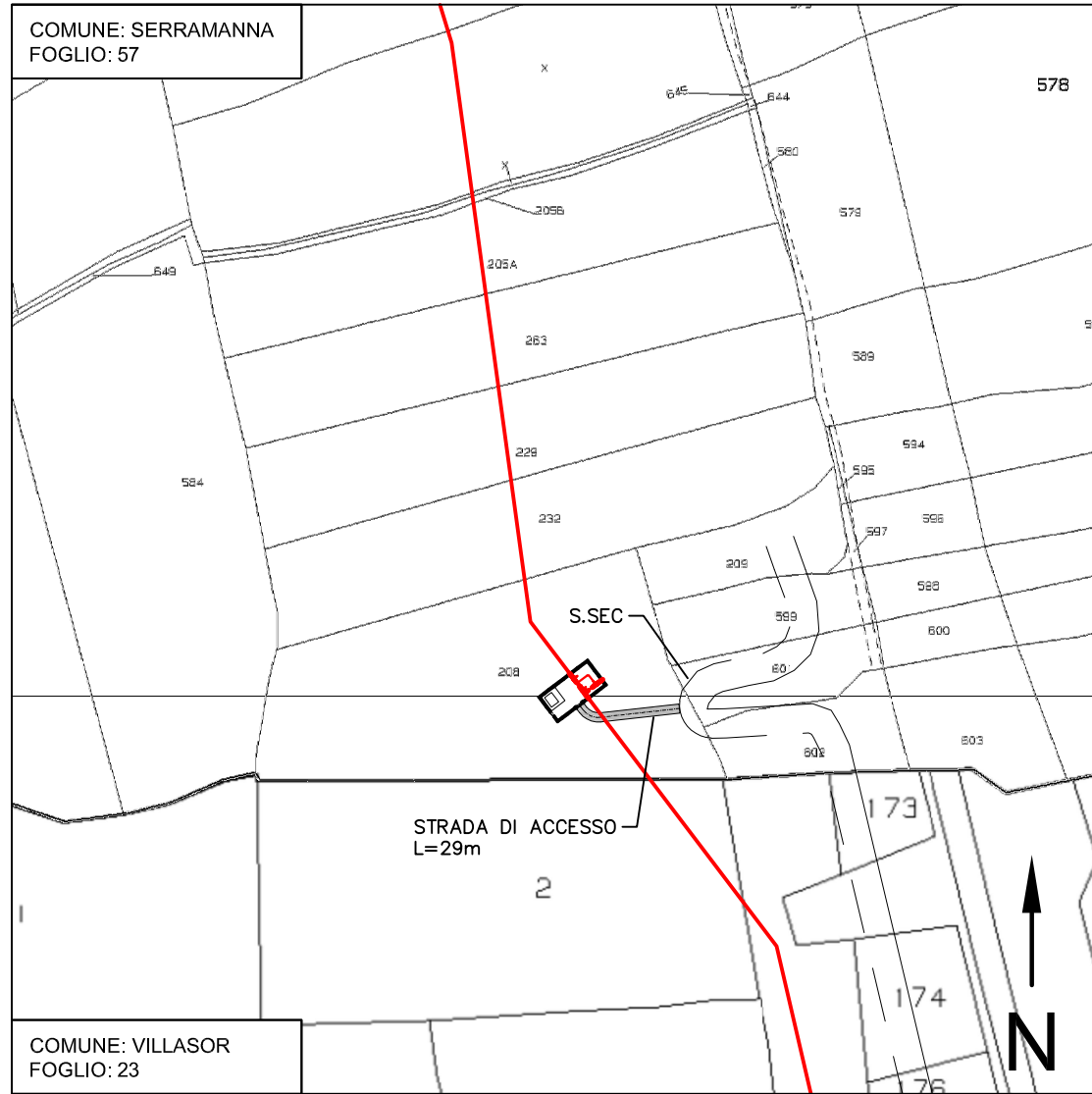
STRALCIO CATASTALE 1:2000
