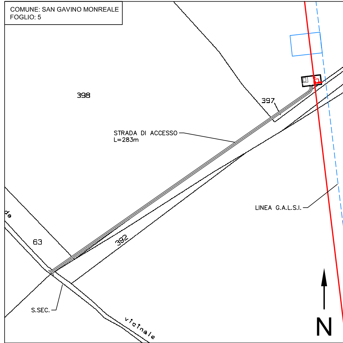
STRALCIO CATASTALE 1:2000
