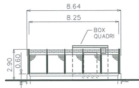
PROSPETTO - B -
