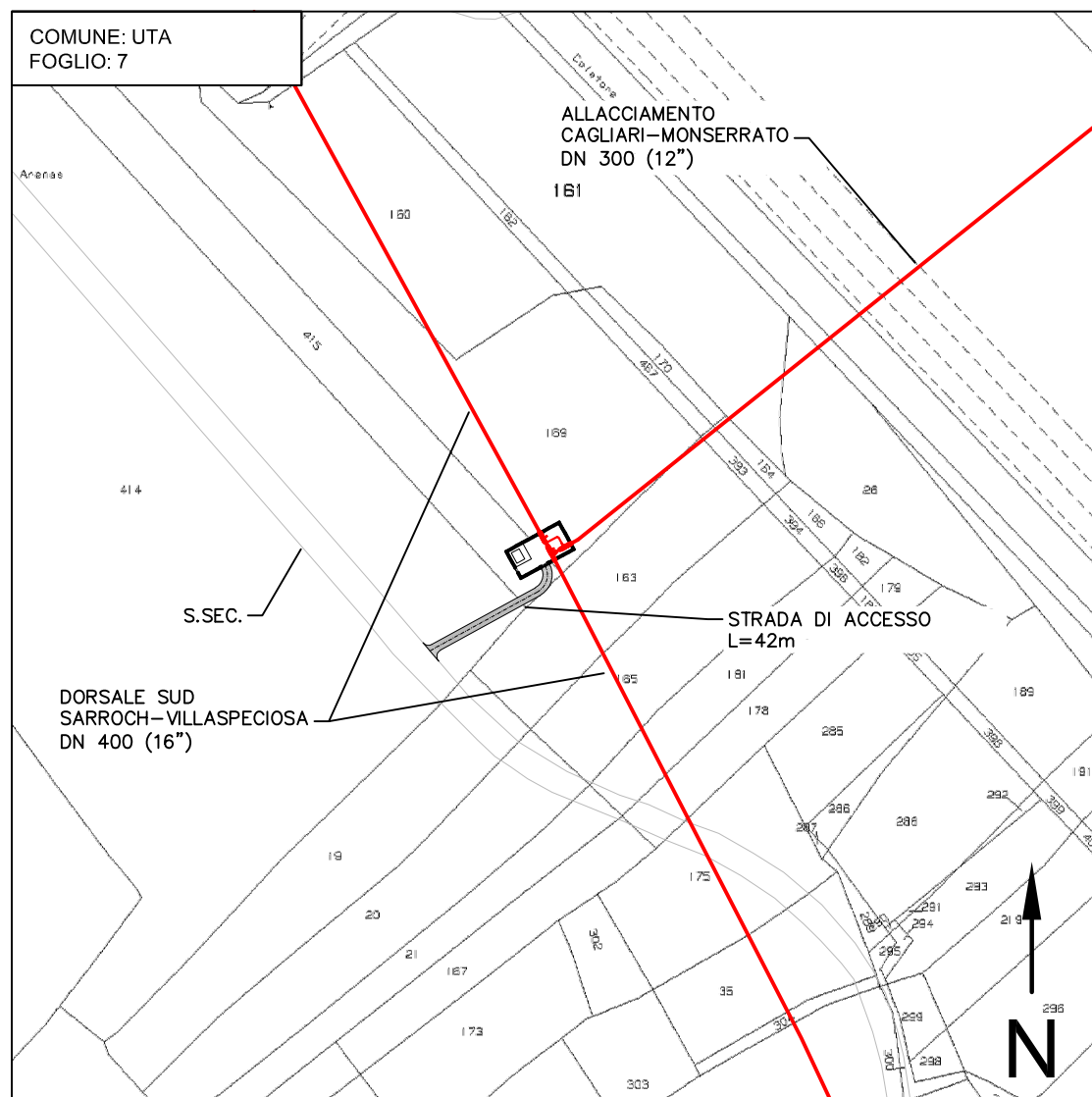
STRALCIO CATASTALE 1:2000
