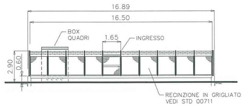
PROSPETTO - A -
