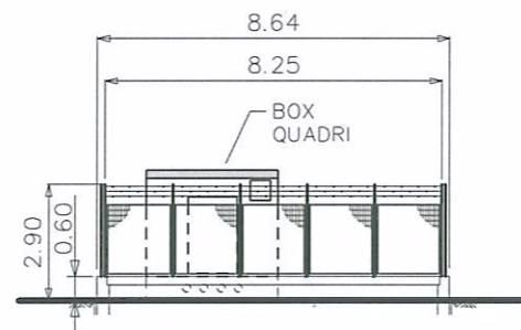
PROSPETTO - B -
