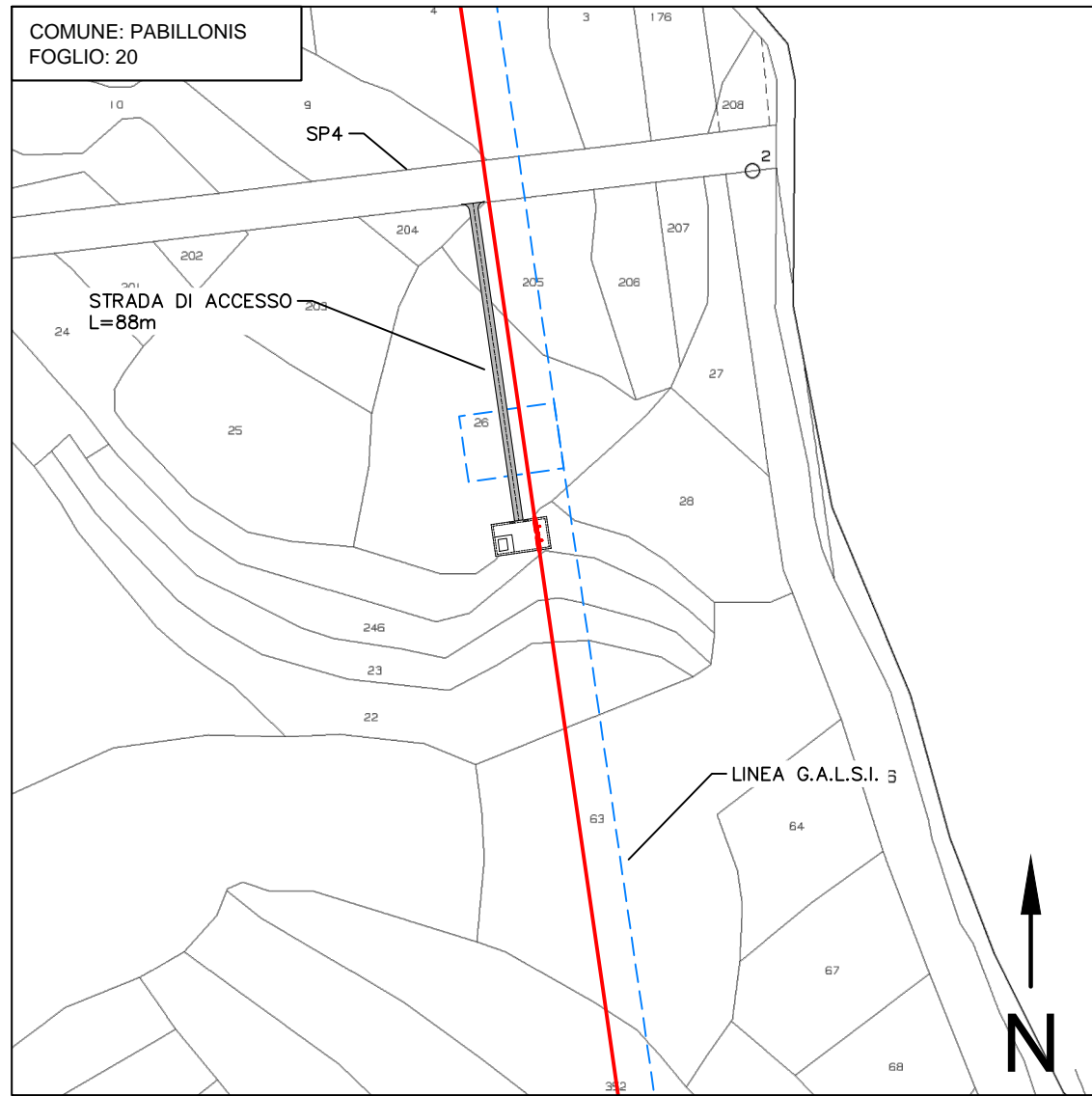
STRALCIO CATASTALE 1:2000
