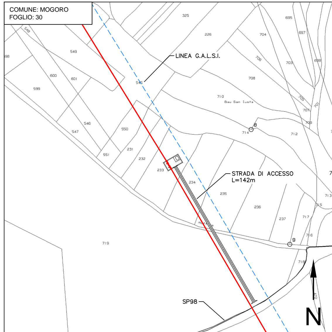
STRALCIO CATASTALE 1:2000
