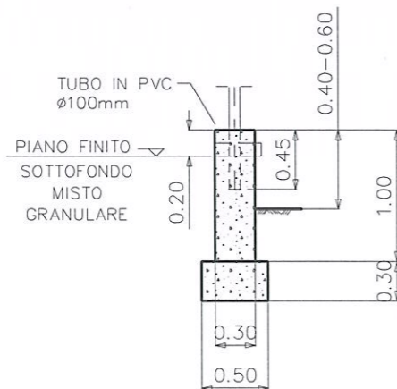
SEZIONE A-A Scala 1:50
