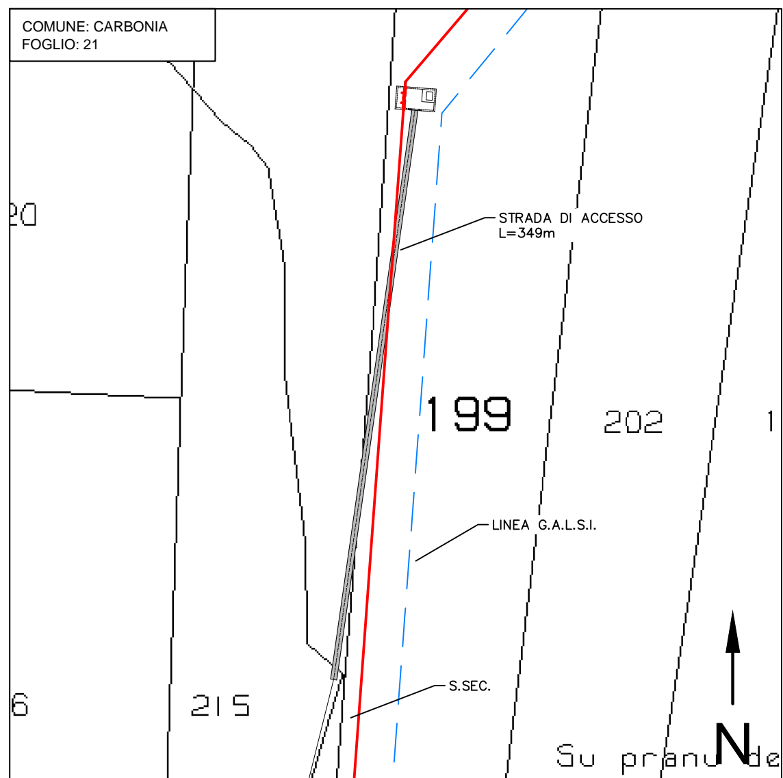
STRALCIO CATASTALE 1:2000
