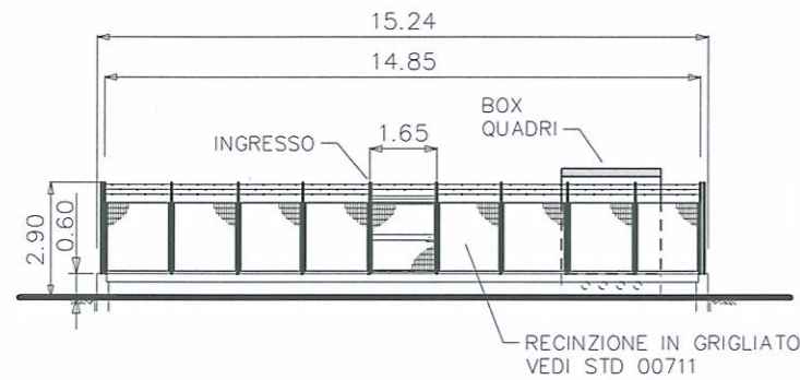
PROSPETTO - A -
