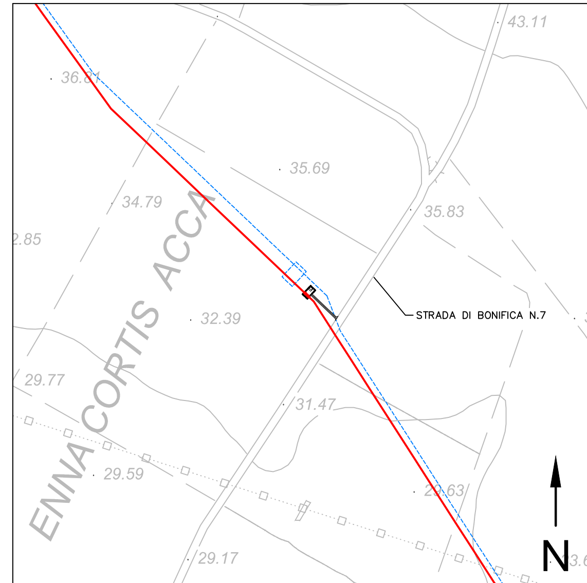
STRALCIO CTR 1:5000
