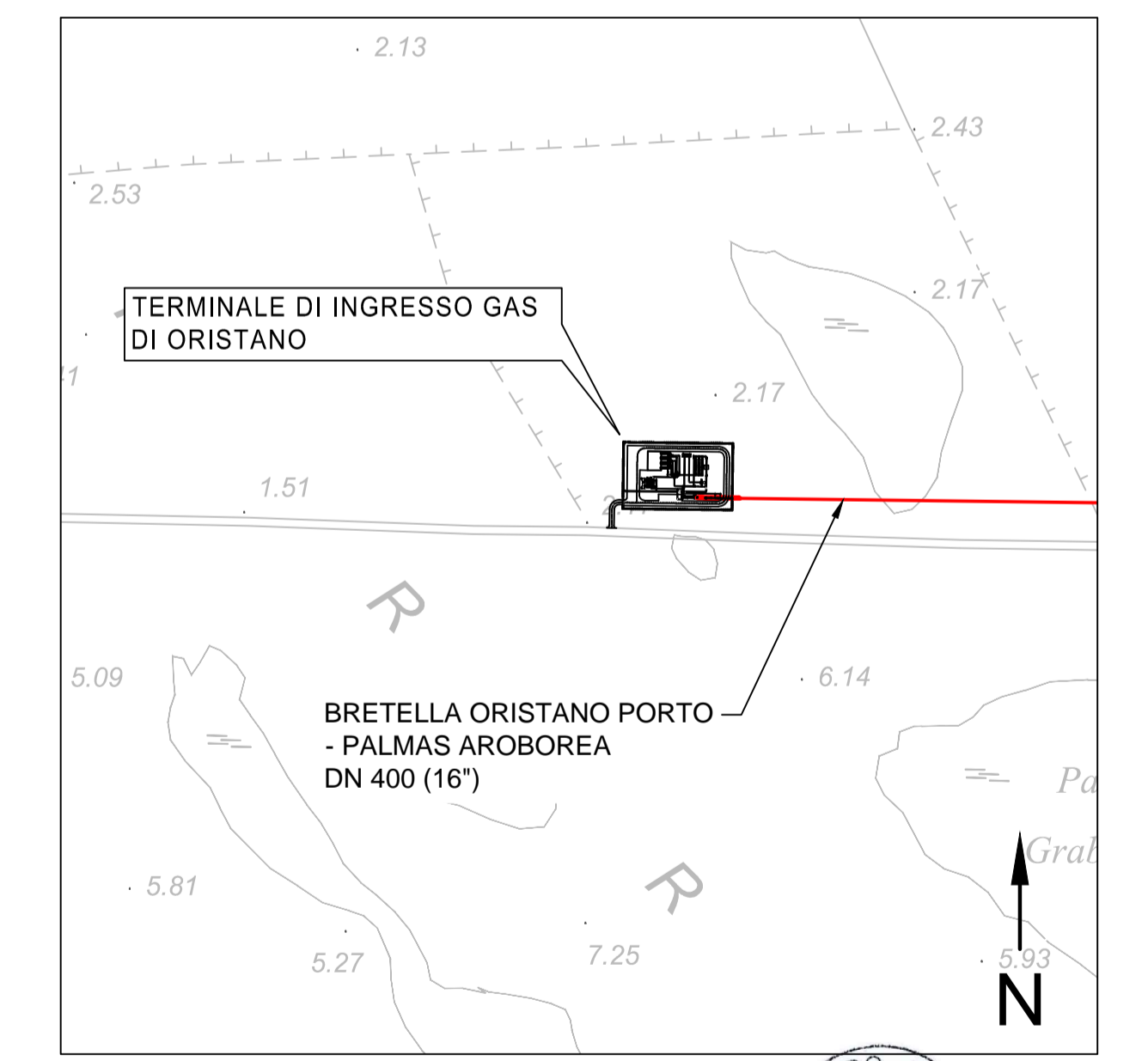
STRALCIO CTR 1:5000
