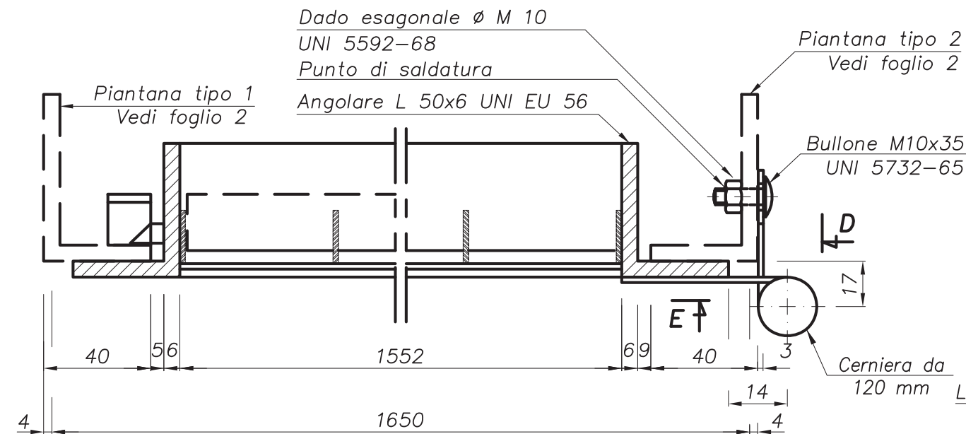
SEZIONE "A-A"
