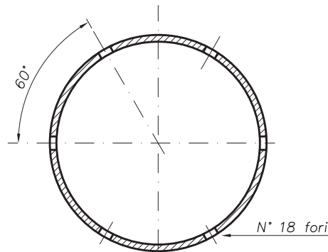
PARTICOLARE TESTATA
