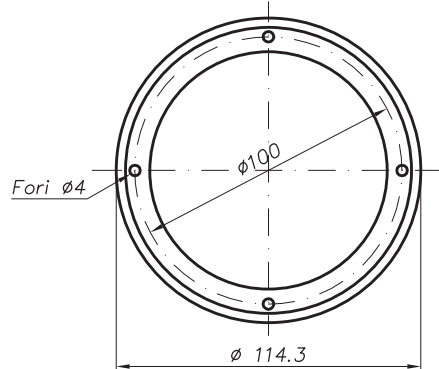
GHIERA
