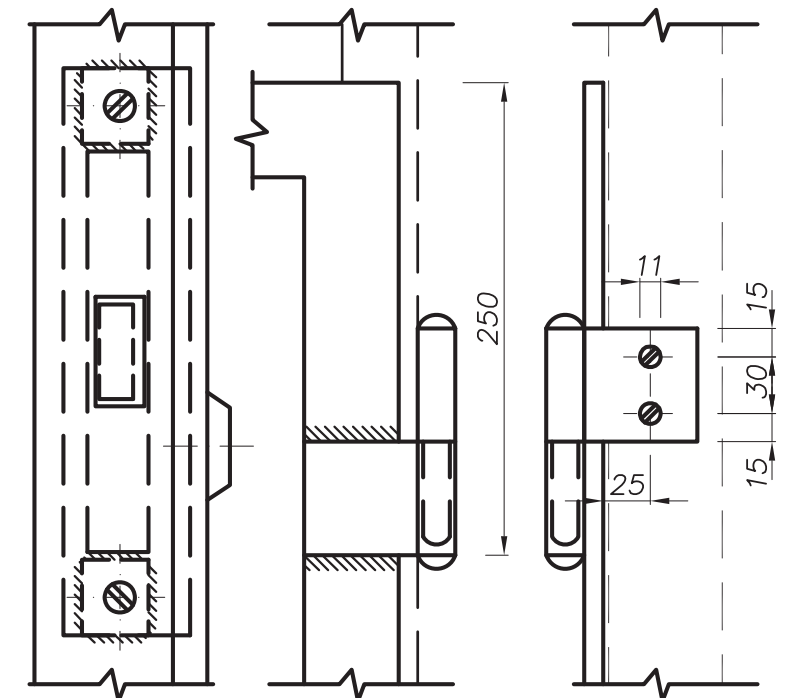
PARTICOLARE CERNIERA SUPERIORE: VISTA DA E VISTA DA D
