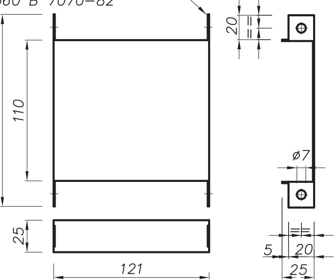
PARTICOLARE LAMIERA TIPO "A" PROTEZIONE SERRATURA
