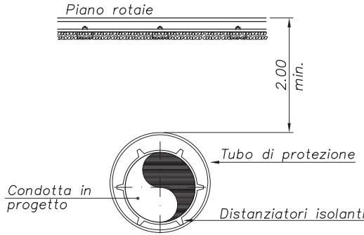
SEZIONE "A-A"
