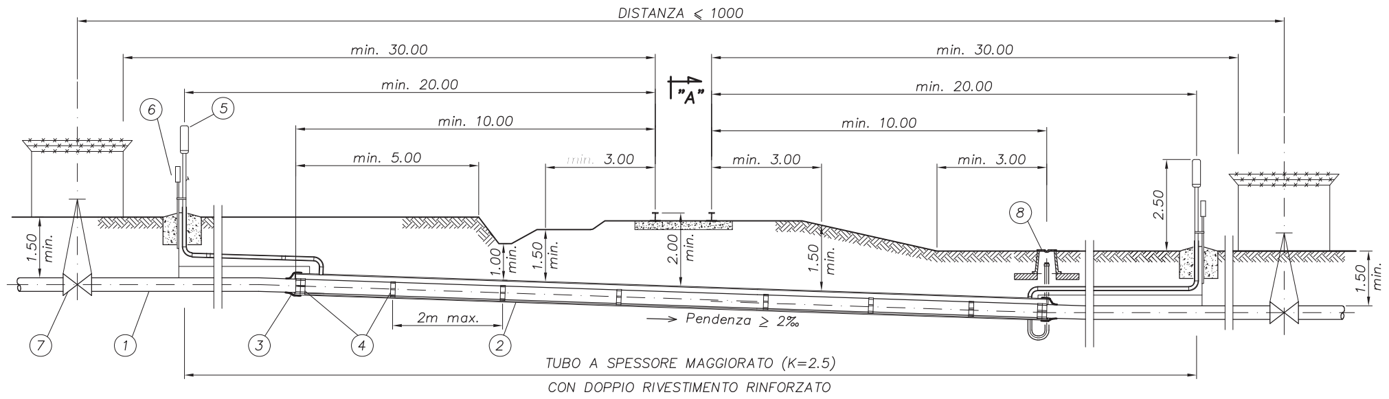
SEZIONE LONGITUDINALE
