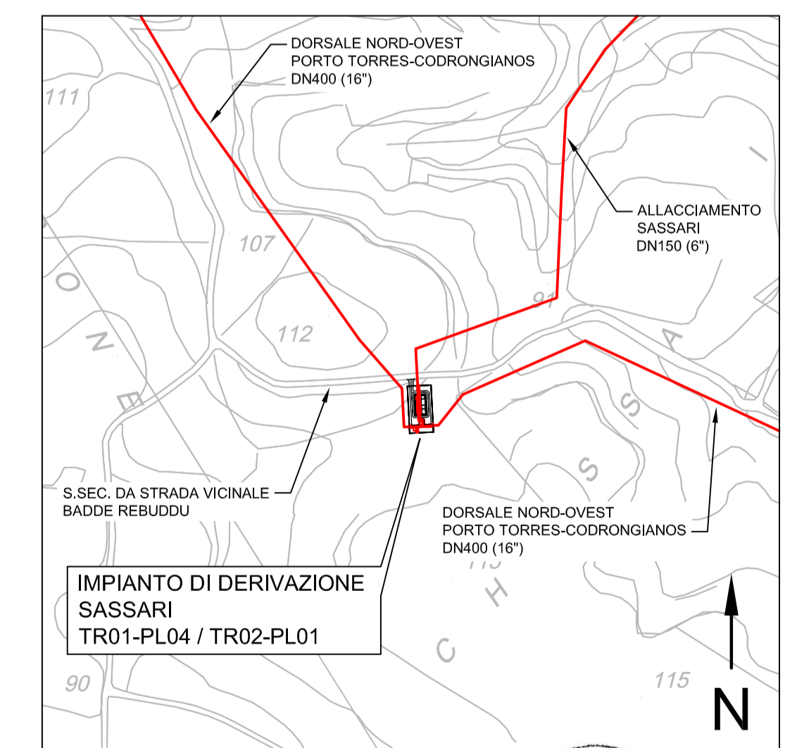
STRALCIO CTR 1:5000
