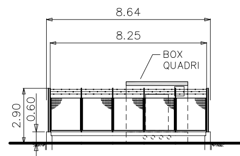
PROSPETTO - B -
