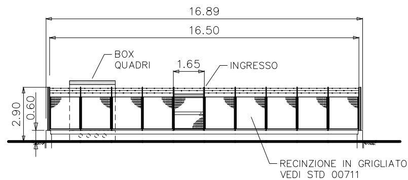
PROSPETTO - A -
