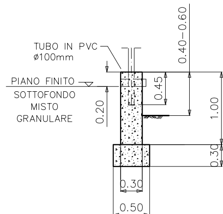
SEZIONE A-A Scala 1:50
