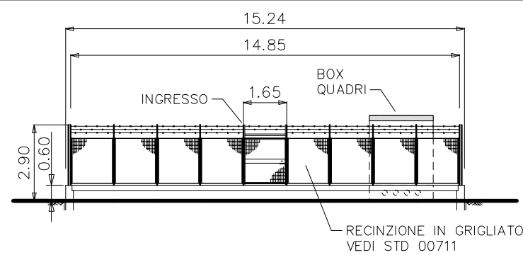
PROSPETTO - A -
