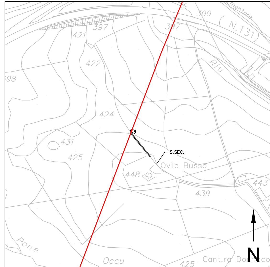
STRALCIO CTR 1:5000
