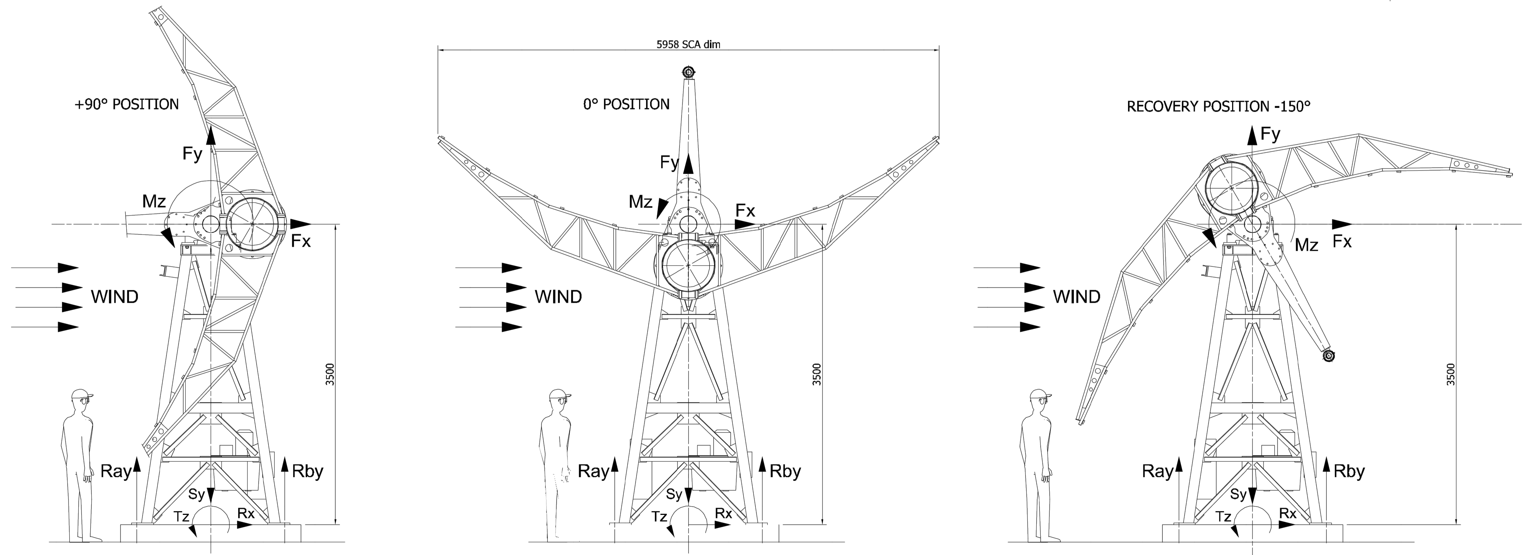
PARTICOLARI COSTRUTTIVI CAMPO SOLARE
