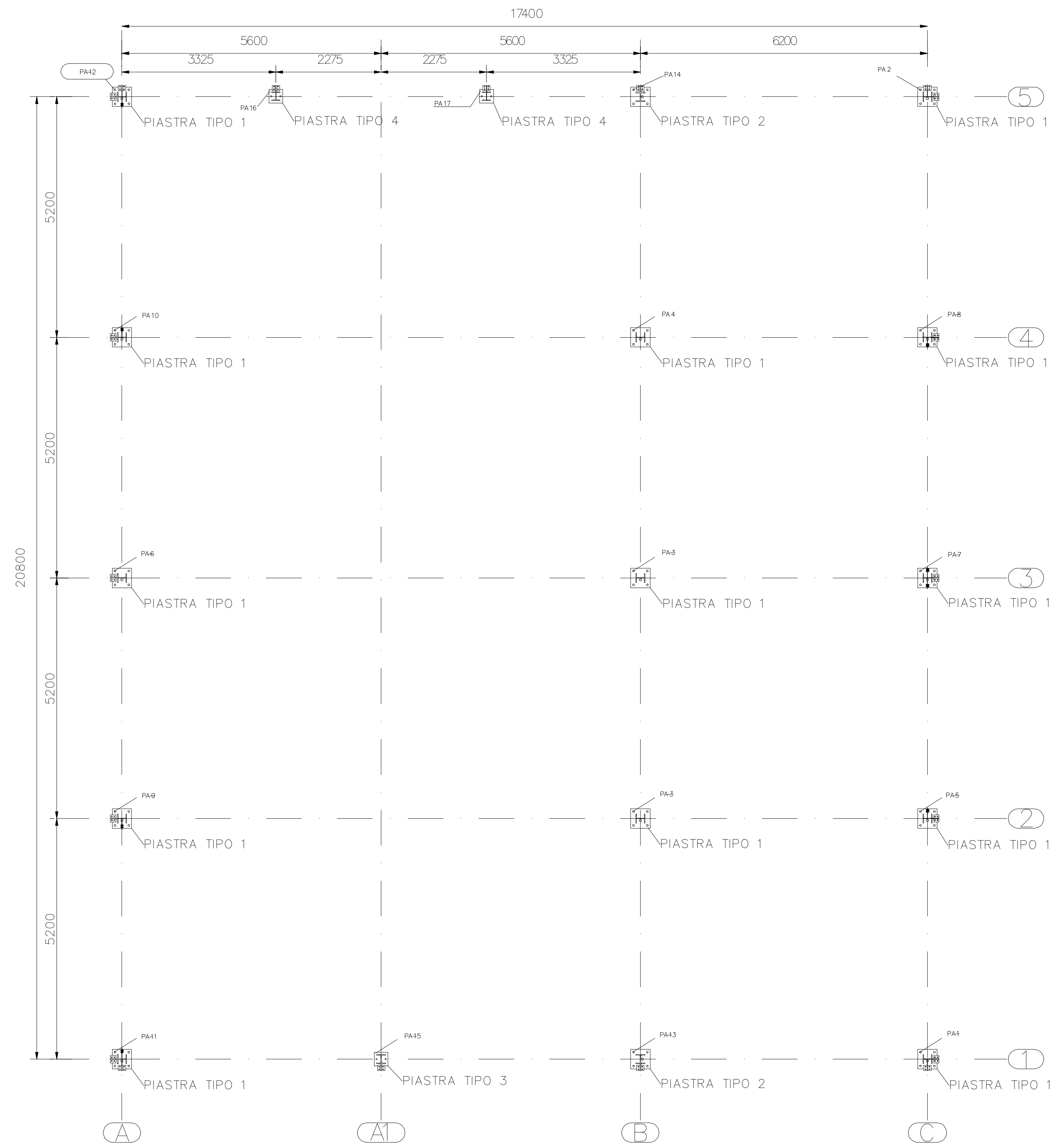
PIANTA FONDAZIONI SC=1:60
