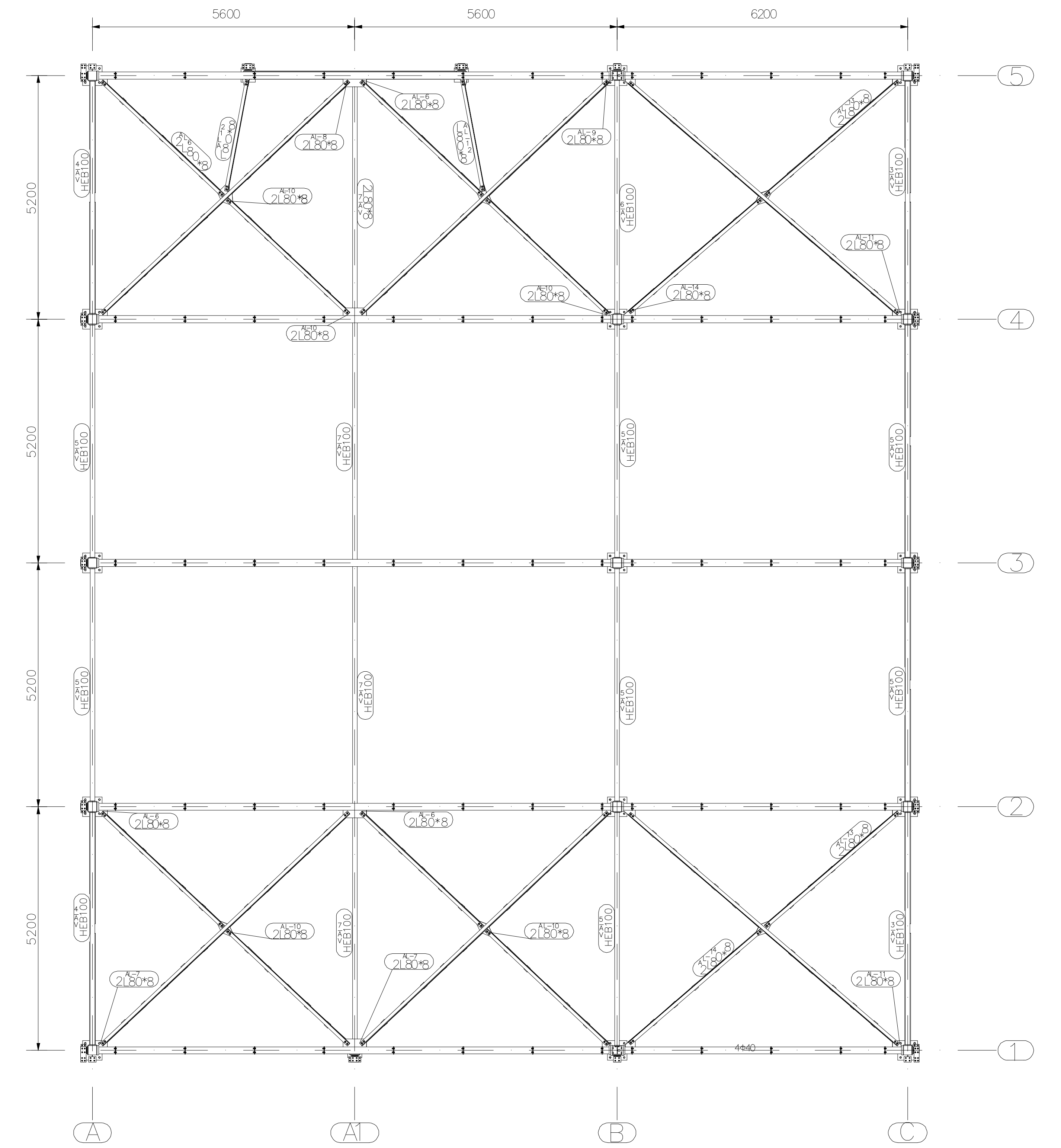
PIANTA COPERTURA SC=1:60
