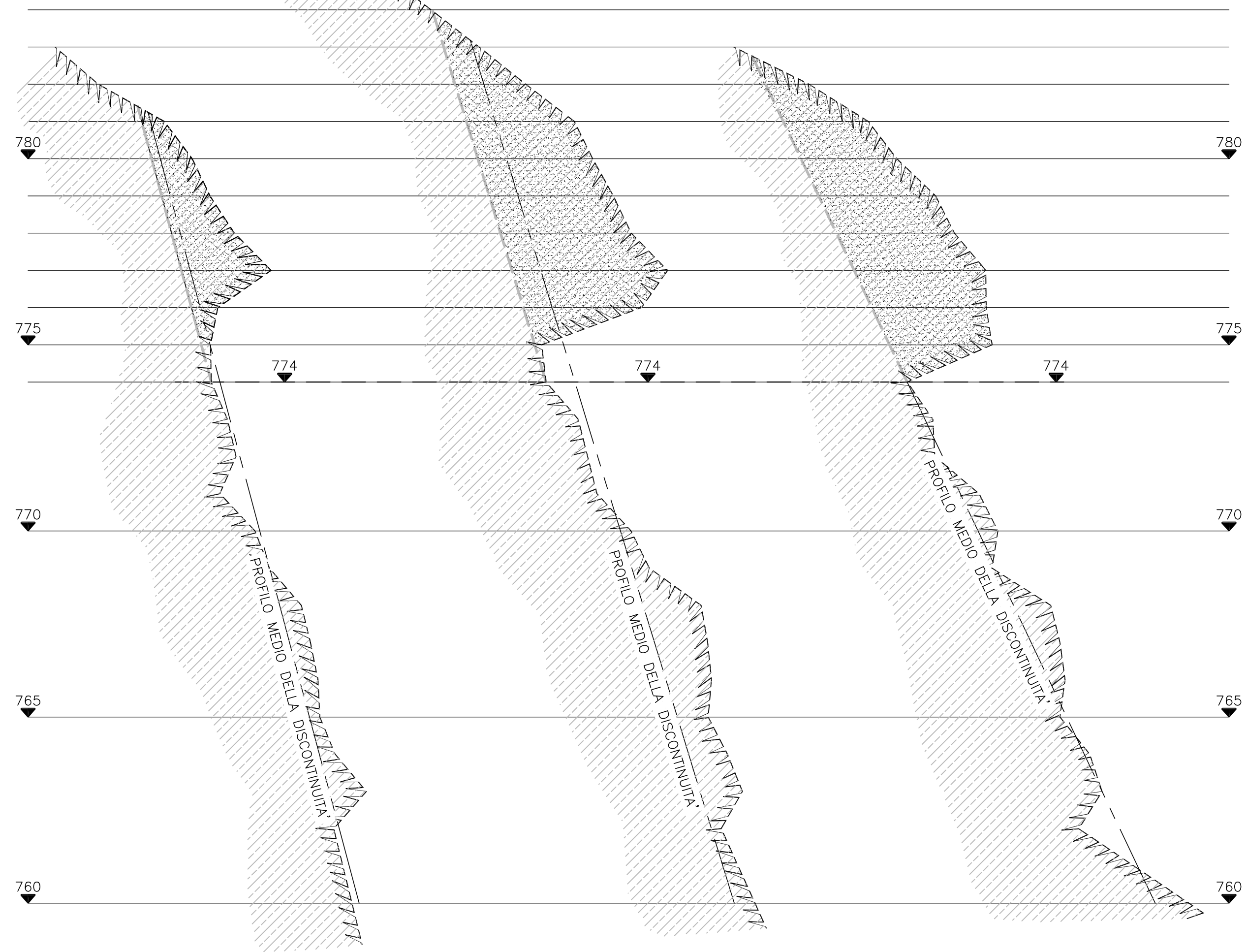
SEZIONE 1-1
