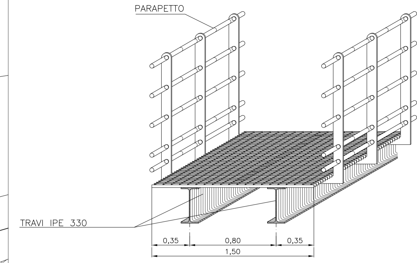
SEZIONE A-A SCALA 1:20
