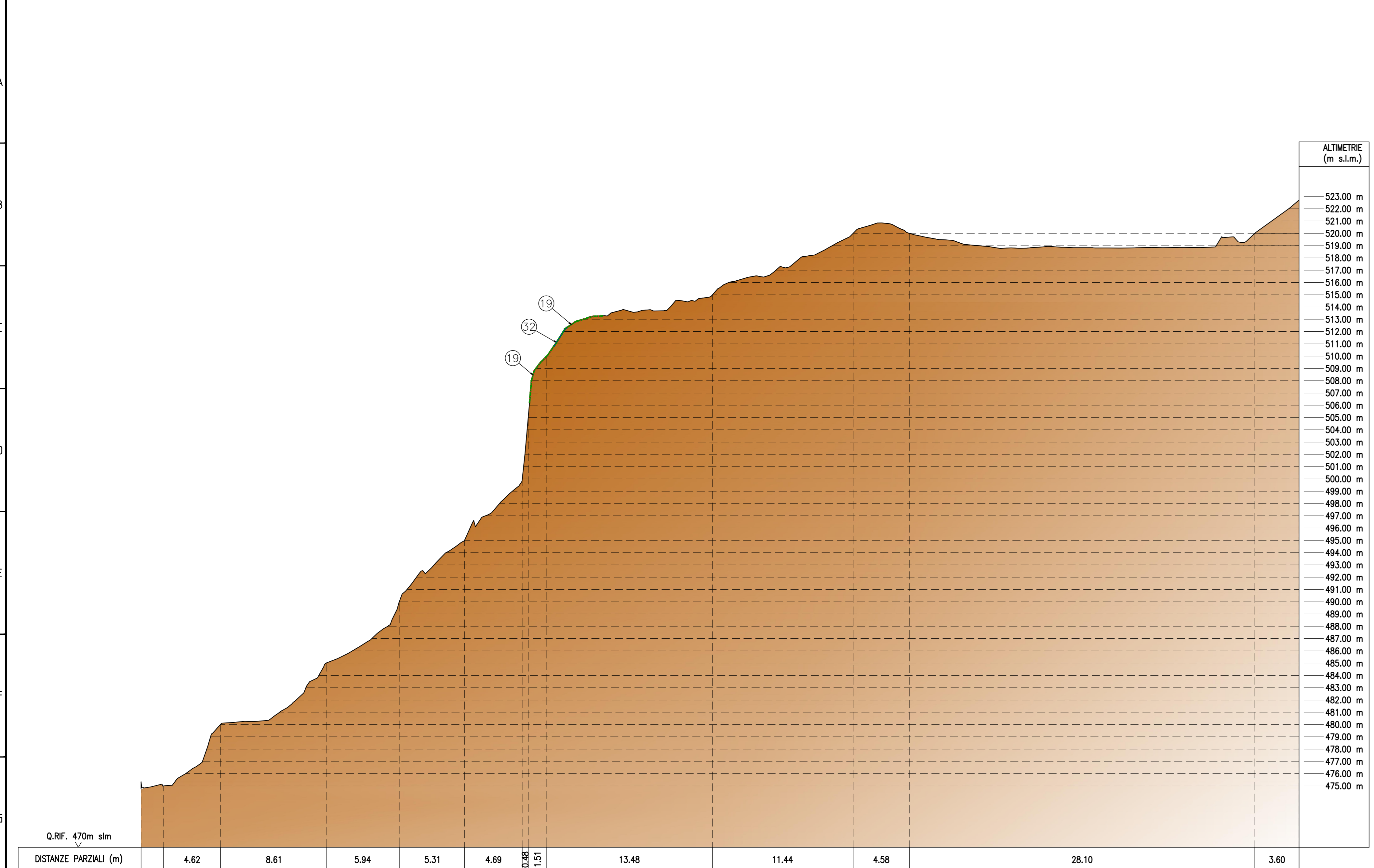
SEZIONE 1 SCALA 1:200
