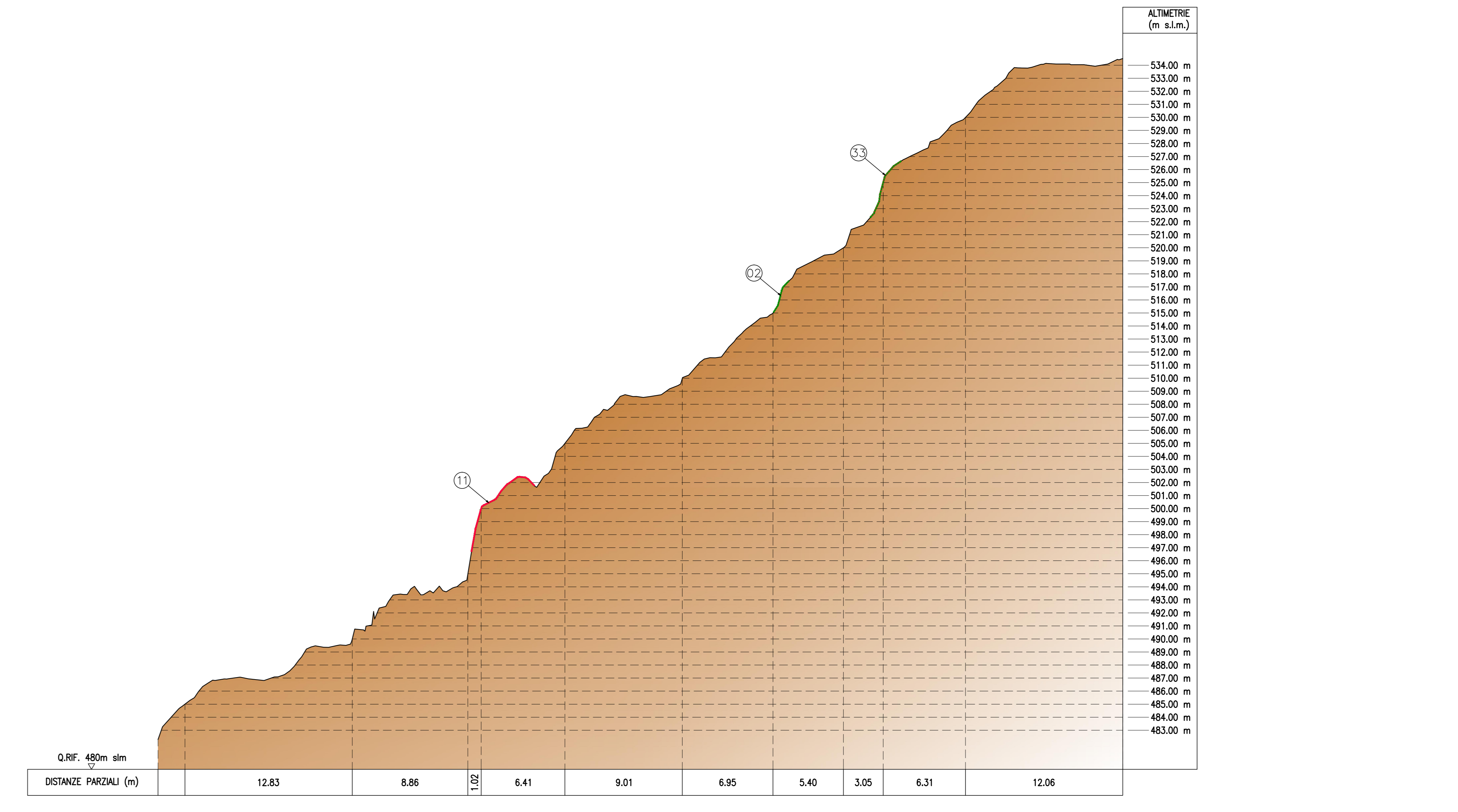
SEZIONE 2 SCALA 1:200
