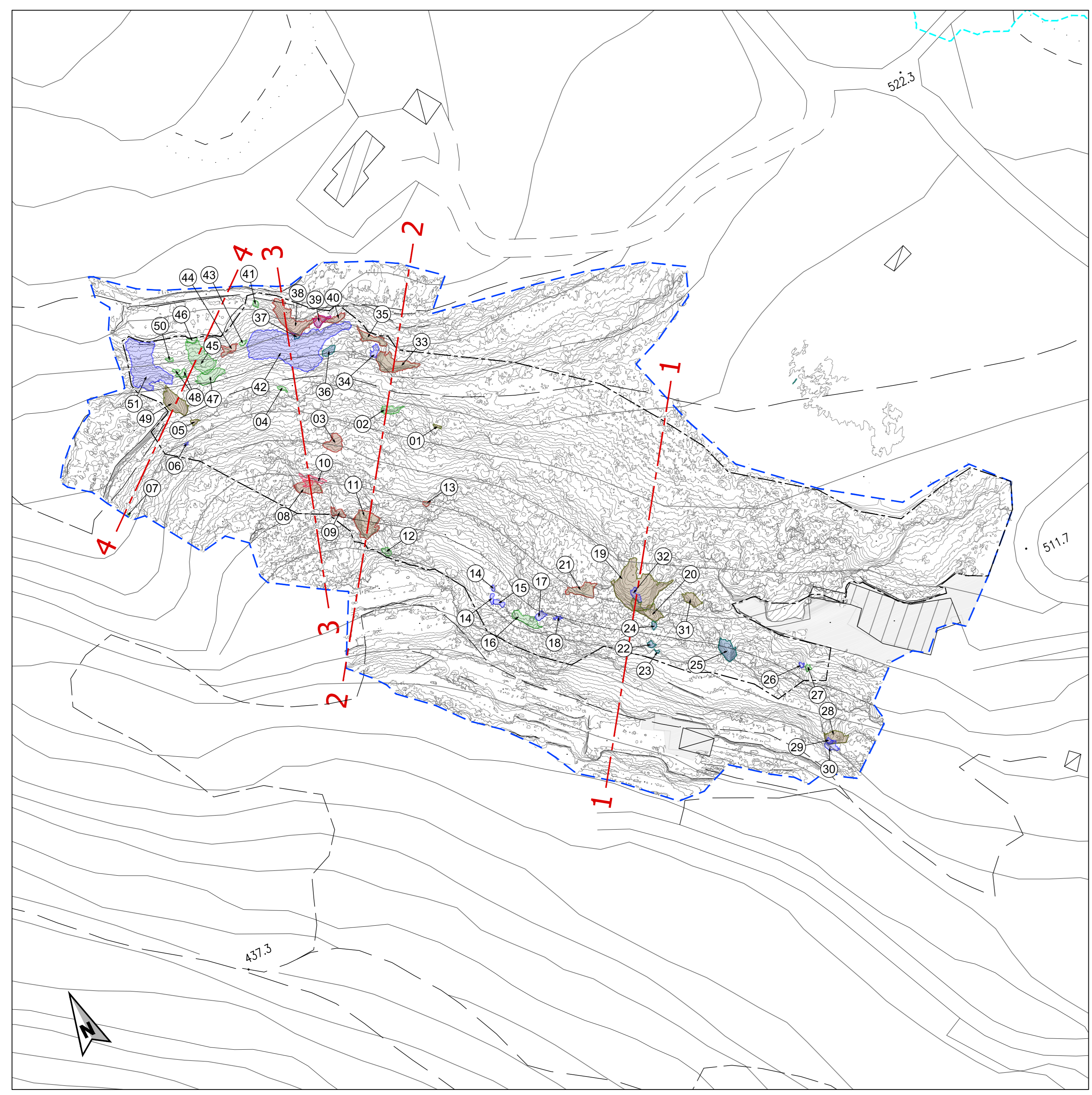
STRALCIO PLANIMETRICO SCALA 1:500
