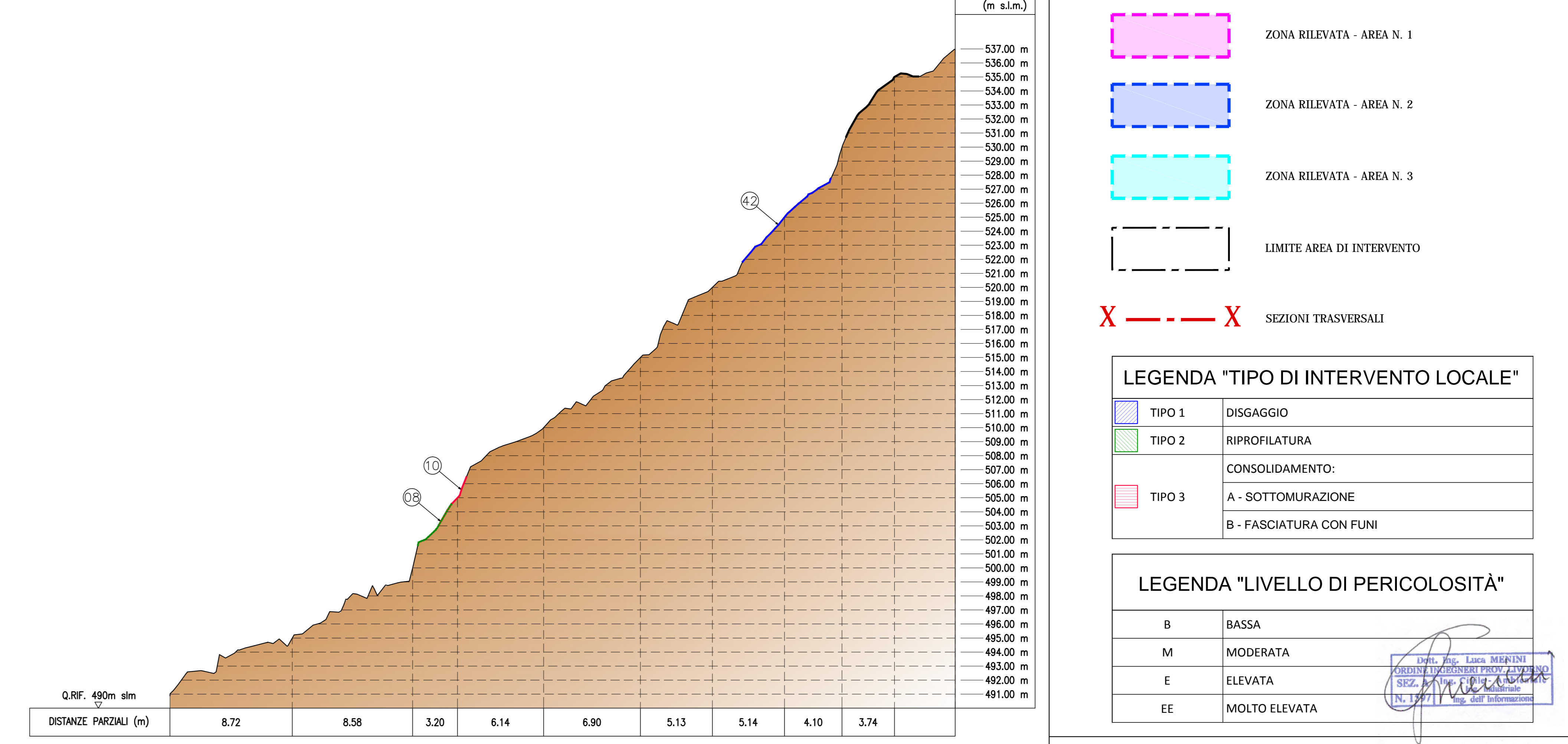
SEZIONE 4 SCALA 1:200
