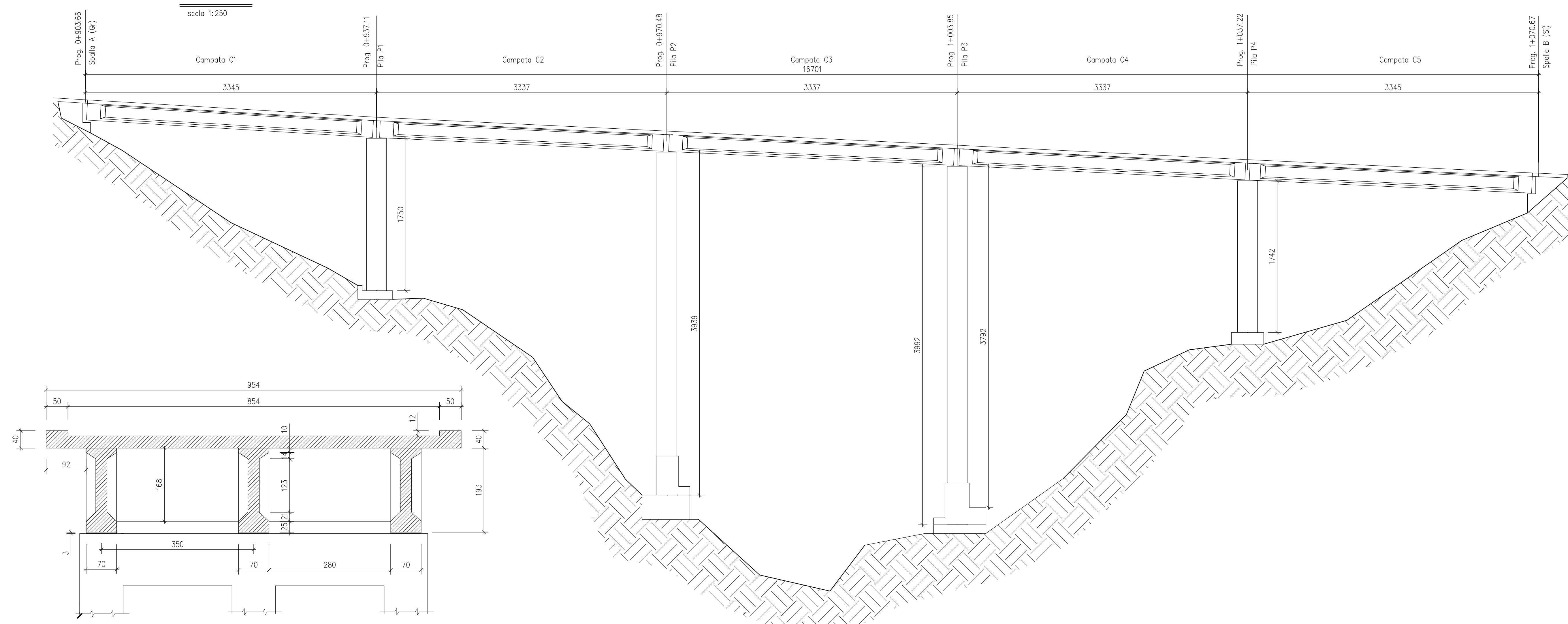
PROSPETTO
