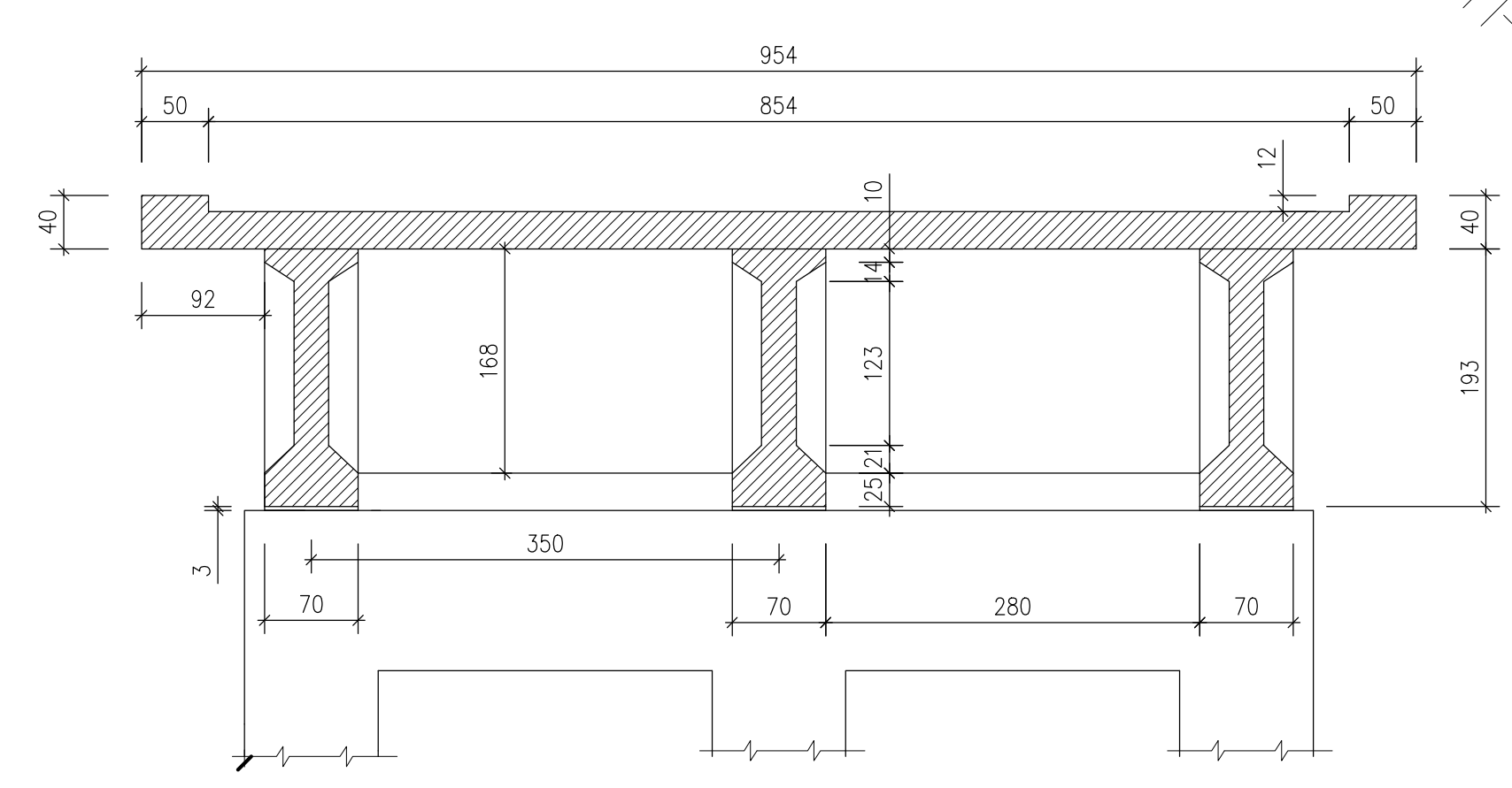
SEZIONE TIPO IN RETTIFILLO
