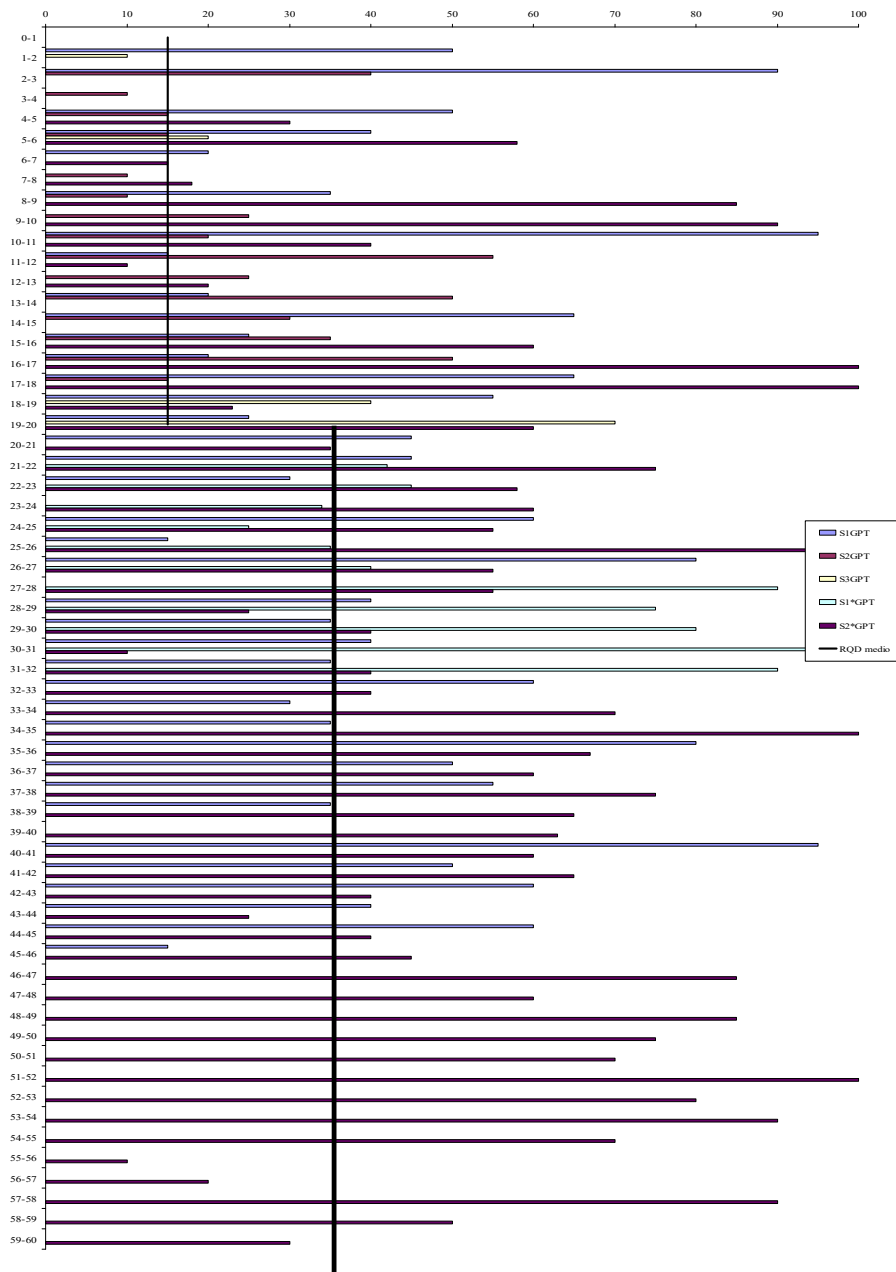
Figura 6: RQD rilevato nei sondaggi eseguiti in corrispondenza della galleria Poggio Tondo.
