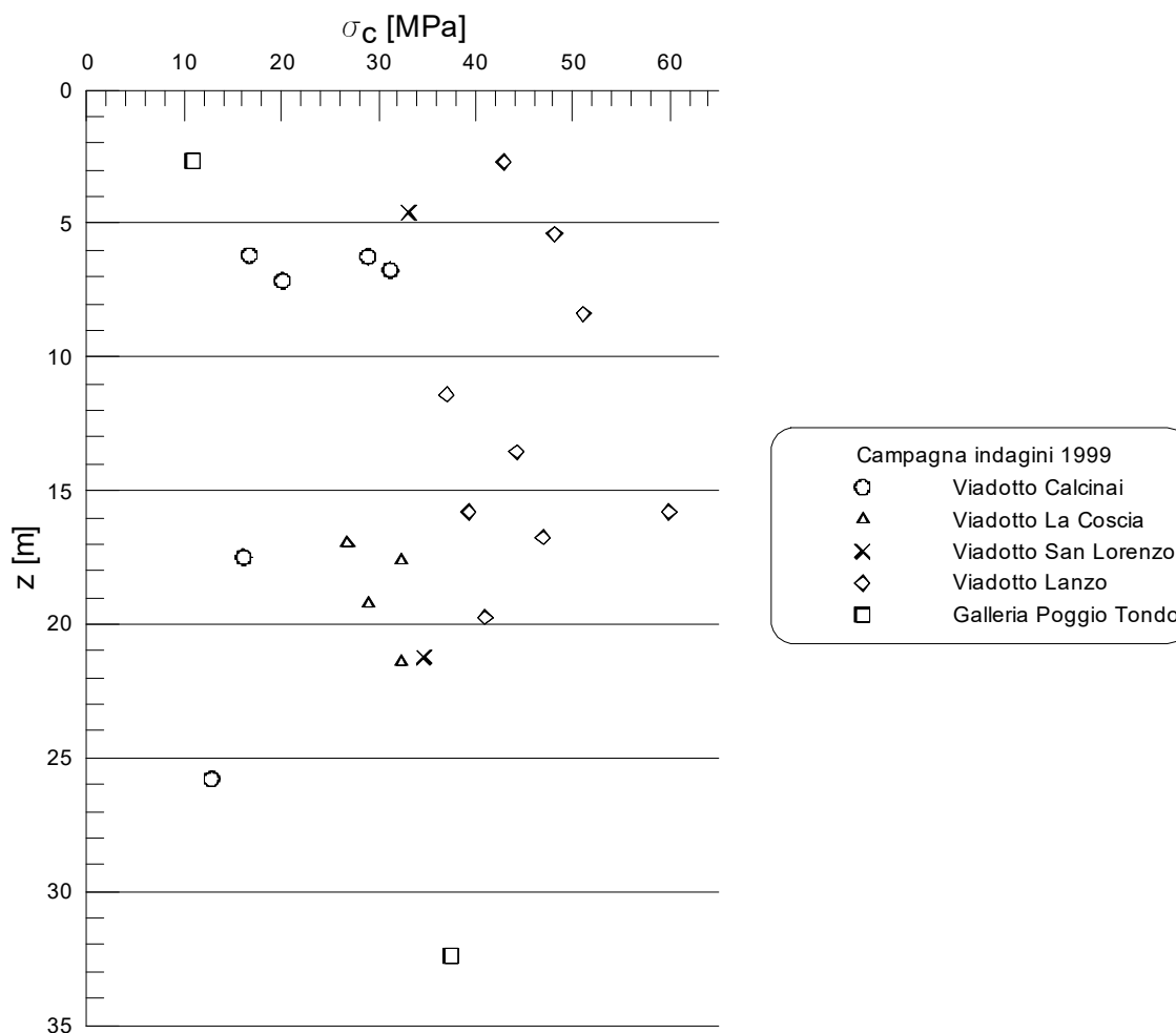
Figura 5: Resistenza a compressione uniassiale.
