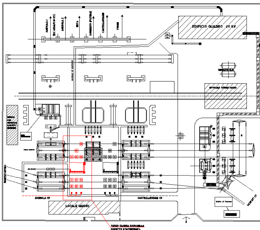
Figura 2 – Stralchio Planimetria generale Doc. C-ENEL-004D
