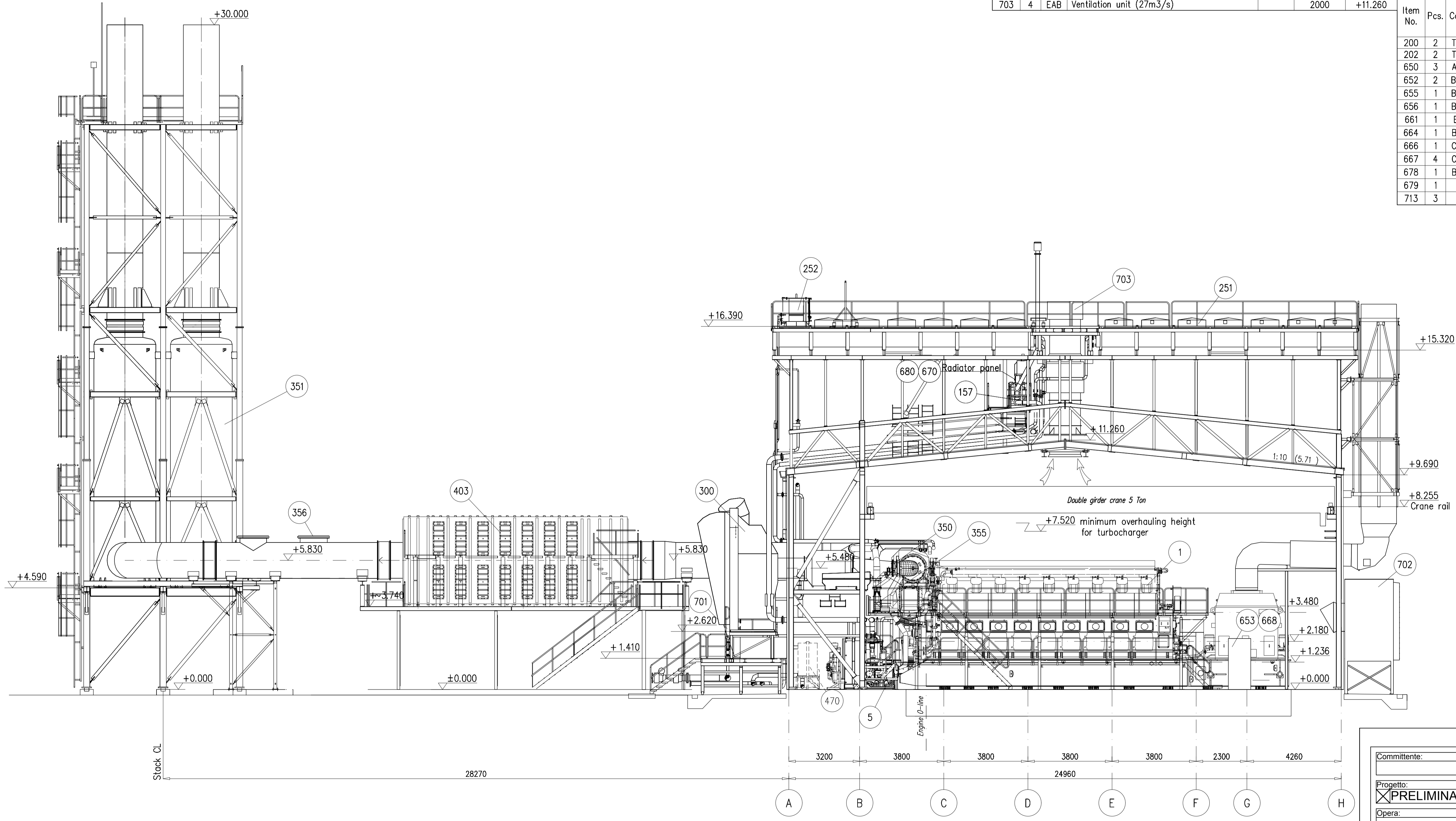
SECTION A-A
