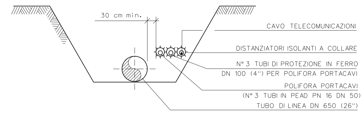
SEZIONE H-H
