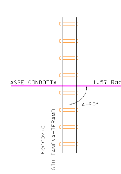
SEZIONE W-W
