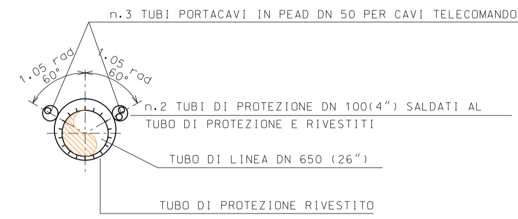
SEZIONE W-W
