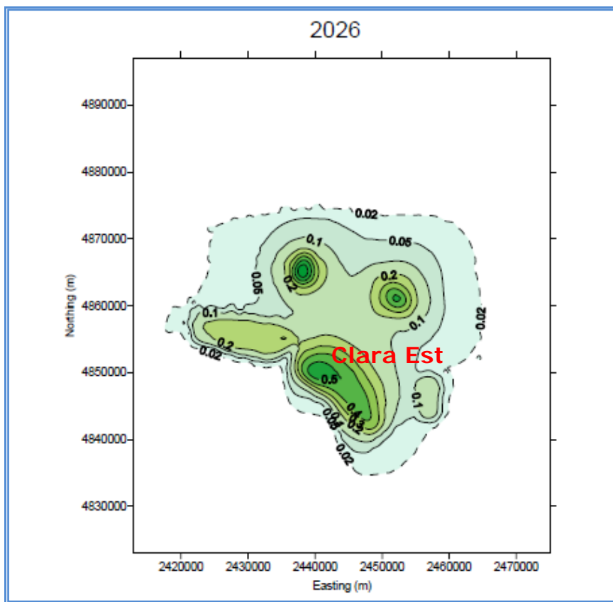
Figura 6 - Modello geomeccanico (settembre 2013): curve d'isosubsidenza (scenario di riferimento Cm_Med). Subs. max. su Clara Est: 56 cm @ 2026
