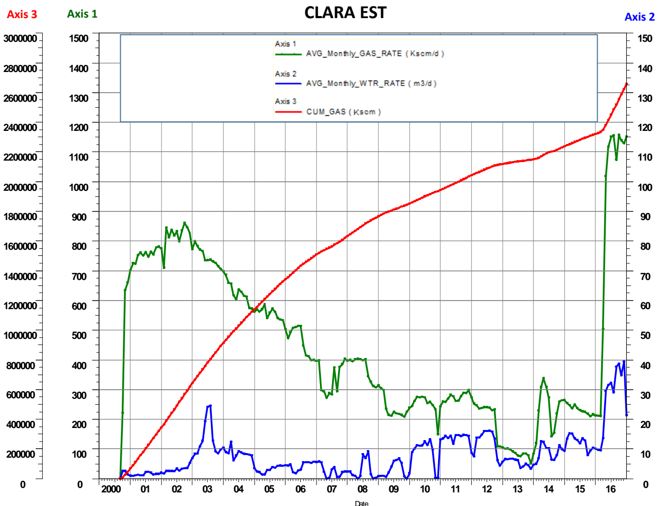
Figura 4- Campo di Clara Est-NW: grafico di produzione storica
