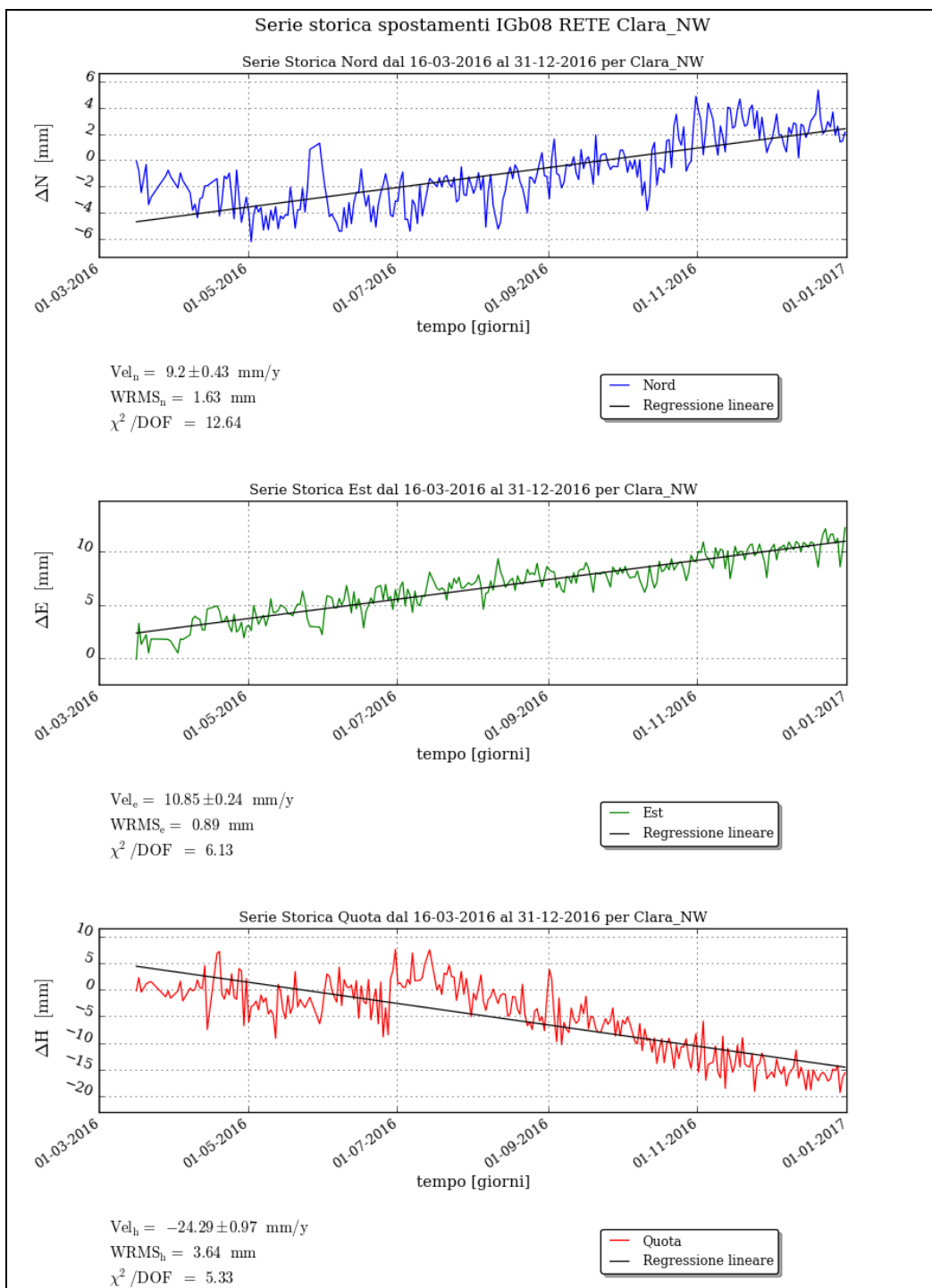
Figura 10 – Campo di Clara Est: serie storiche di misure plano-altimetriche registrate dal CGPS installato sulla p.ma Clara NW
