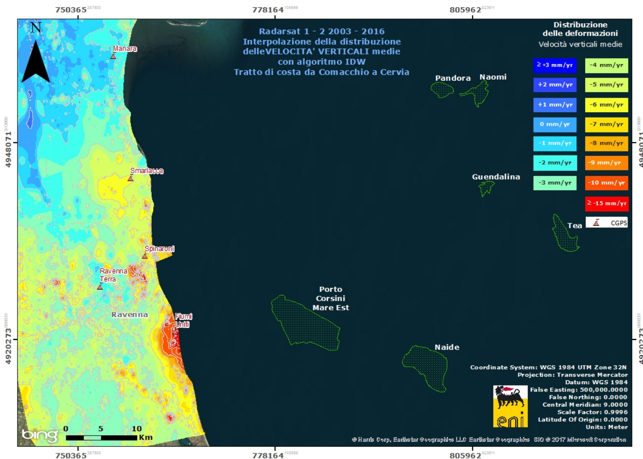
Fig. 2A - Interpolazione IDW (Inverse Distance Weighted) dei dati Radarsat 1 -2, per il periodo 2003 – 2016, con Tool ArcGis Spatial Analyst®. Tratto di costa da Comacchio a Cervia
