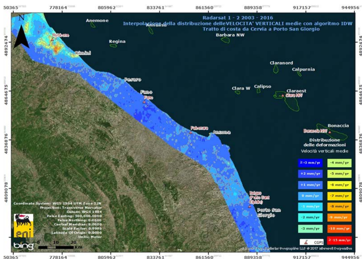
Fig. 4A - Interpolazione IDW (Inverse Distance Weighted) dei dati Radarsat 1 -2, per il periodo 2003 – 2016, con Tool ArcGis Spatial Analyst®. Tratto di costa da Cervia a Porto San Giorgio
