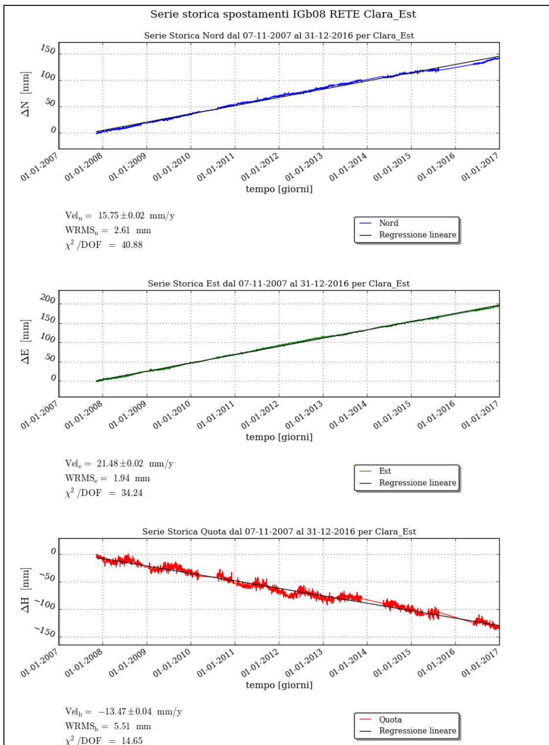
Figura 11 – Campo di Clara Est: serie storiche di misure plano-altimetriche registrate dal CGPS installato sulla p.ma Clara Est
