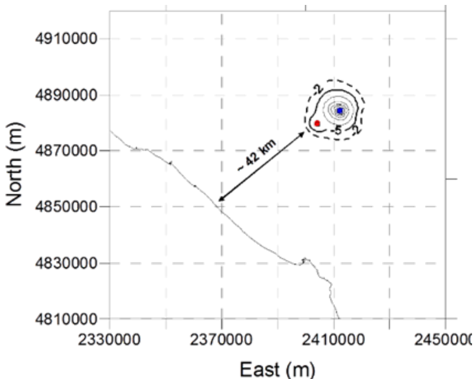
Figura 6 – Campo di Fauzia: curve d'isosubsidenza per lo scenario di riferimento a fine simulazione (2060). Max subs su Fauzia: 11 cm@2060
