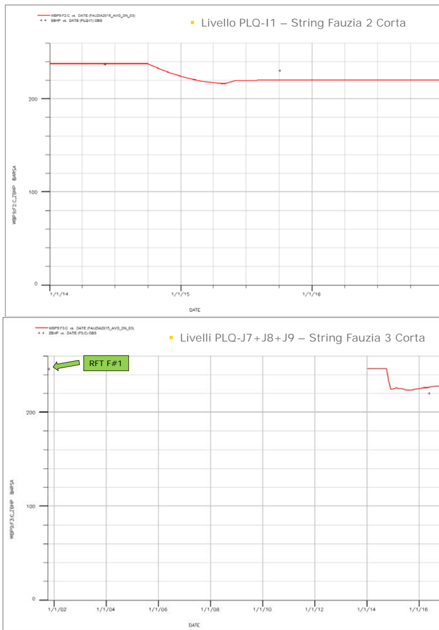
Figura 5 – Campo di Fauzia: dati di pressione (da RFT) vs. modello Eclipse 2015
