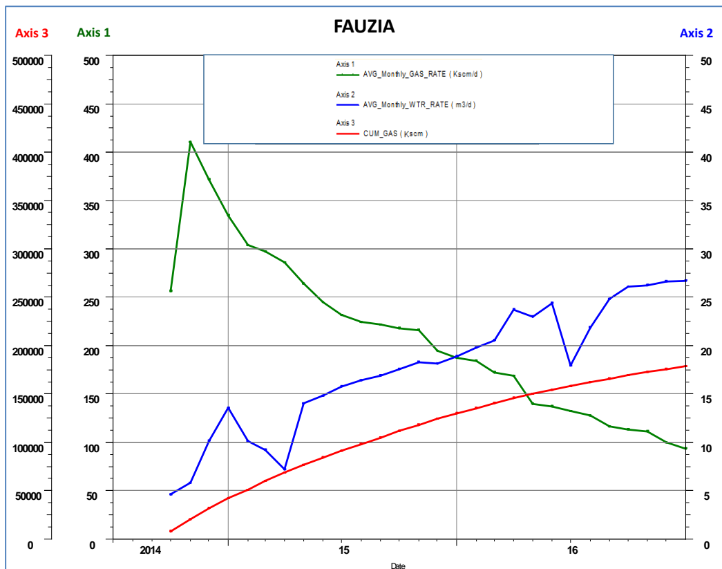
Figura 4 - Campo di Fauzia: grafico di produzione storica
