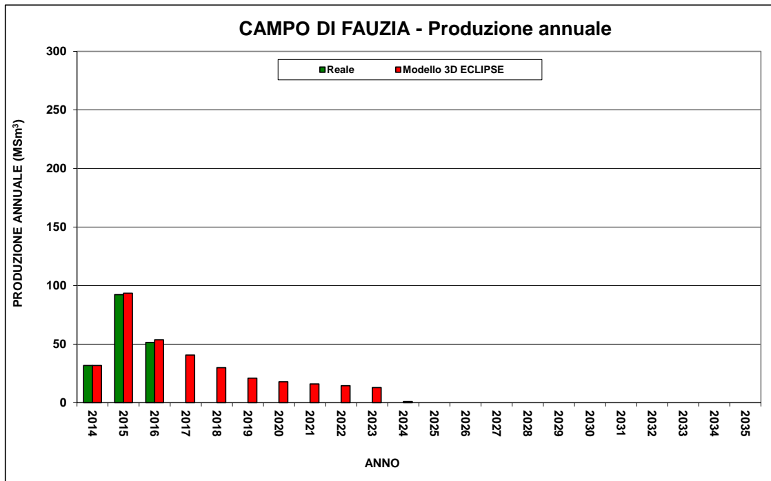
Figura 3 - Campo di Fauzia: tabelle e grafici di produzione vs. modello Eclipse (2015)
