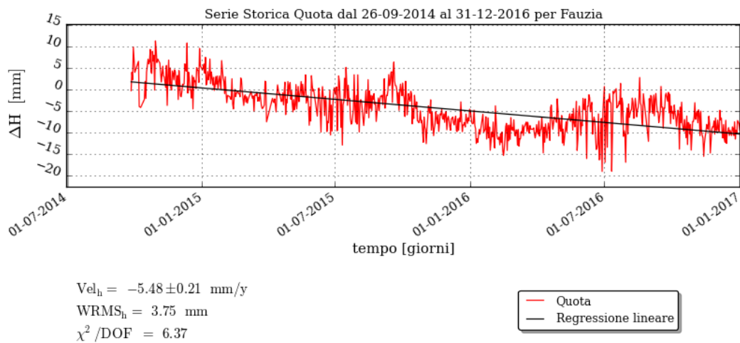
Figura 10 - Campo di Fauzia: serie storiche plano-altimetriche CGPS completa
