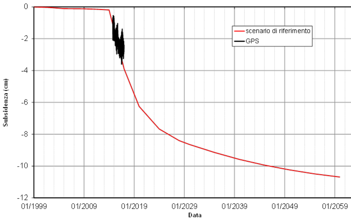
Figura 12 – Campo di Fauzia: andamento della subsidenza prevista da modello geomeccanico (dic. 2013 - scenario di riferimento) in corrispondenza della p.ma di produzione vs. le misure da CGPS aggiornate al dic. 2016
