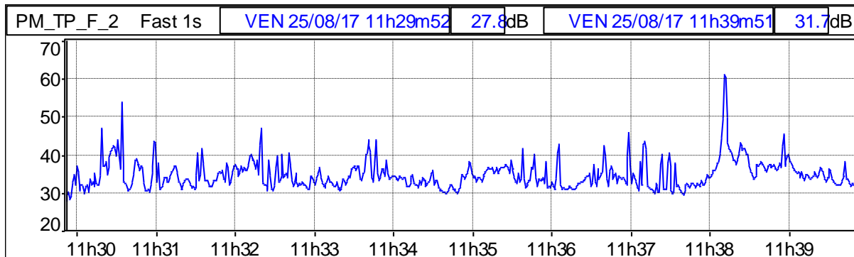
Grafico 133: Profilo temporale ponderato in curva "A" e costante di tempo "FAST"
