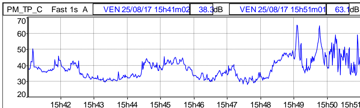
Grafico 89: Profilo temporale ponderato in curva "A" e costante di tempo "FAST"
