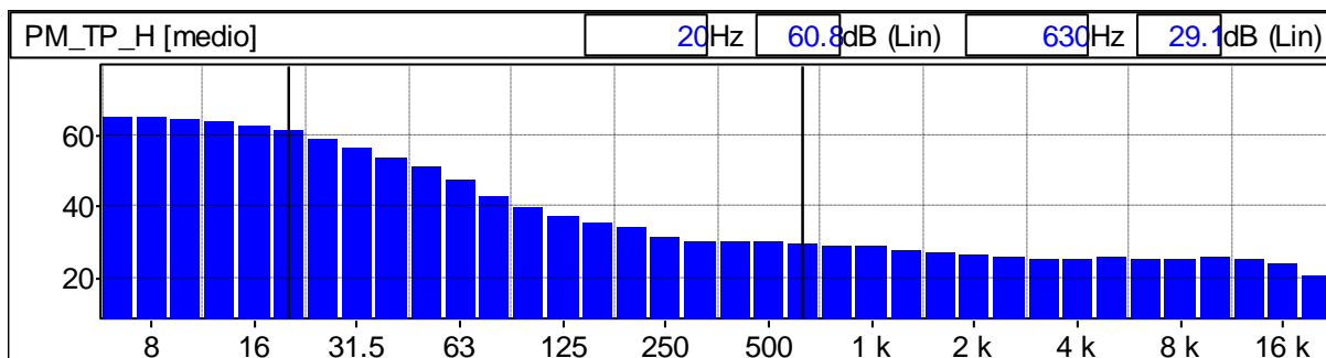
Grafico 150: Spettro del rumore rilevato 1/3 Ottava Leq Lineare
