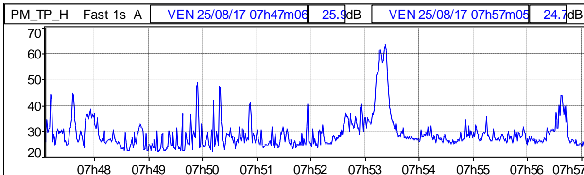
Grafico 145: Profilo temporale ponderato in curva "A" e costante di tempo "FAST"
