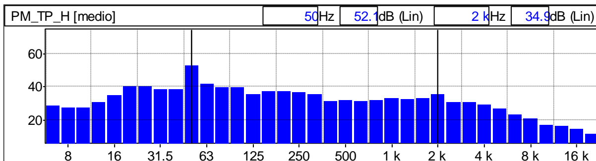
Grafico 146: Spettro del rumore rilevato 1/3 Ottava Leq Lineare
