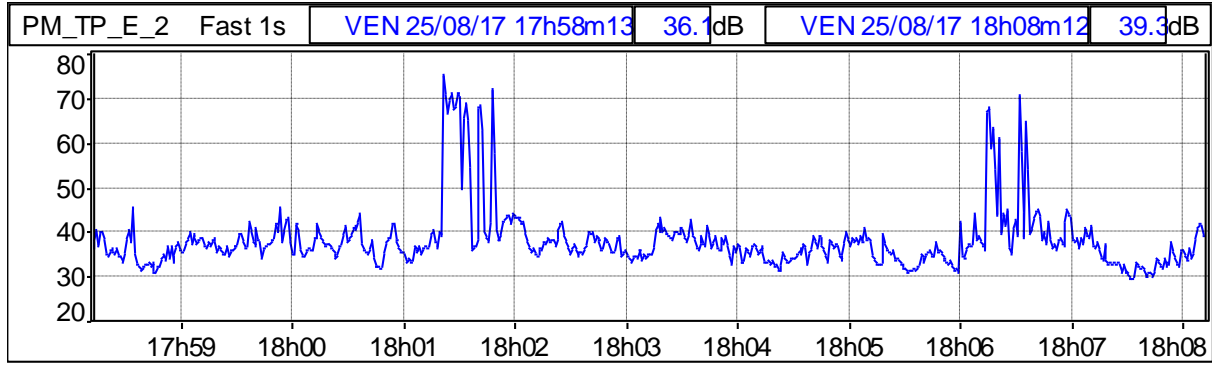
Grafico 125: Profilo temporale ponderato in curva "A" e costante di tempo "FAST"
