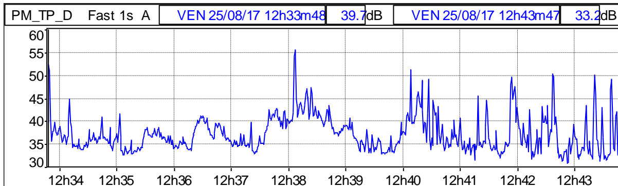
Grafico 101: Profilo temporale ponderato in curva "A" e costante di tempo "FAST"
