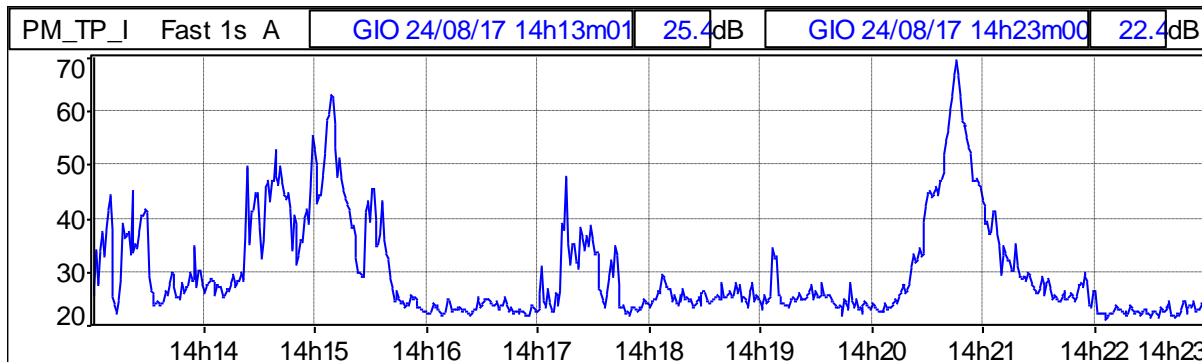
Grafico 169: Profilo temporale ponderato in curva "A" e costante di tempo "FAST"
