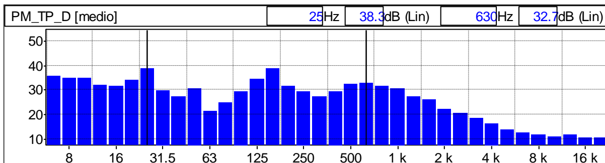
Grafico 110: Spettro del rumore rilevato 1/3 Ottava Leq Lineare
