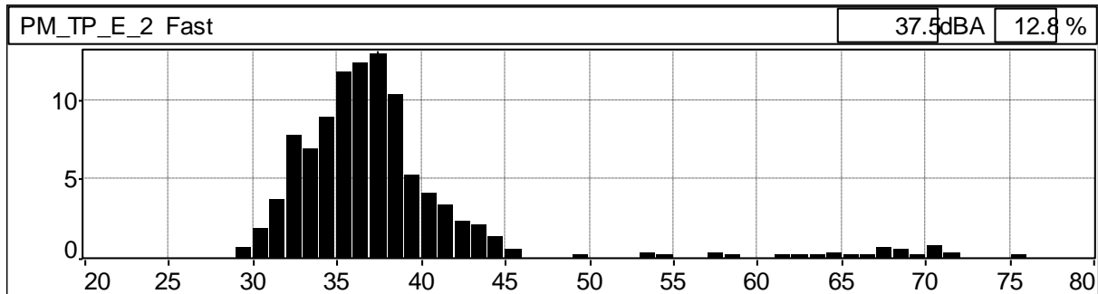
Grafico 128: Distribuzione cumulativa ponderata in curva "A" e costante di tempo "FAST"
