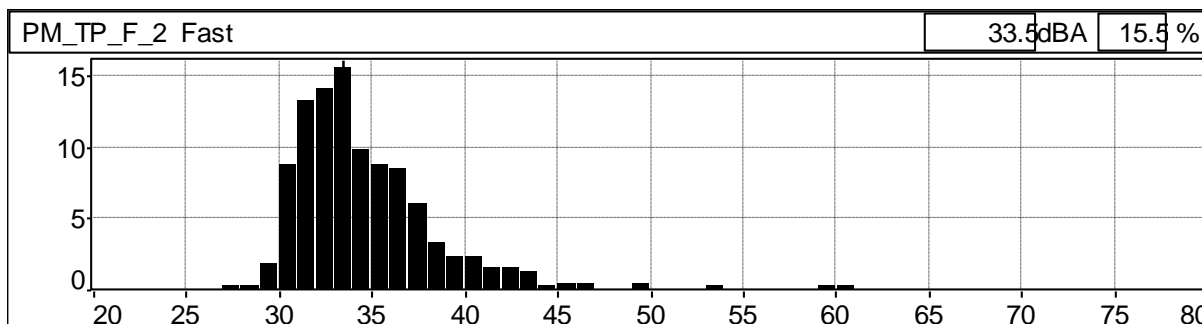
Grafico 136: Distribuzione cumulativa ponderata in curva "A" e costante di tempo "FAST"
