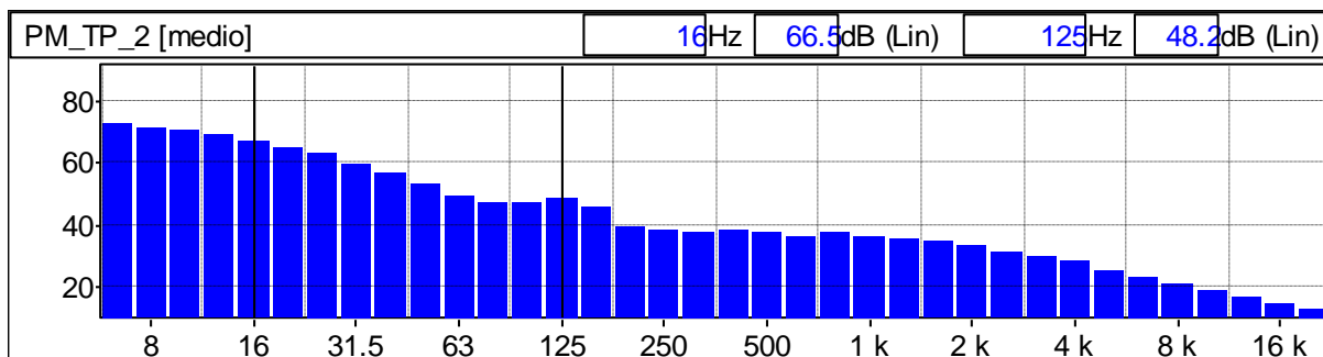
Grafico 22: Spettro del rumore rilevato 1/3 Ottava Leq Lineare
