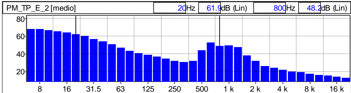
Grafico 126: Spettro del rumore rilevato 1/3 Ottava Leq Lineare
