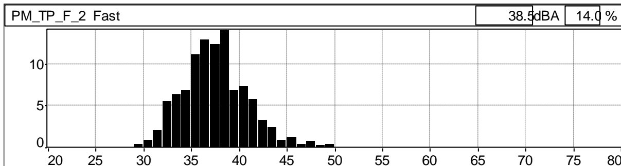
Grafico 140: Distribuzione cumulativa ponderata in curva "A" e costante di tempo "FAST"
