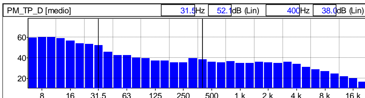
Grafico 106: Spettro del rumore rilevato 1/3 Ottava Leq Lineare
