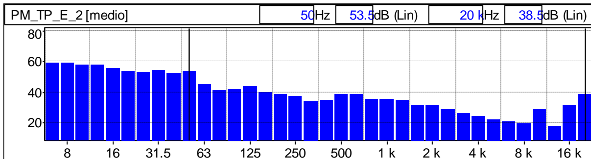
Grafico 118: Spettro del rumore rilevato 1/3 Ottava Leq Lineare
