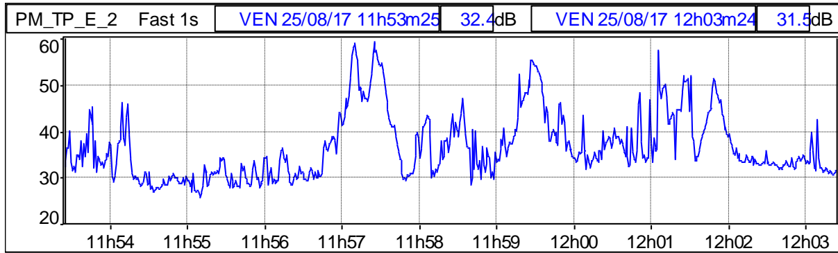
Grafico 117: Profilo temporale ponderato in curva "A" e costante di tempo "FAST"
