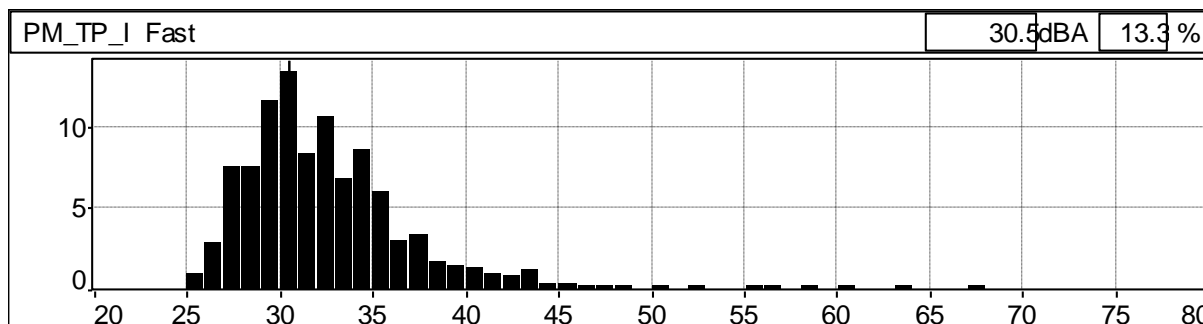
Grafico 176: Distribuzione cumulativa ponderata in curva "A" e costante di tempo "FAST"
