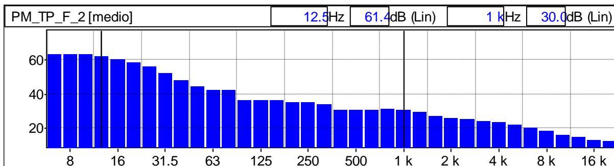
Grafico 134: Spettro del rumore rilevato 1/3 Ottava Leq Lineare
