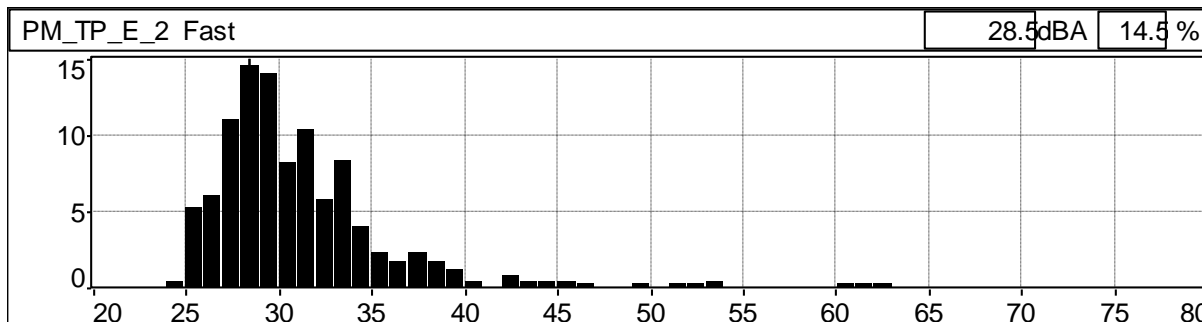
Grafico 124: Distribuzione cumulativa ponderata in curva "A" e costante di tempo "FAST"
