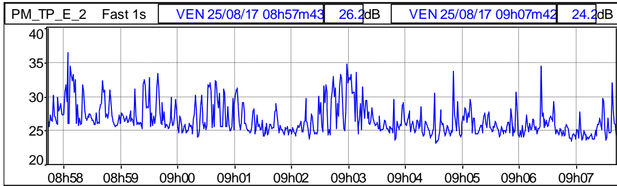
Grafico 113: Profilo temporale ponderato in curva "A" e costante di tempo "FAST"
