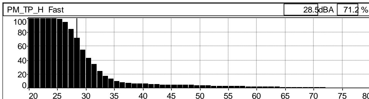
Grafico 156: Distribuzione cumulativa ponderata in curva "A" e costante di tempo "FAST"
