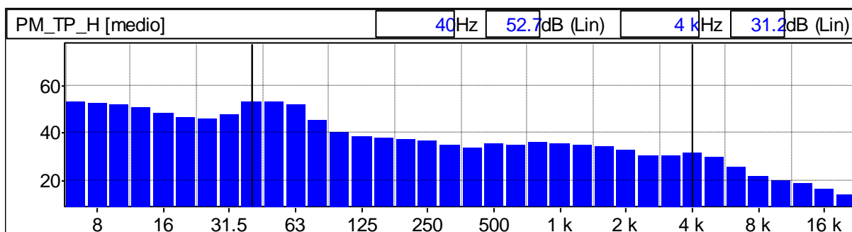
Grafico 158: Spettro del rumore rilevato 1/3 Ottava Leq Lineare
