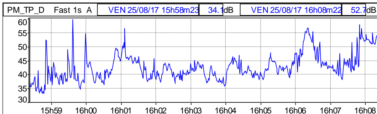
Grafico 105: Profilo temporale ponderato in curva "A" e costante di tempo "FAST"
