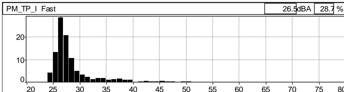
Grafico 168: Distribuzione cumulativa ponderata in curva "A" e costante di tempo "FAST"
