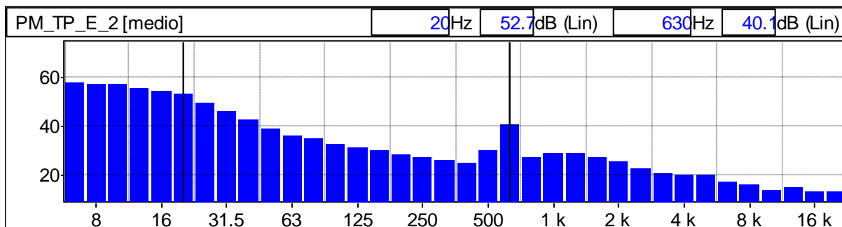
Grafico 122: Spettro del rumore rilevato 1/3 Ottava Leq Lineare
