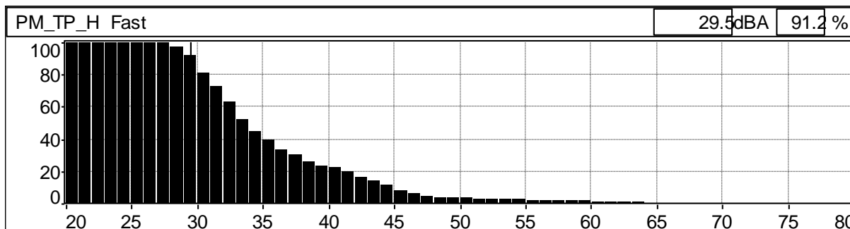
Grafico 160: Distribuzione cumulativa ponderata in curva "A" e costante di tempo "FAST"
