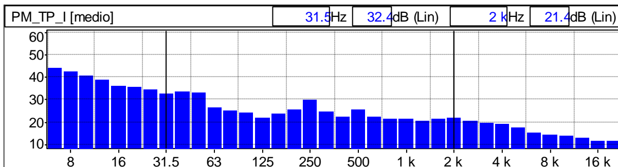
Grafico 166: Spettro del rumore rilevato 1/3 Ottava Leq Lineare
