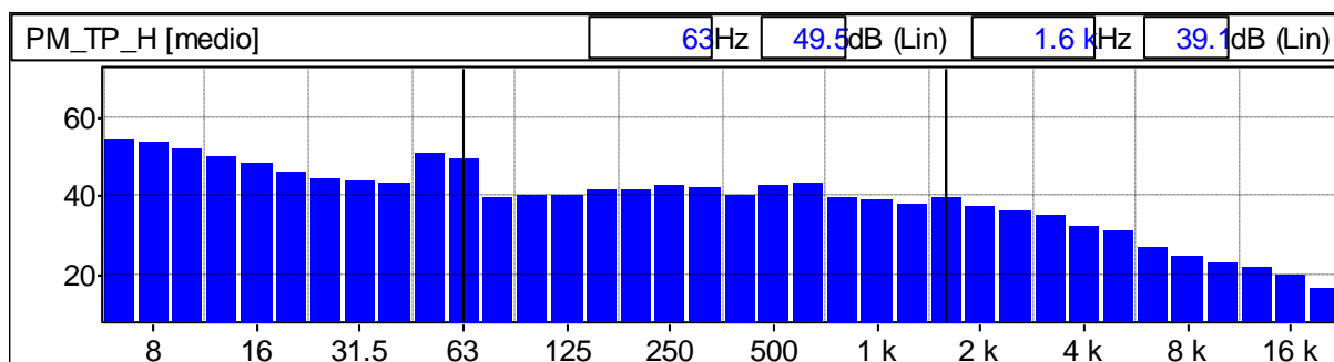
Grafico 154: Spettro del rumore rilevato 1/3 Ottava Leq Lineare
