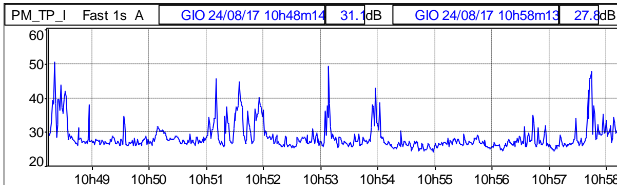
Grafico 165: Profilo temporale ponderato in curva "A" e costante di tempo "FAST"
