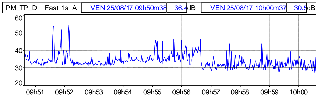
Grafico 97: Profilo temporale ponderato in curva "A" e costante di tempo "FAST"
