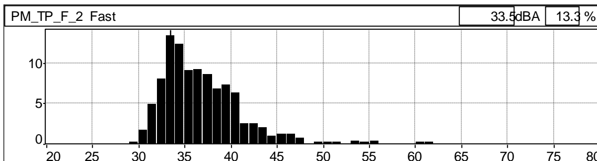
Grafico 144: Distribuzione cumulativa ponderata in curva "A" e costante di tempo "FAST"
