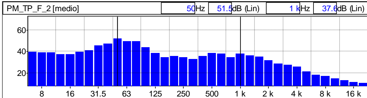
Grafico 130: Spettro del rumore rilevato 1/3 Ottava Leq Lineare
