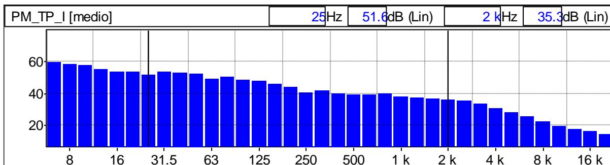
Grafico 170: Spettro del rumore rilevato 1/3 Ottava Leq Lineare
