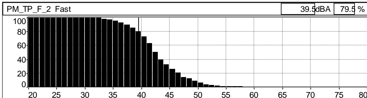
Grafico 132: Distribuzione cumulativa ponderata in curva "A" e costante di tempo "FAST"
