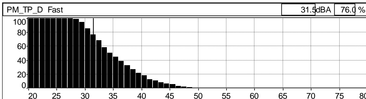
Grafico 112: Distribuzione cumulativa ponderata in curva "A" e costante di tempo "FAST"
