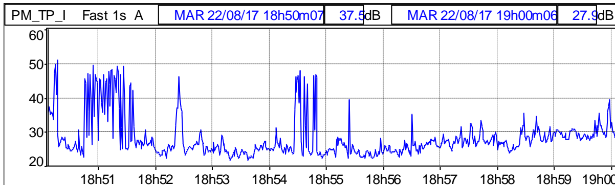
Grafico 161: Profilo temporale ponderato in curva "A" e costante di tempo "FAST"
