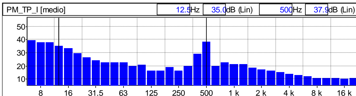
Grafico 162: Spettro del rumore rilevato 1/3 Ottava Leq Lineare
