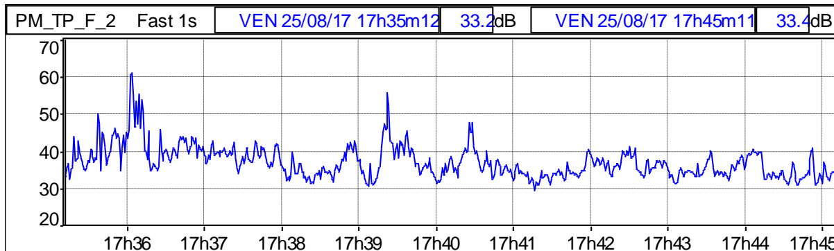
Grafico 141: Profilo temporale ponderato in curva "A" e costante di tempo "FAST"
