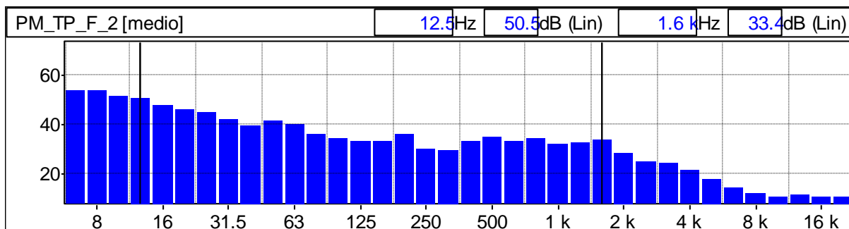
Grafico 142: Spettro del rumore rilevato 1/3 Ottava Leq Lineare
