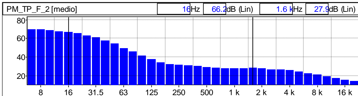
Grafico 138: Spettro del rumore rilevato 1/3 Ottava Leq Lineare
