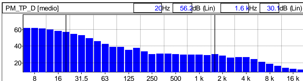
Grafico 102: Spettro del rumore rilevato 1/3 Ottava Leq Lineare
