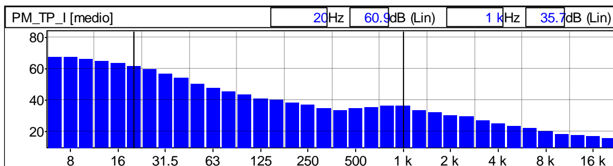
Grafico 174: Spettro del rumore rilevato 1/3 Ottava Leq Lineare
