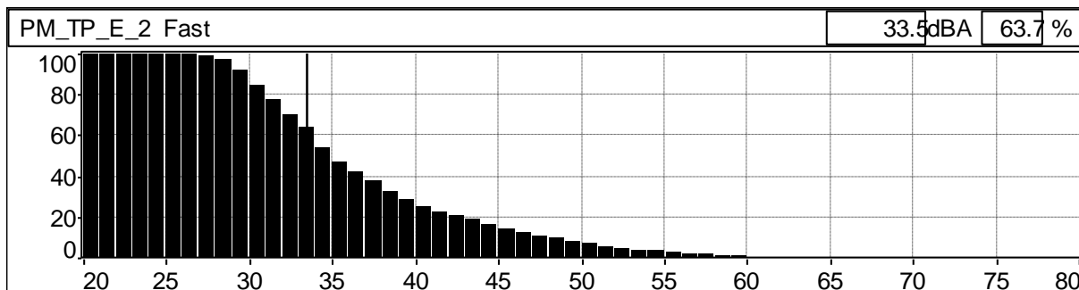
Grafico 120: Distribuzione cumulativa ponderata in curva "A" e costante di tempo "FAST"
