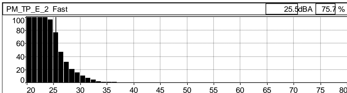
Grafico 116: Distribuzione cumulativa ponderata in curva "A" e costante di tempo "FAST"
