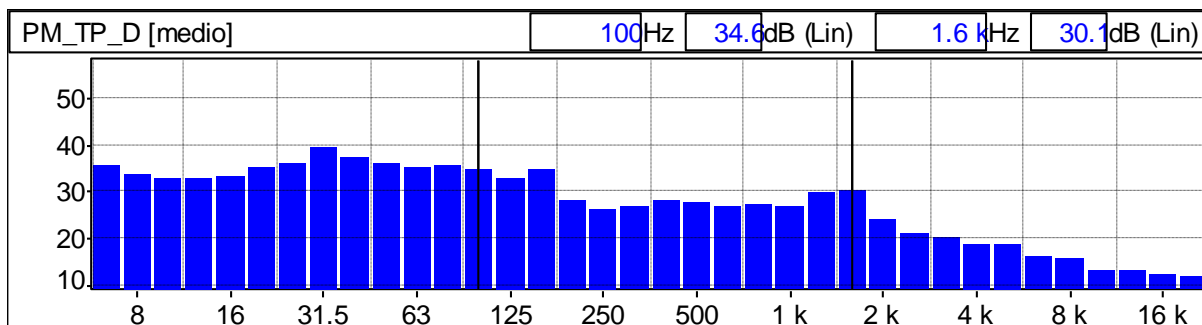
Grafico 98: Spettro del rumore rilevato 1/3 Ottava Leq Lineare
