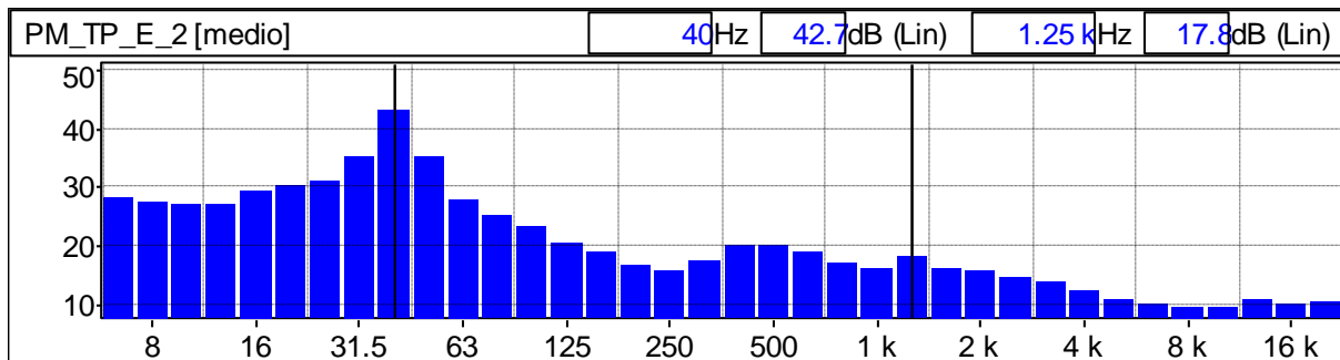
Grafico 114: Spettro del rumore rilevato 1/3 Ottava Leq Lineare
