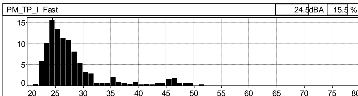
Grafico 164: Distribuzione cumulativa ponderata in curva "A" e costante di tempo "FAST"
