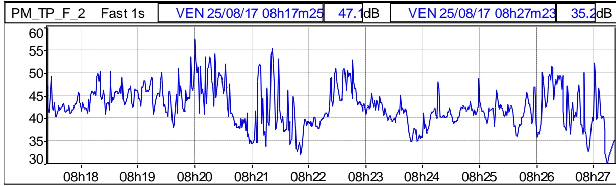
Grafico 129: Profilo temporale ponderato in curva "A" e costante di tempo "FAST"
