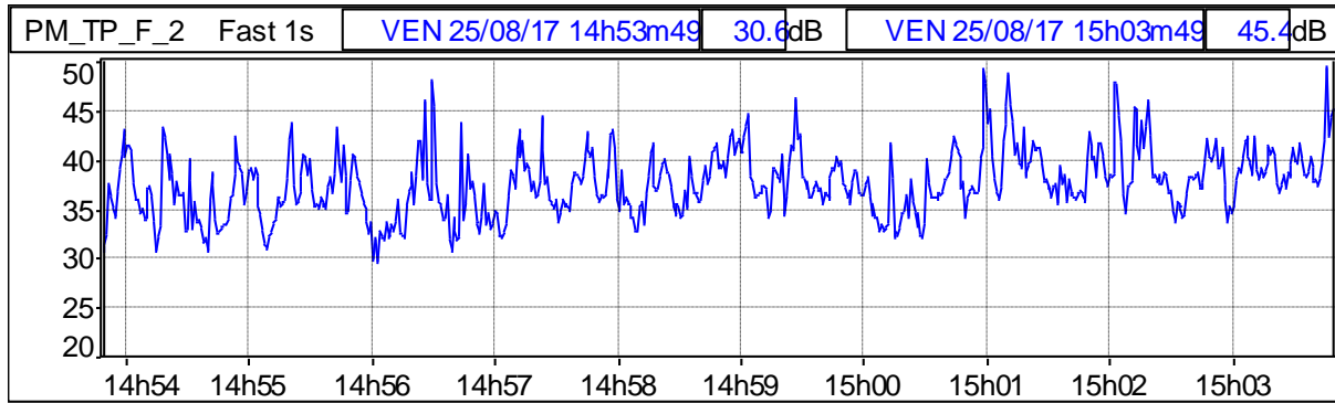
Grafico 137: Profilo temporale ponderato in curva "A" e costante di tempo "FAST"
