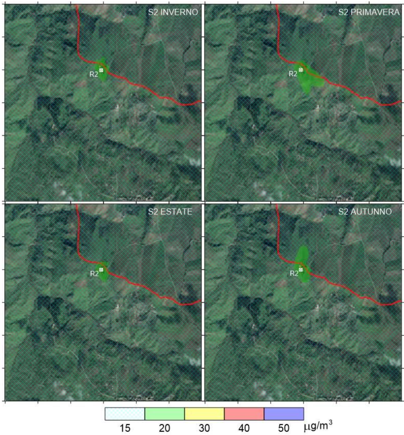
Figura All-2: Massimo stagionale delle concentrazioni giornaliere di PM 10 per la sorgente S2
