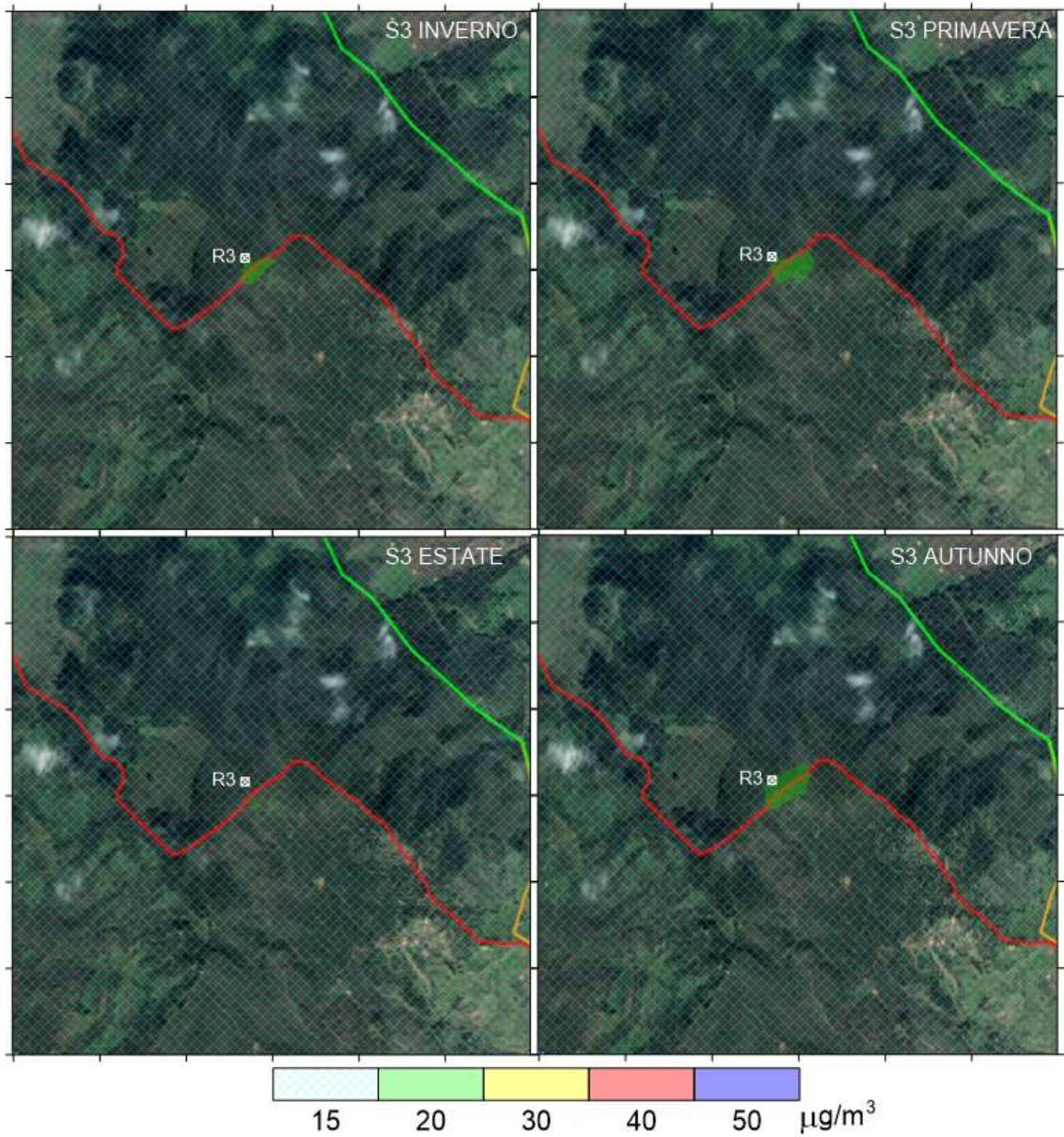
Figura All-3: Massimo stagionale delle concentrazioni giornaliere di PM 10 per la sorgente S3
