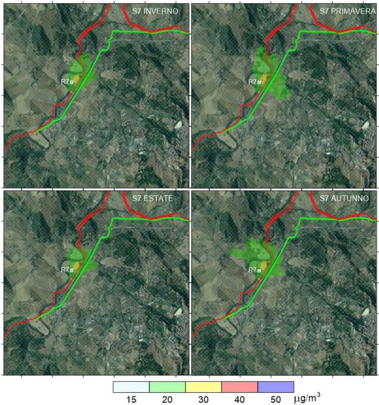
Figura All-7: Massimo stagionale delle concentrazioni giornaliere di PM 10 per la sorgente S7
