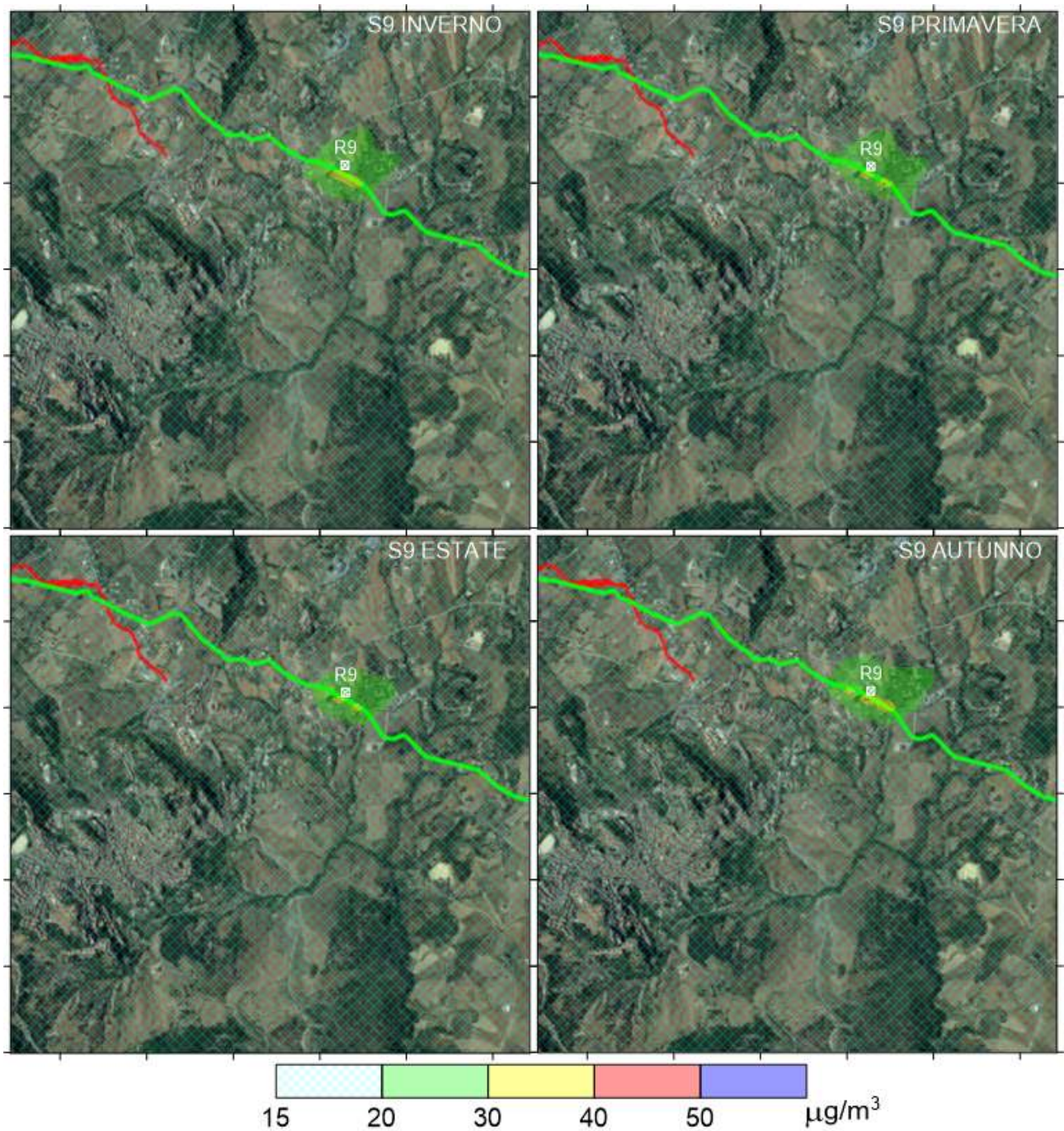
Figura All-9: Massimo stagionale delle concentrazioni giornaliere di PM 10 per la sorgente S9
