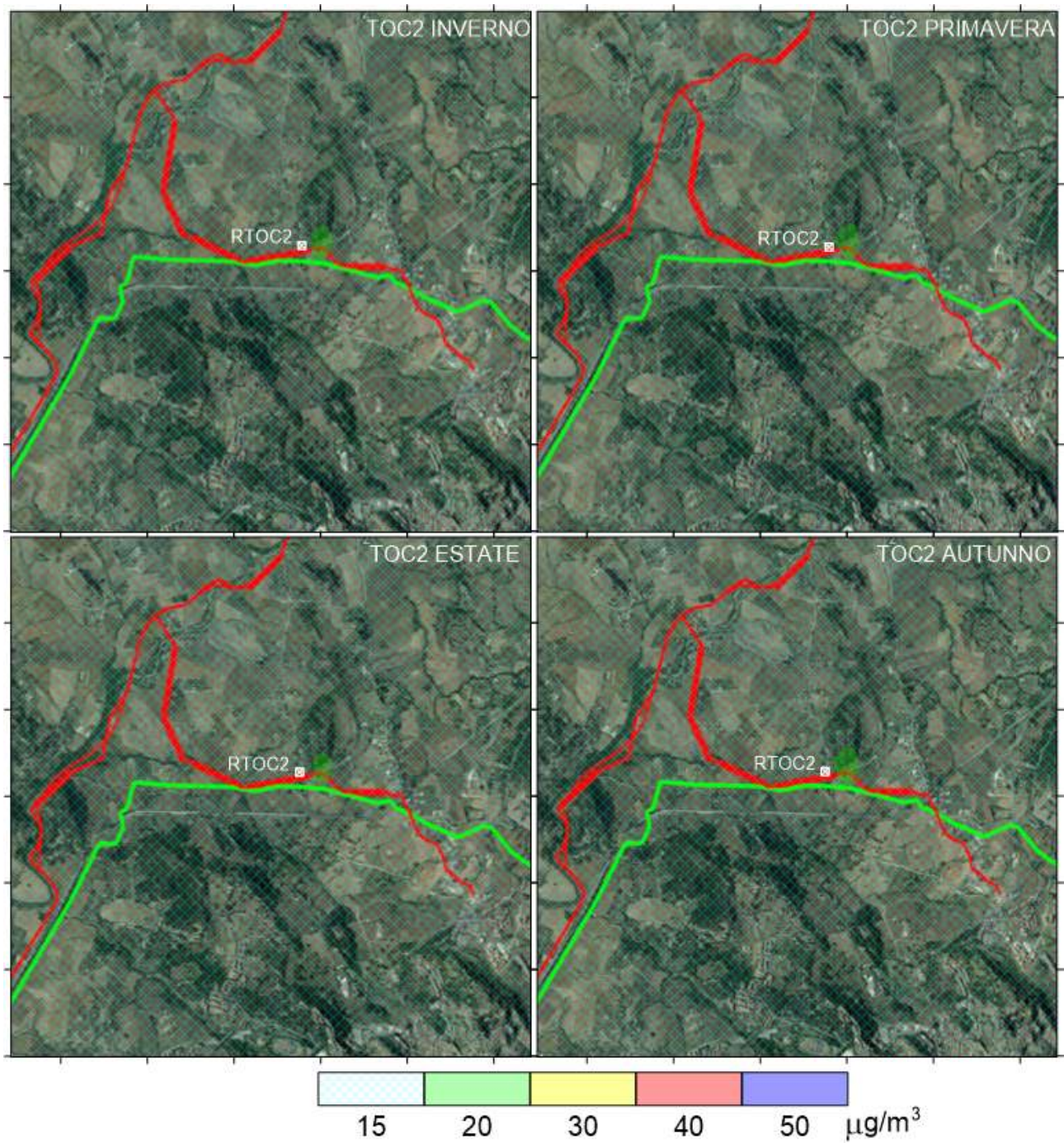
Figura All-TOC2: Massimo stagionale delle concentrazioni giornaliere di PM 10 per la sorgente STOC2
