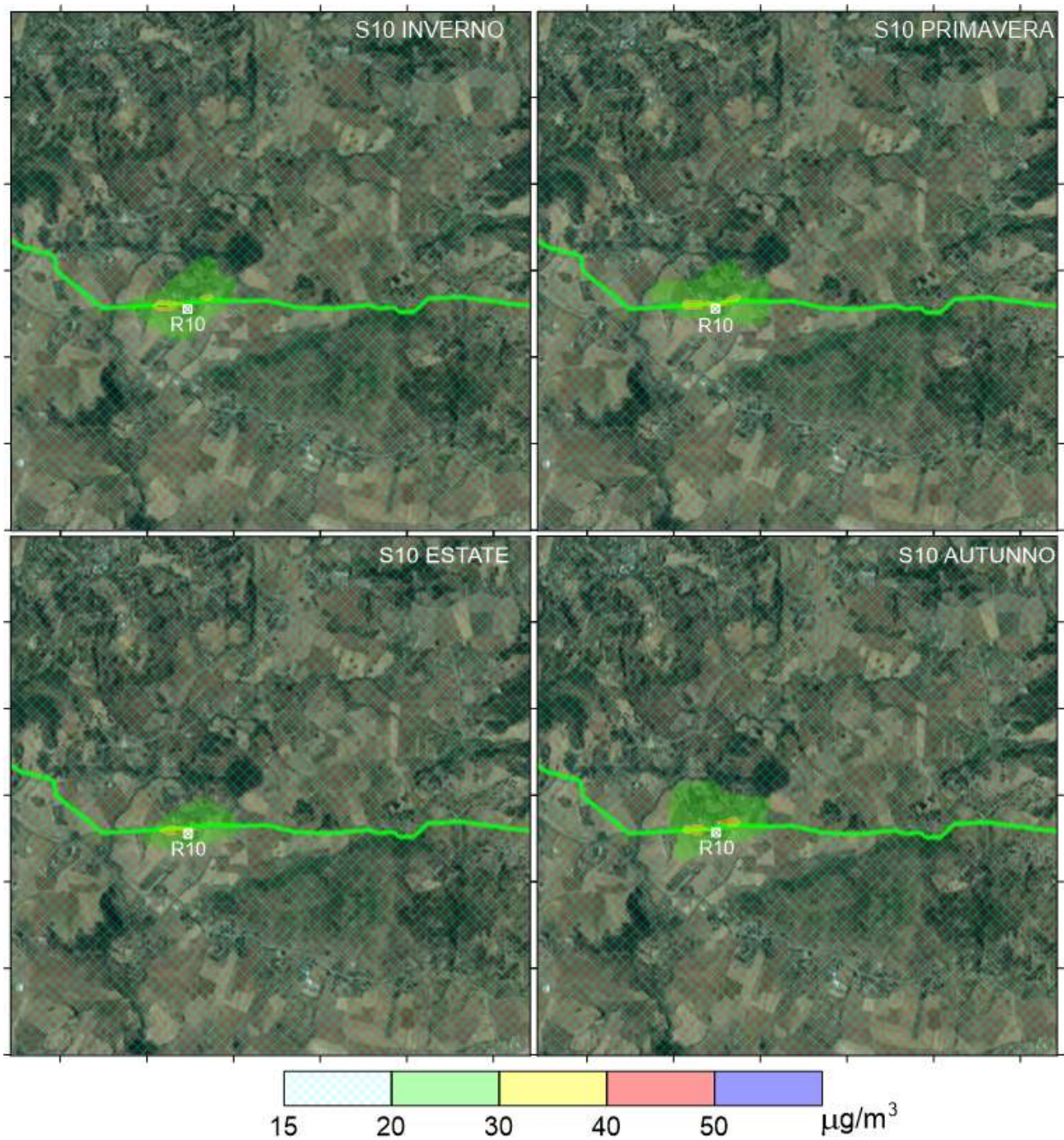
Figura All-10: Massimo stagionale delle concentrazioni giornaliere di PM 10 per la sorgente S10
