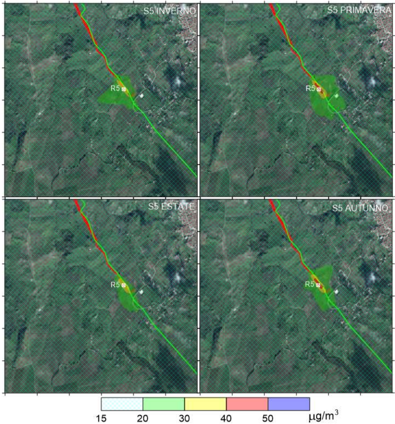
Figura All-5: Massimo stagionale delle concentrazioni giornaliere di PM 10 per la sorgente S5
