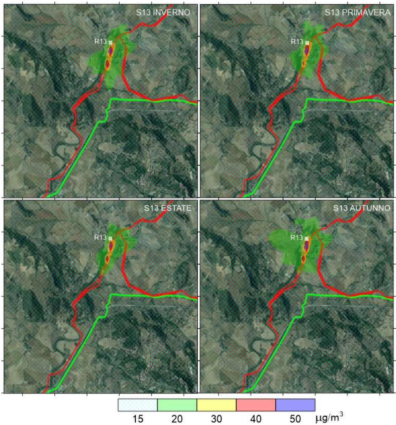
Figura All-13: Massimo stagionale delle concentrazioni giornaliere di PM 10 per la sorgente S13
