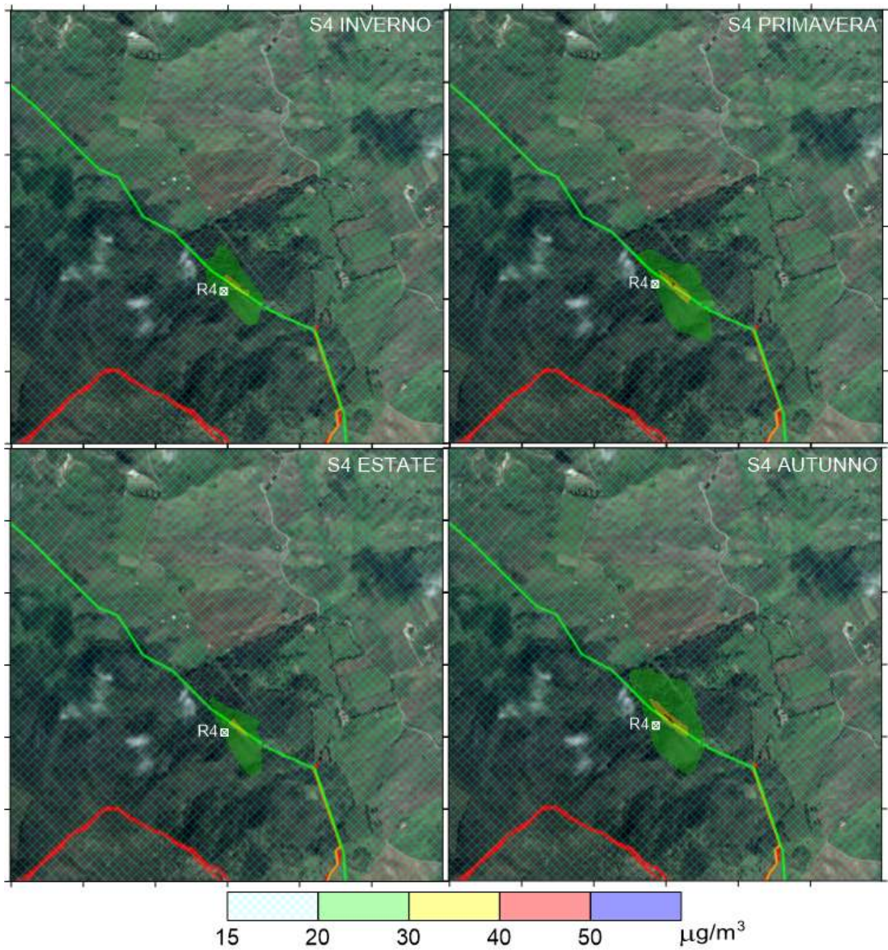
Figura All-4: Massimo stagionale delle concentrazioni giornaliere di PM 10 per la sorgente S4
