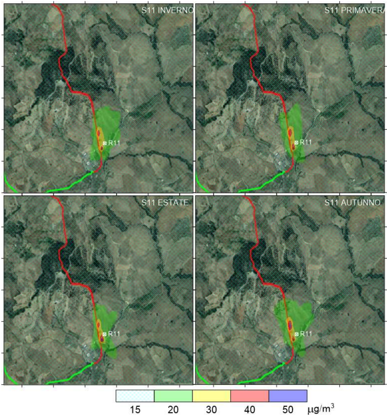
Figura All-11: Massimo stagionale delle concentrazioni giornaliere di PM 10 per la sorgente S11
