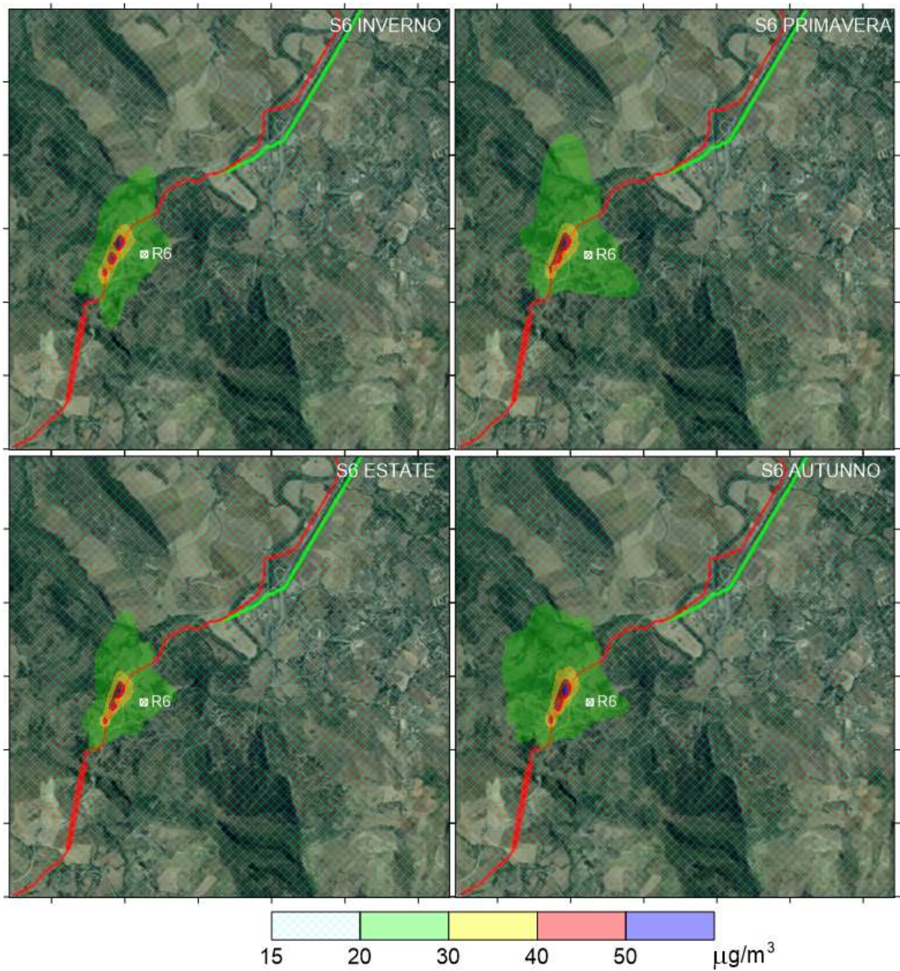
Figura All-6 Massimo stagionale delle concentrazioni giornaliere di PM 10 per la sorgente S6
