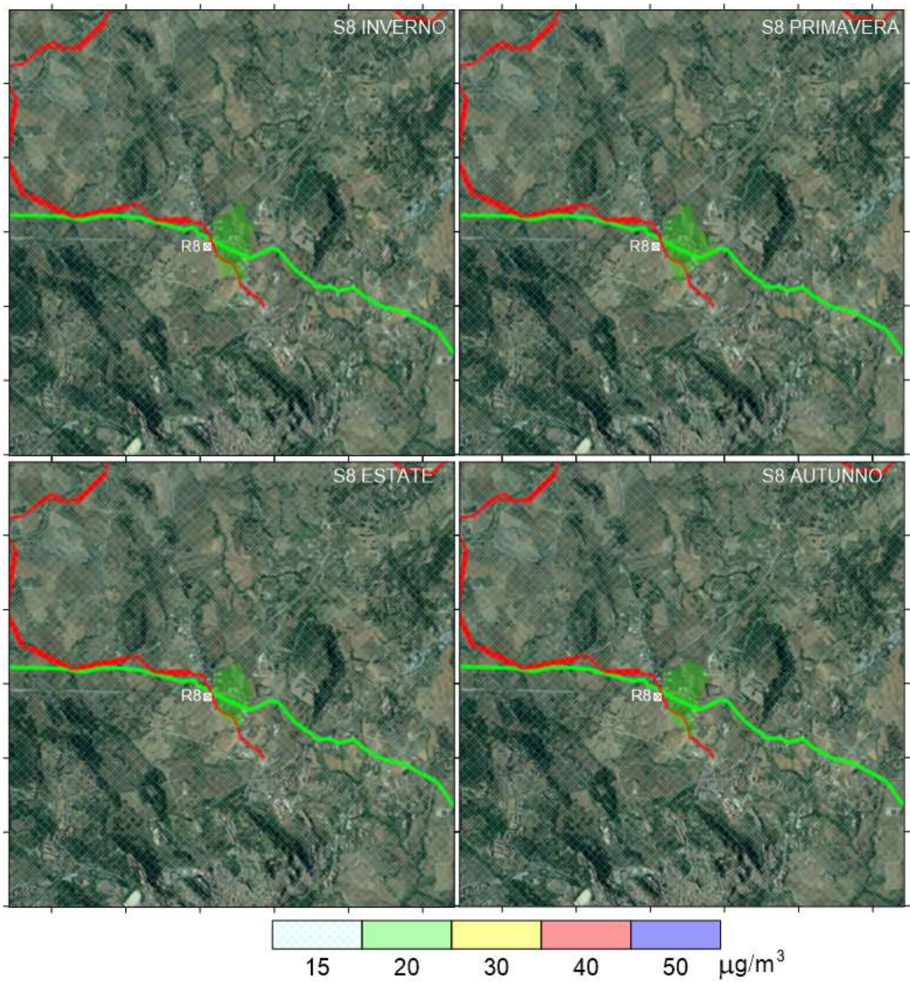
Figura All-8: Massimo stagionale delle concentrazioni giornaliere di PM 10 per la sorgente S8
