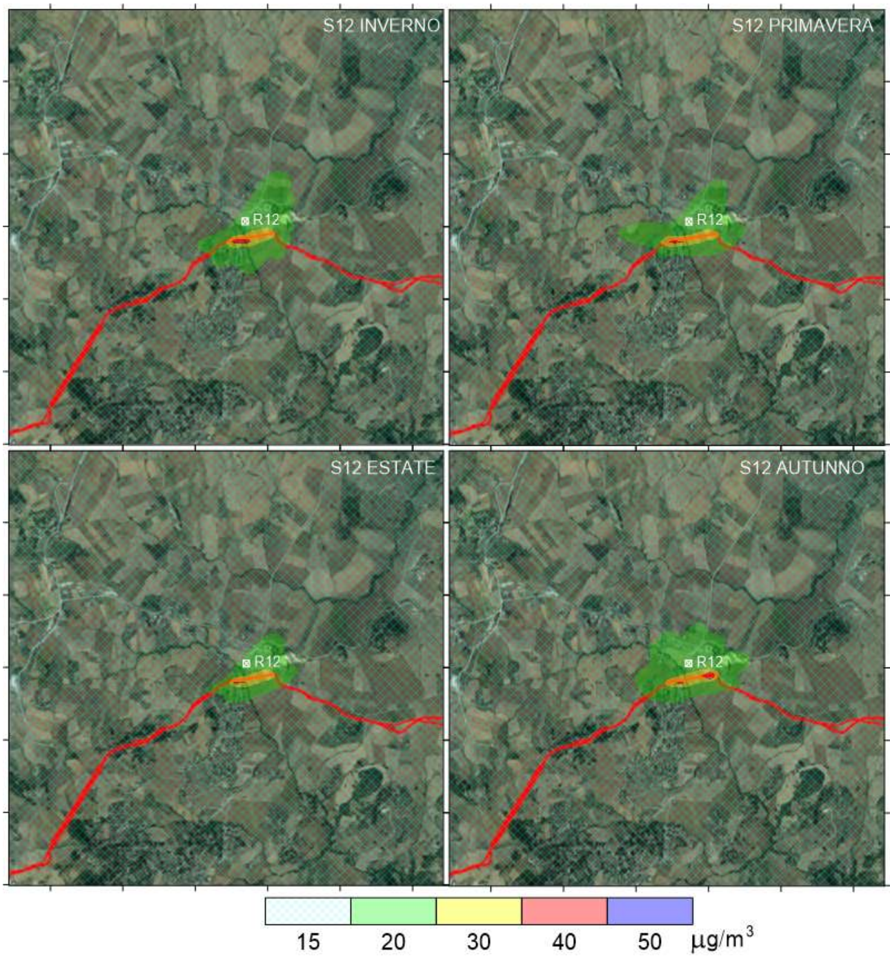
Figura All-12: Massimo stagionale delle concentrazioni giornaliere di PM 10 per la sorgente S12
