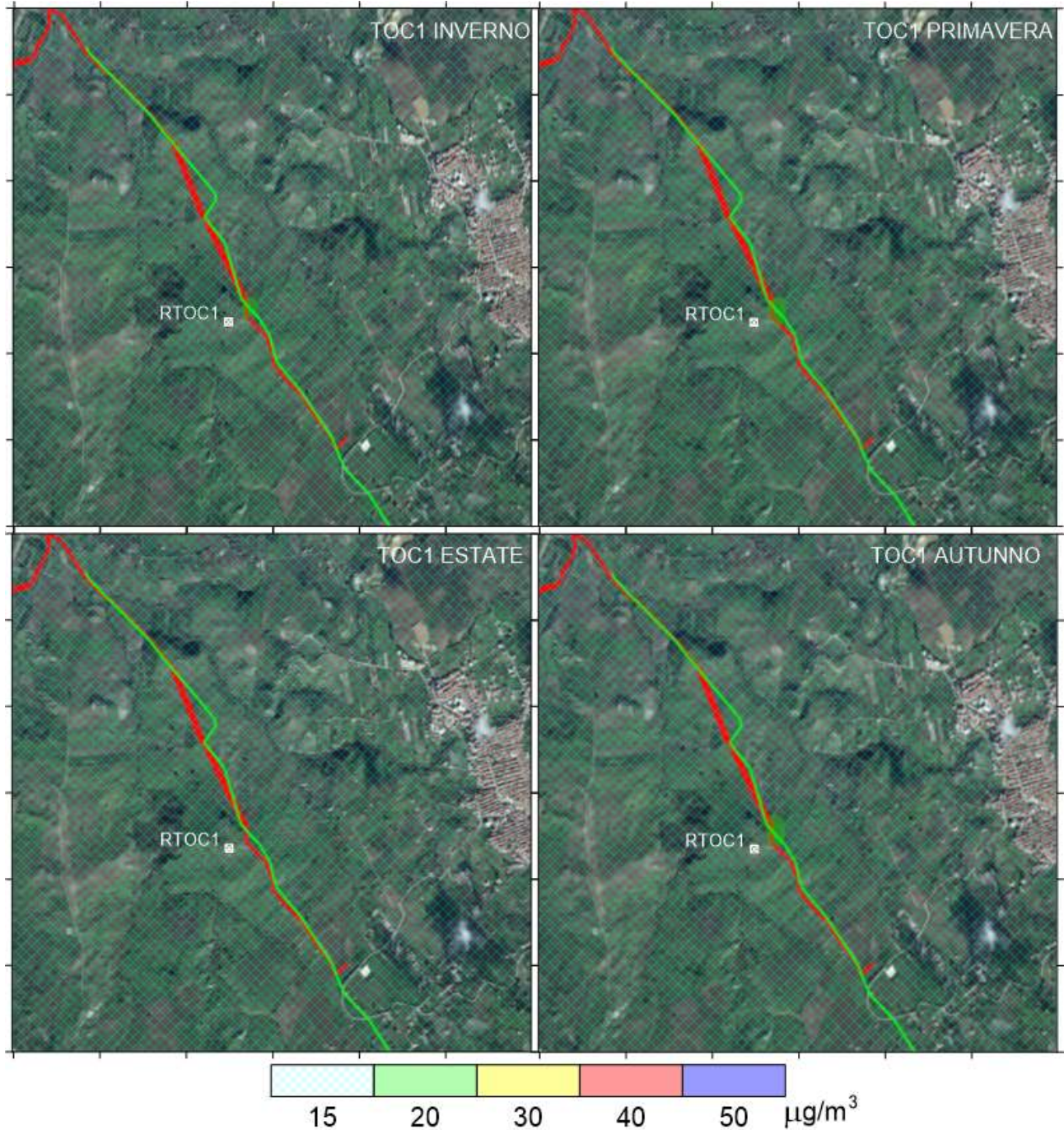
Figura All-TOC1: Massimo stagionale delle concentrazioni giornaliere di PM 10 per la sorgente STOC1
