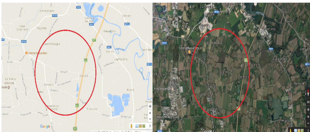
Figura 1 Inquadramento topografico e geomorfologico dell'area in esame (da google maps).
