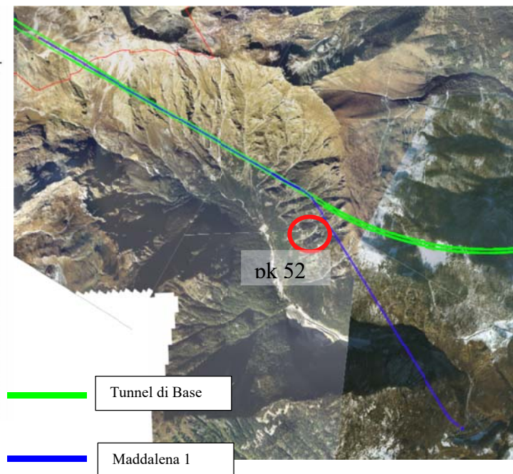
tracciato galleria maddalena su foto aerea
