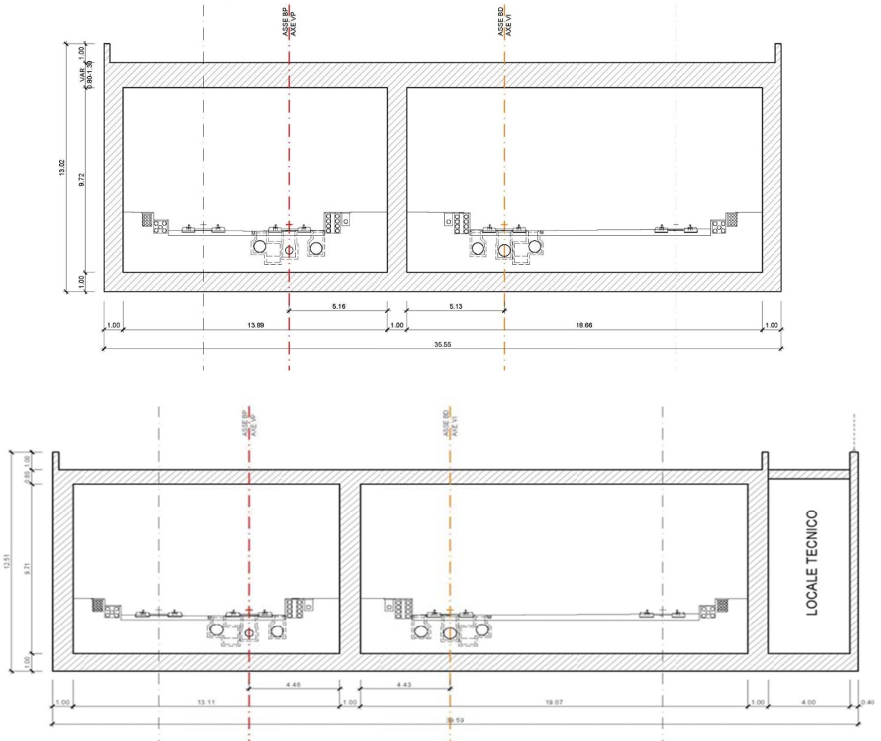
Sezione Tipo Galleria Artificiale Da Pk 61+105 A Pk 61+182 Binario Pari
